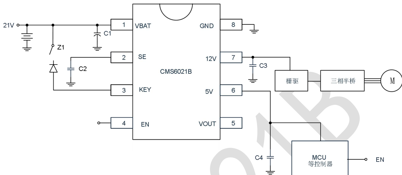
图 7-1 典型应用电路图
