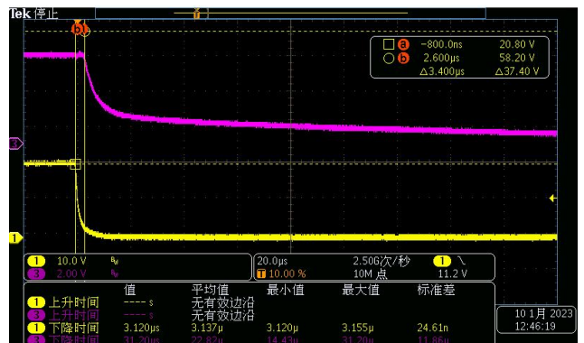
VBAT=VKEY=21V, 5V 带载 30mA 图 9-30 VBAT 下电 5V 输出
