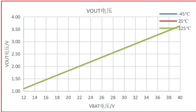
图 9-13 分压输出 V_{OUT} vs V_{BAT}
