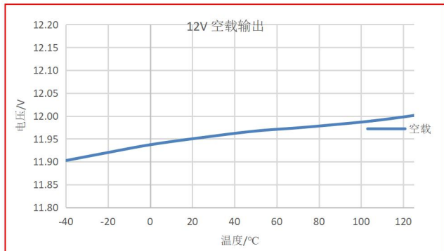
图 9-1 12V 空载输出 vs 温度
