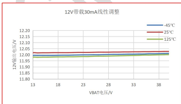
图 9-5 12V 带载 30mA 输出 vs VBAT
