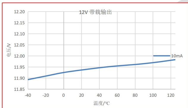
图 9-3 12V 带载输出 vs 温度
