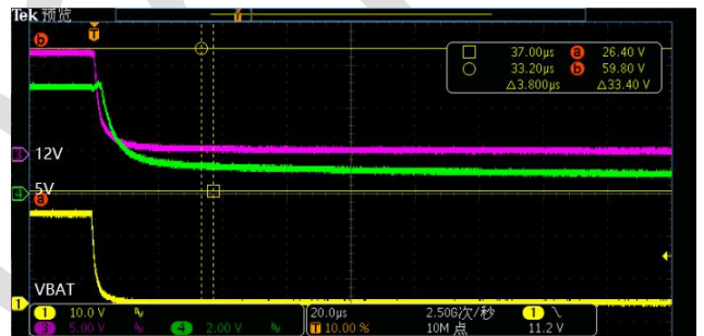
VBAT=VKEY=21V, 12V 带载 60mA 图 9-28 VBAT 下电 12V 输出
