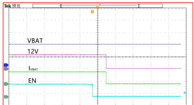
图 9-18 EN 关断零待机电流
