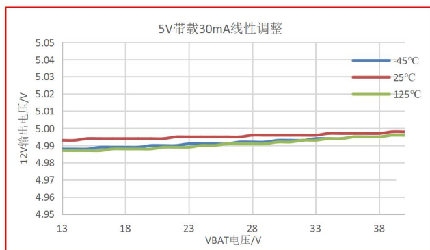
图 9-6 5V 带载 30mA 输出 vs VBAT
