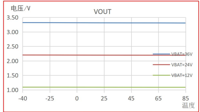
图 9-14 V_{OUT} vs 温度
