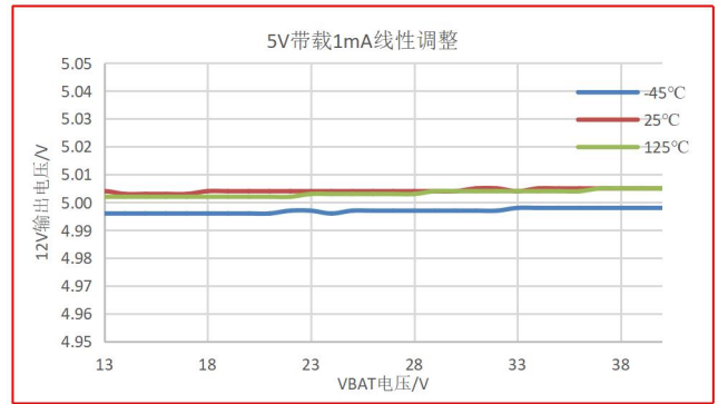
图 9-8 5V 线性调整 vs VBAT
