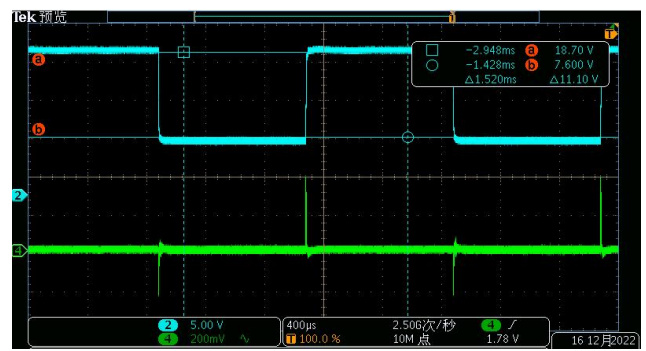
\Delta V_{BAT}=10V, I_{5V}=30mA, SR_{BAT}=1.8V/us 图 9-24 5V 电源响应
