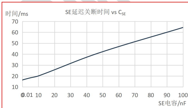
图 9-17 SE 延迟关断时间 vs C_{SE}
