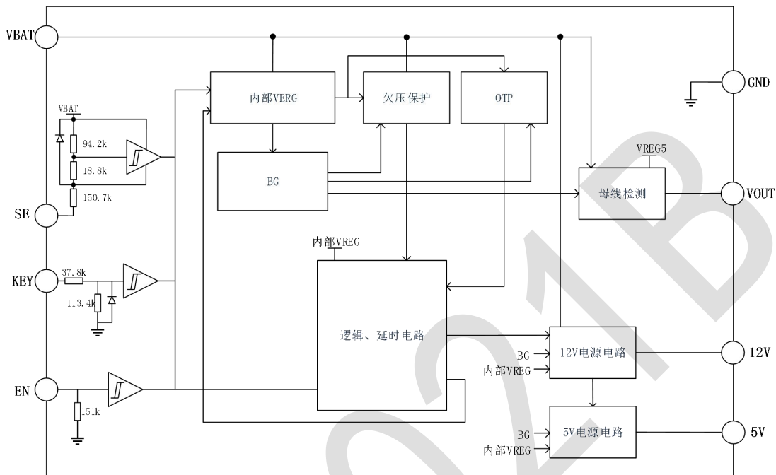
图 3-1 CMS6021B 内部框图
