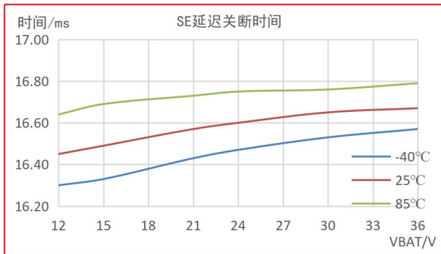
图 9-15 SE 延迟关断时间 vs V_{BAT}
