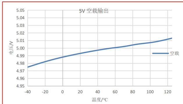
图 9-2 5V 空载输出 vs 温度
