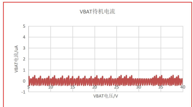
图 9-12 VBAT 待机电流 vs VBAT
