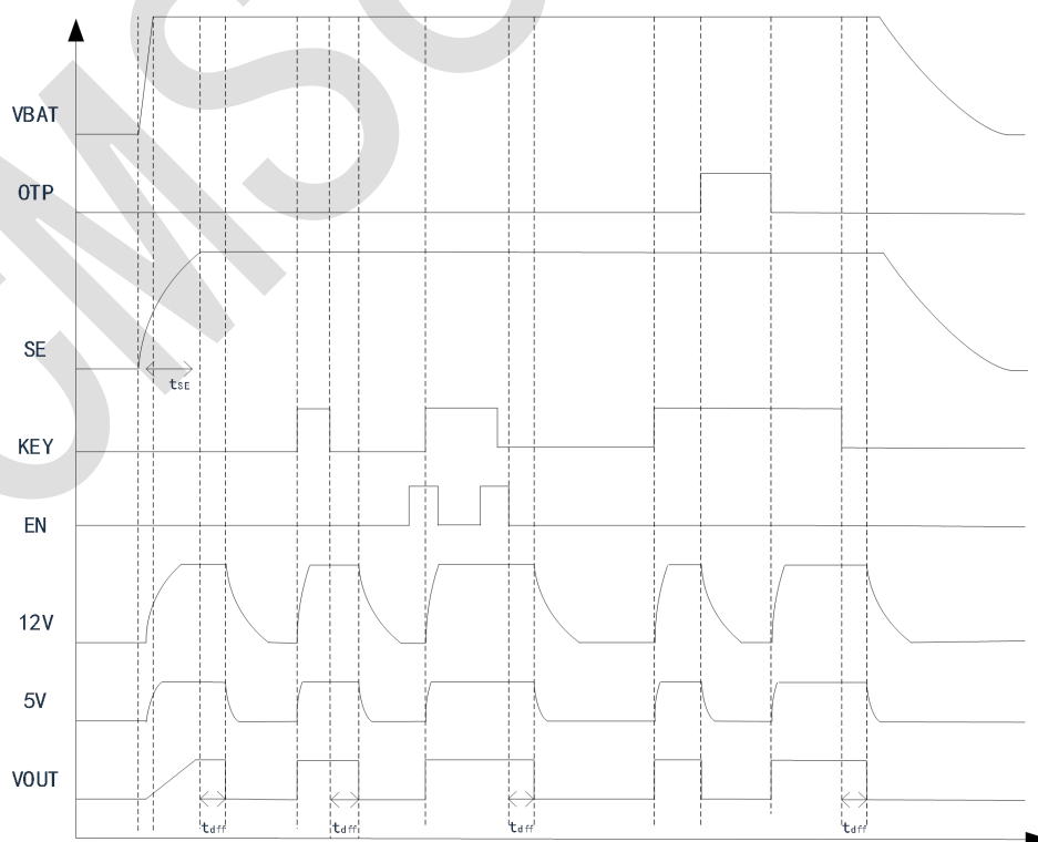
图 3-2 逻辑时序图
