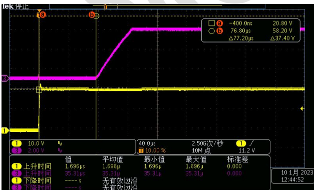
VBAT=VKEY=21V, 5V 带载 30mA 图 9-29 VBAT 上电 5V 输出
