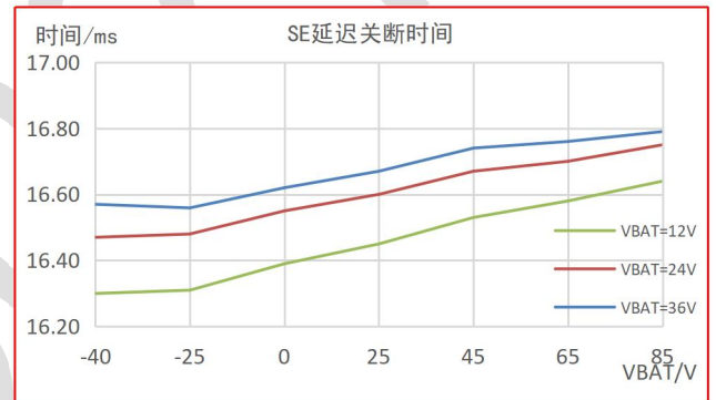
图 9-16 SE 延迟关断时间 vs 温度
