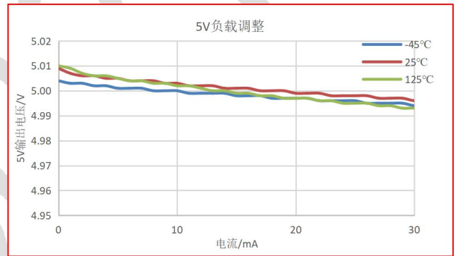
图 9-10 5V 负载调整
