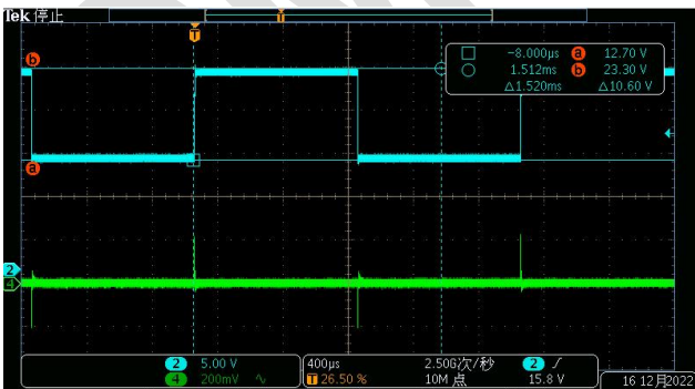
\Delta V_{BAT}=10V, I_{12V}=30mA, SR_{BAT}=1.8V/us 图 9-23 12V 电源响应
