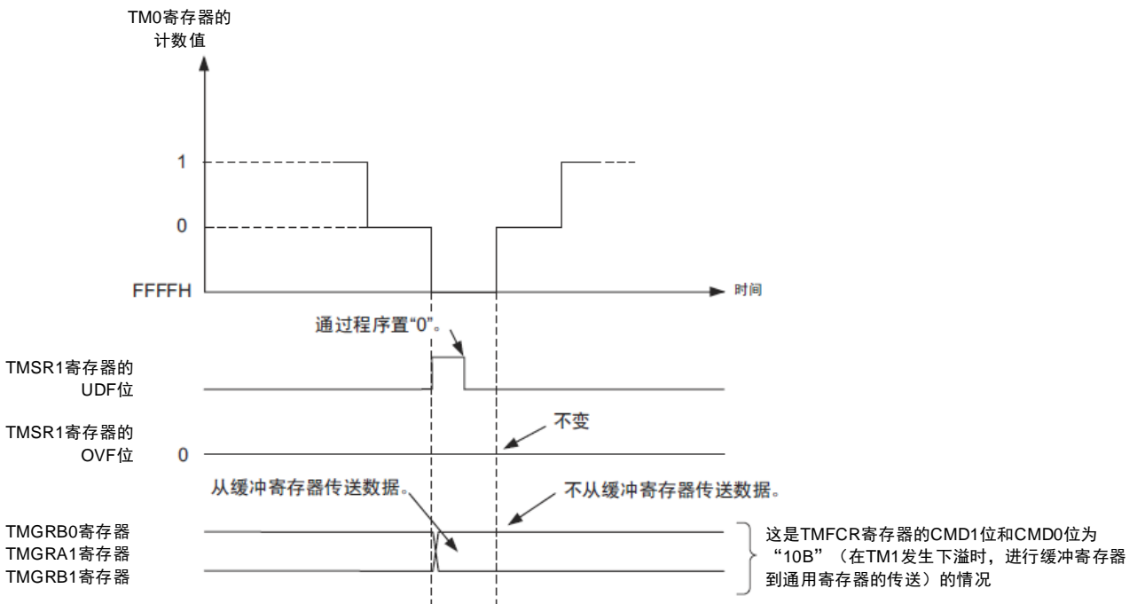
图10-65 互补PWM模式中的TM1发生下溢时的运行例子
