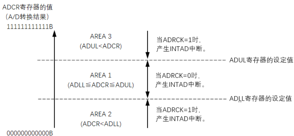
图15-8 ADRCK位的中断信号产生范围
