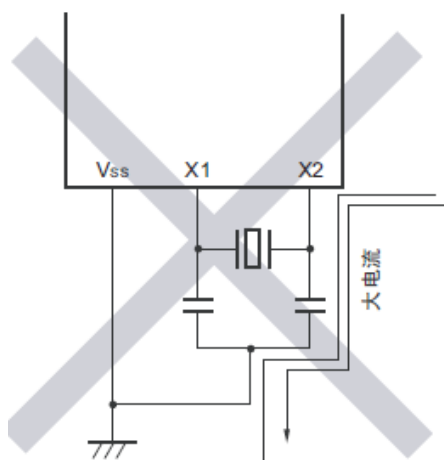
(e) 有变化的大电流接近信号线
