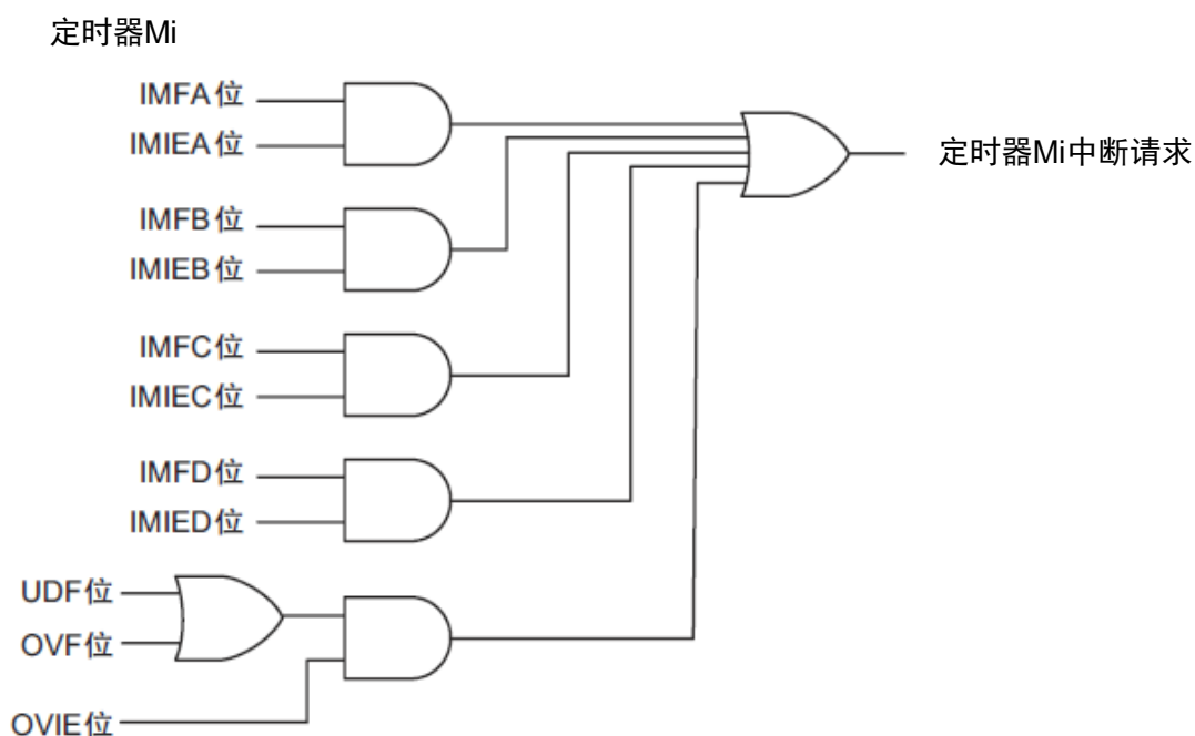
图10-63 定时器M中断的框图
