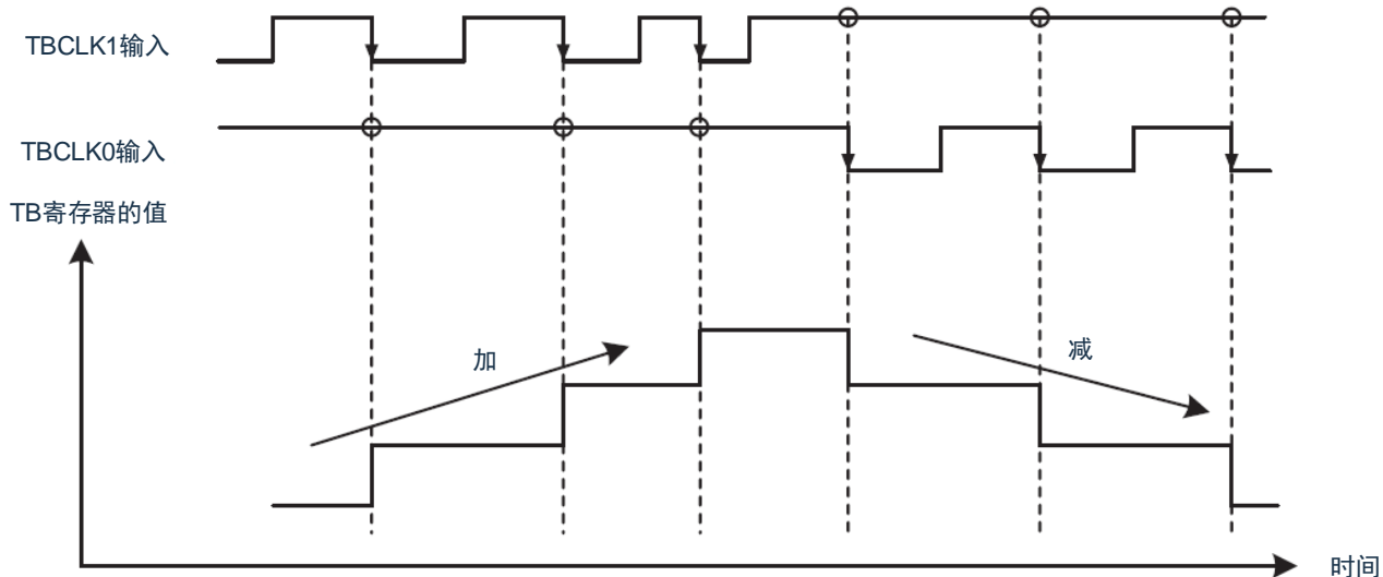
图8-30 相位计数模式的运行例子4
