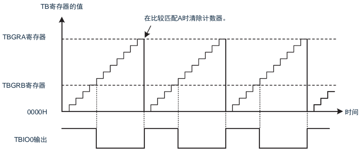
图8-24 PWM模式的运行例子(1)
