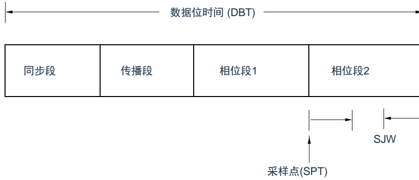
图21-19. 参考: 由 CAN 规范定义的数据位时间配置
