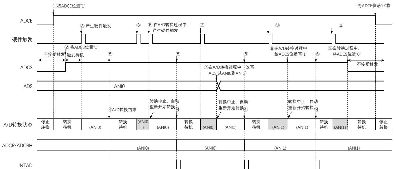
图15-22 硬件触发无等待模式(选择模式、单次转换模式)的运行时序例子
