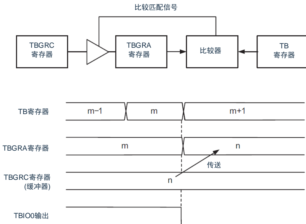
图8-14 输出比较功能的缓冲器运行
