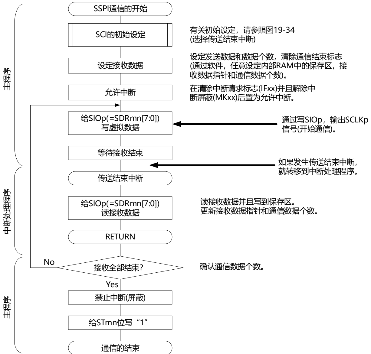
图19-38 主控接收(单次接收模式)的流程图
