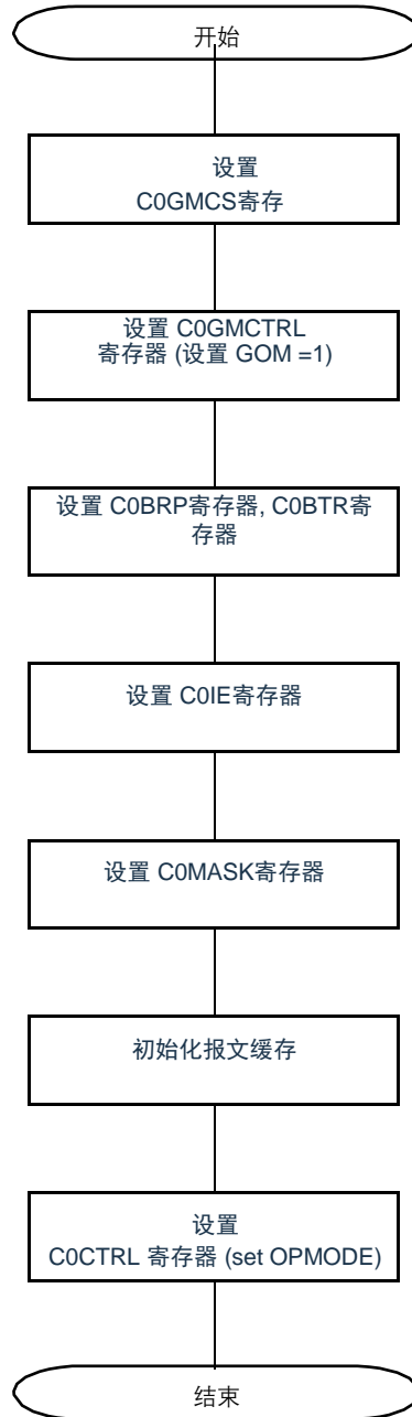
图21-63.初始化
