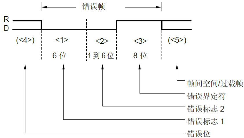
图21-15. 错误帧
