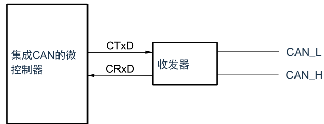
图21-22. 连接到CAN总线
