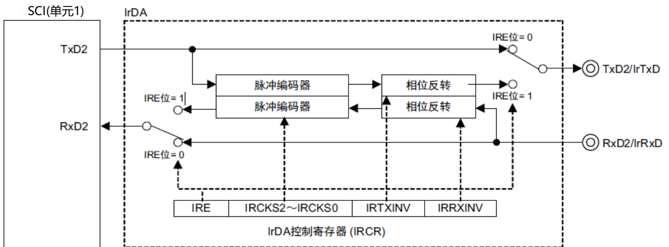
图22-1 IrDA与SCI的合作示意框图
