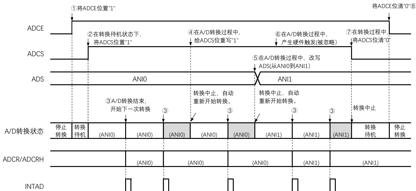
图15-17 软件触发模式(选择模式、连续转换模式)的运行时序例子
