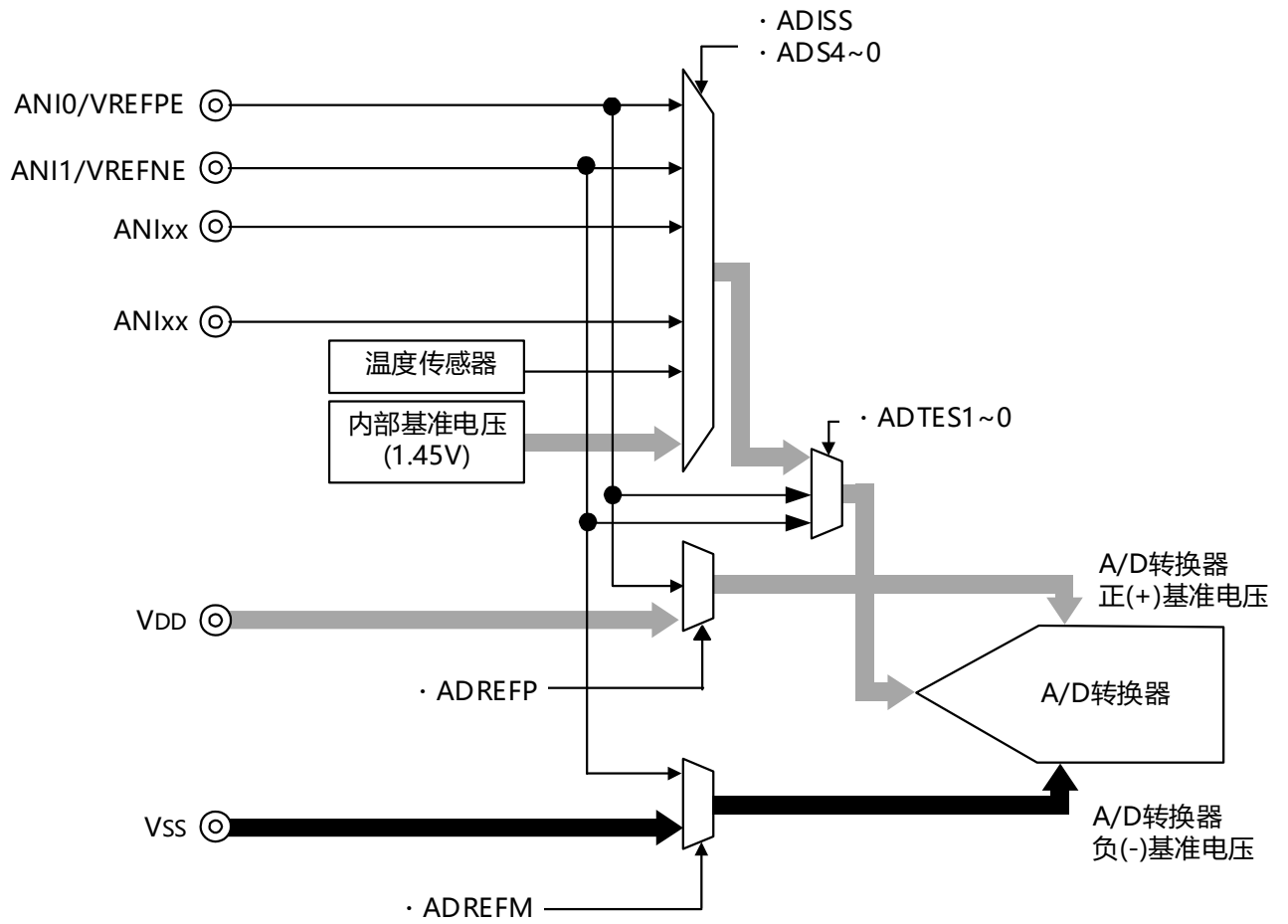
图31-11 A/D测试功能的结构
