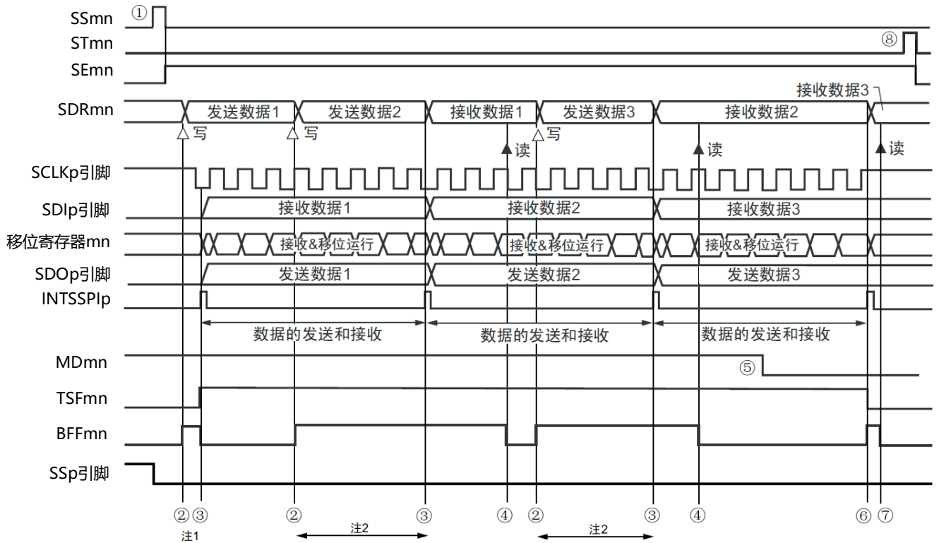
图19-98 从属发送和接收(连续发送和接收模式)的时序图(类型1: DAPmn=0、CKPmn=0)
