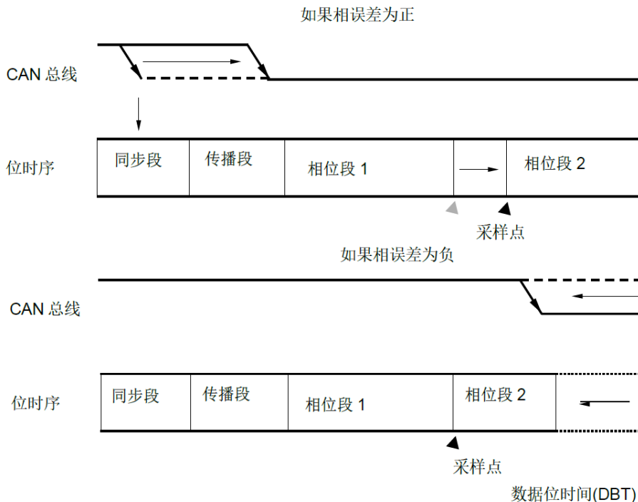
图21-21.重同步
