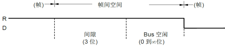
图21-13. 帧间空间(错误活动节点)
