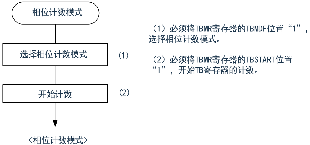
图8-26 相位计数模式的设置步骤例子
