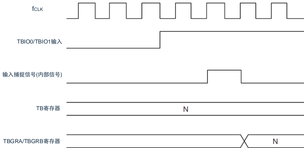
图8-17 输入捕捉的输入信号时序
