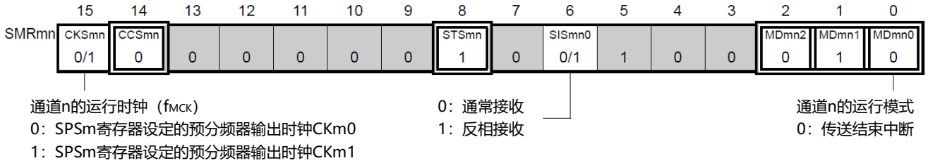
图19-109 UART(UART0~UART2)的UART接收时的寄存器设置内容例子(1/2)
