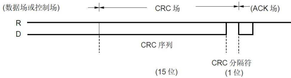
图21-10. CRC场
