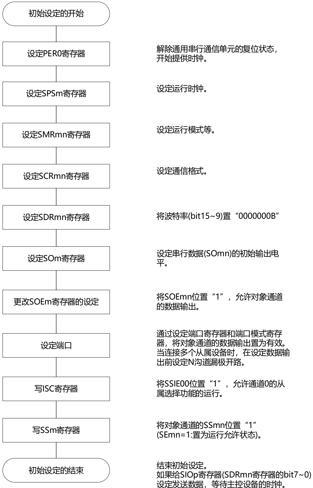
图19-93 从属发送和接收的初始设置步骤
