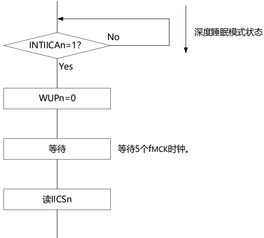
图20-23 通过地址匹配将WUPn位置“0”时的流程(包括接收扩展码)
