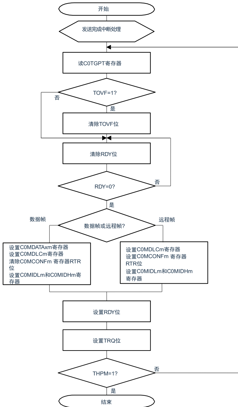
图21-71. 通过中断发送(使用C0TGPT寄存器)
