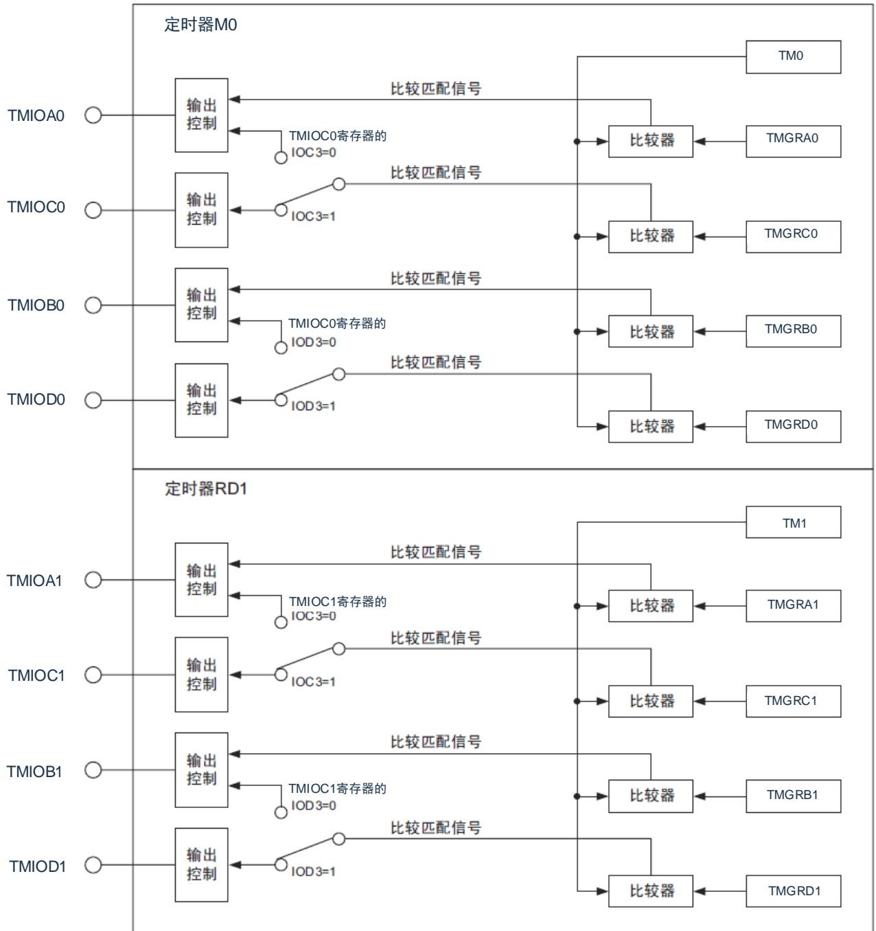
图 10-51 TMGR C i 和 TMGRD i 的输出引脚的变更
