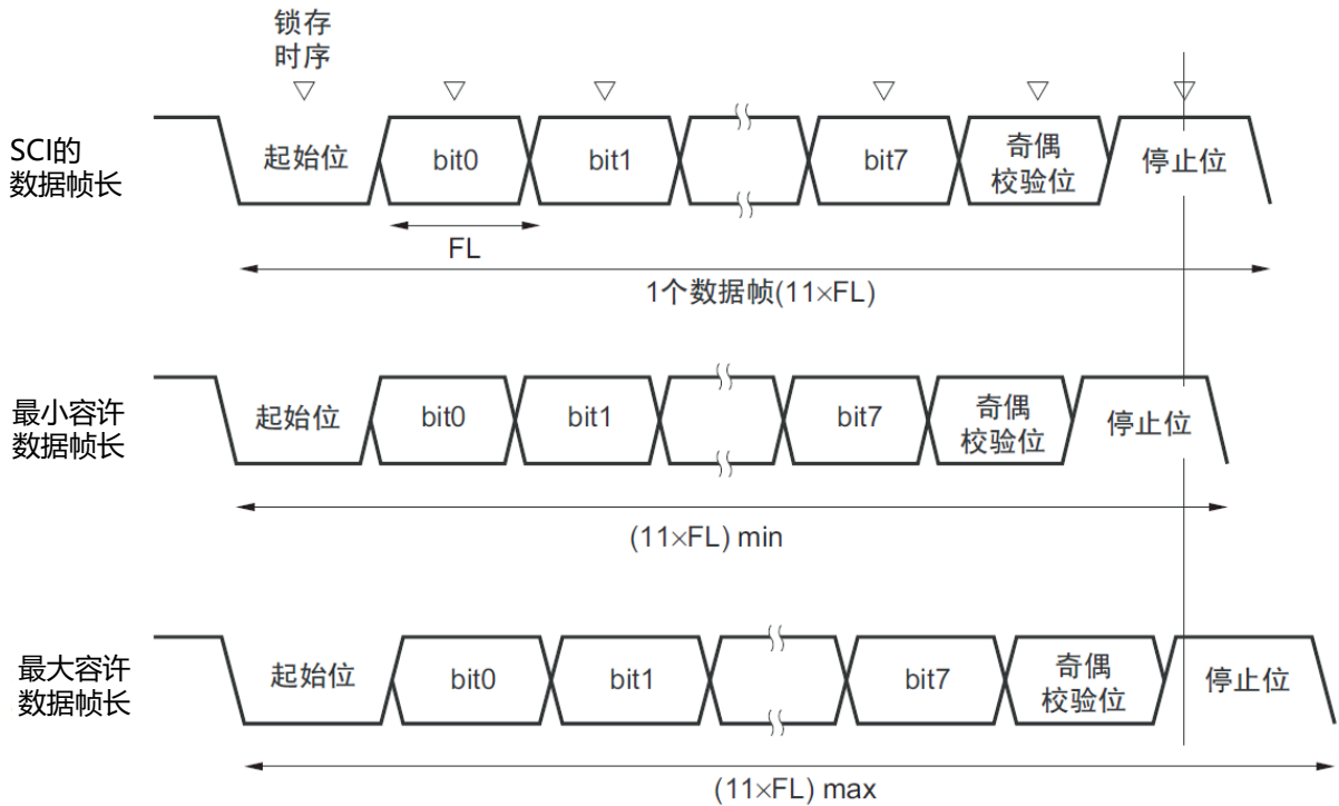
图19-120 接收时的波特率容许范围(1个数据的帧长=11位的情况)
