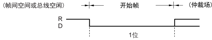
图21-5. 开始帧(SOF)
