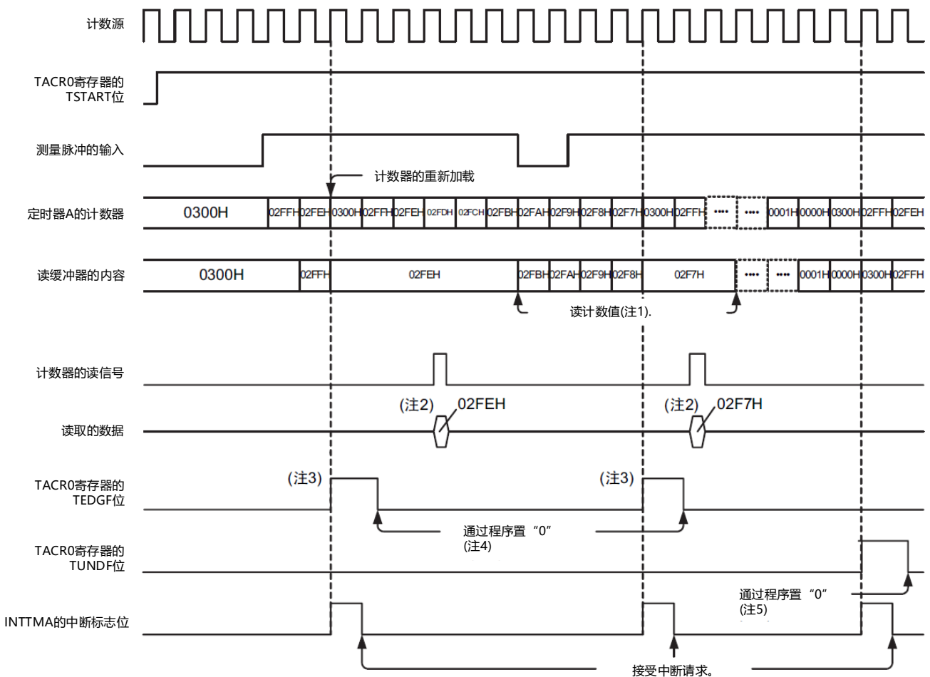
图7-15 脉冲周期测量模式的运行例子
