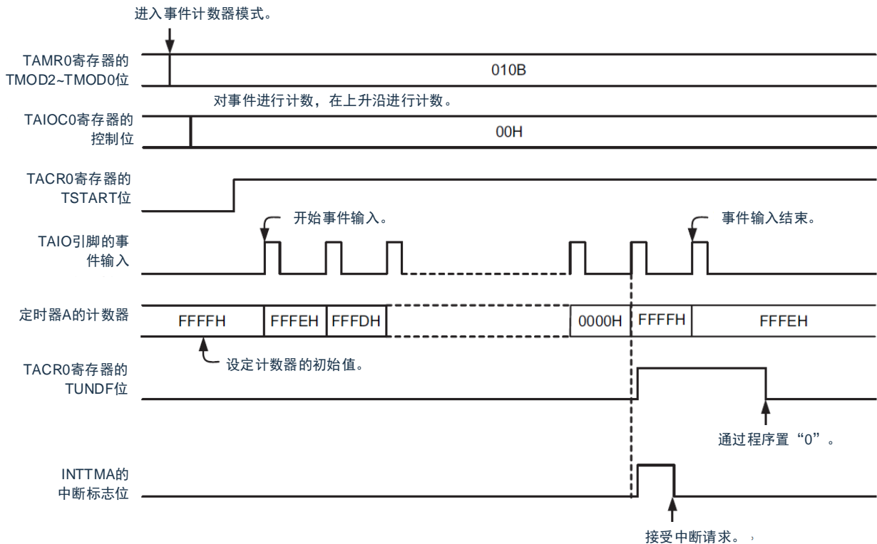
图7-12 事件计数器模式的运行例子1
