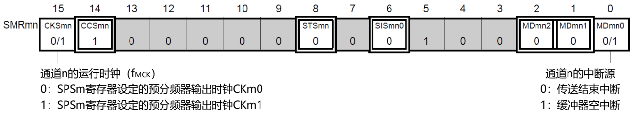
图19-49 3线串行I/O(SSPI00、SSPI01、SSPI10、SSPI11、SSPI20、SSPI21) 从属发送时的寄存器设置内容例子
