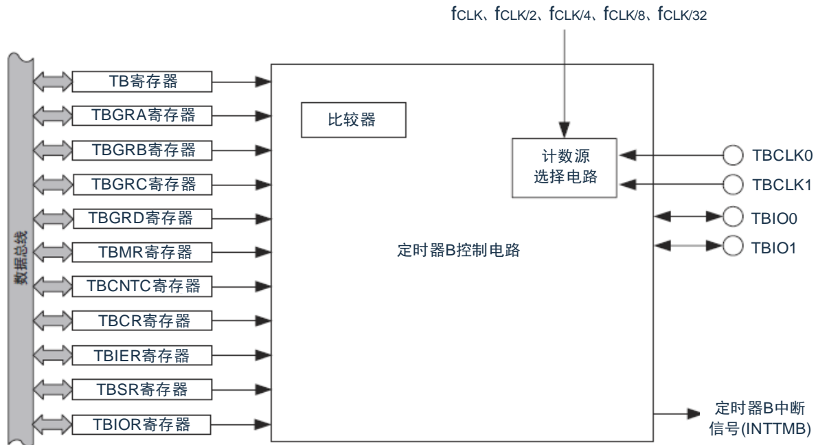
图8-1 定时器B的框图
