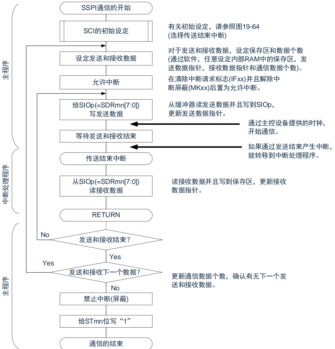
图19-68 从属发送和接收(单次发送和接收模式)的流程图
