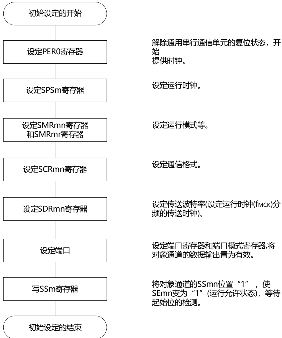
图19-110 UART接收的初始设置步骤
