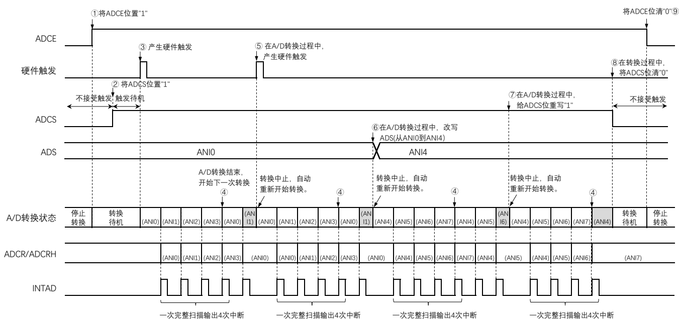
图15-23 硬件触发无等待模式(扫描模式、连续转换模式)的运行时序例子
