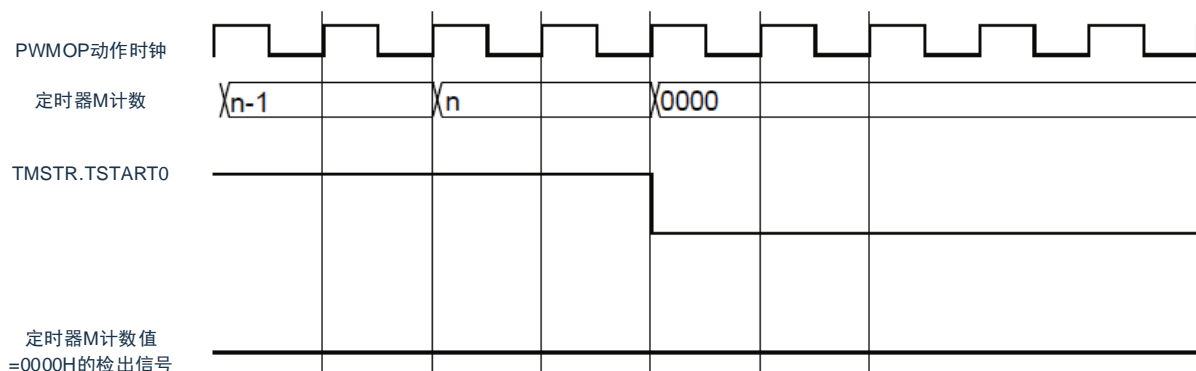
图10-90 计数值=0000H时的判定时序 (计数源=Fclk/2，定时器M计数值到达0000H的同时计数器停止)
