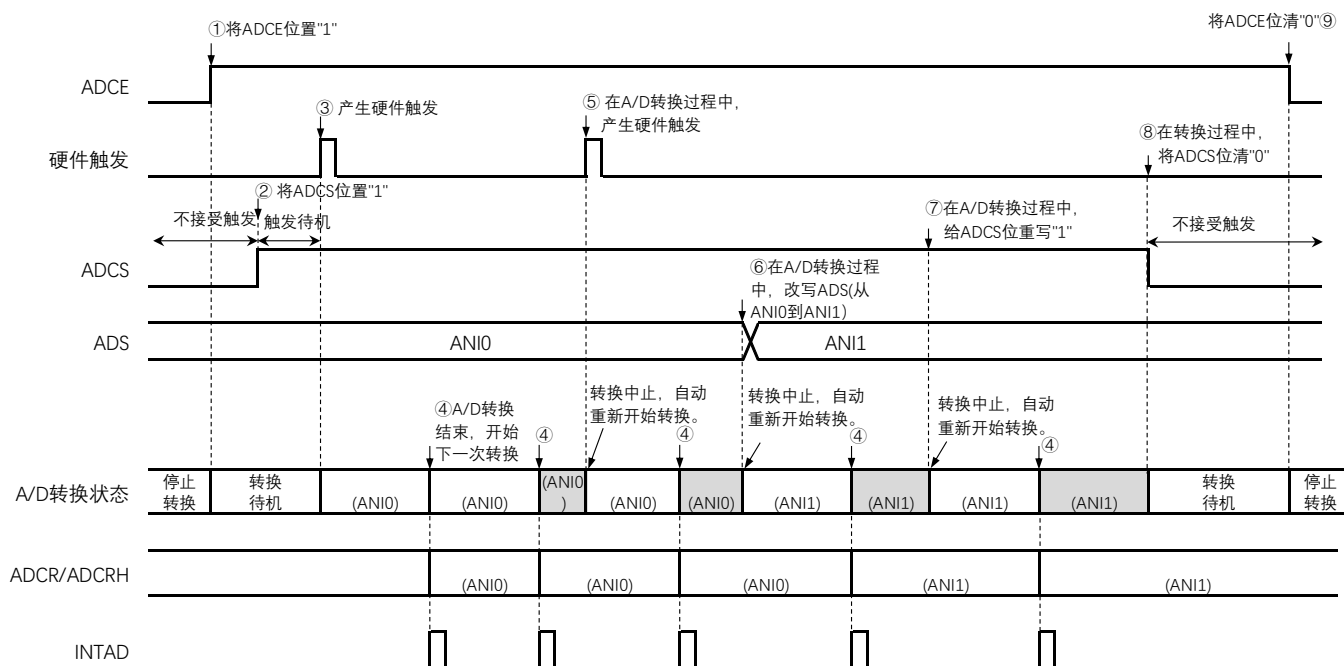
图15-21 硬件触发无等待模式(选择模式、连续转换模式)的运行时序例子
