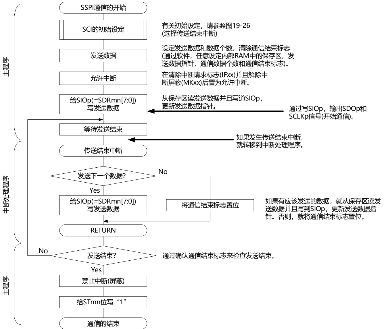
图19-30 主控发送(单次发送模式)的流程图
