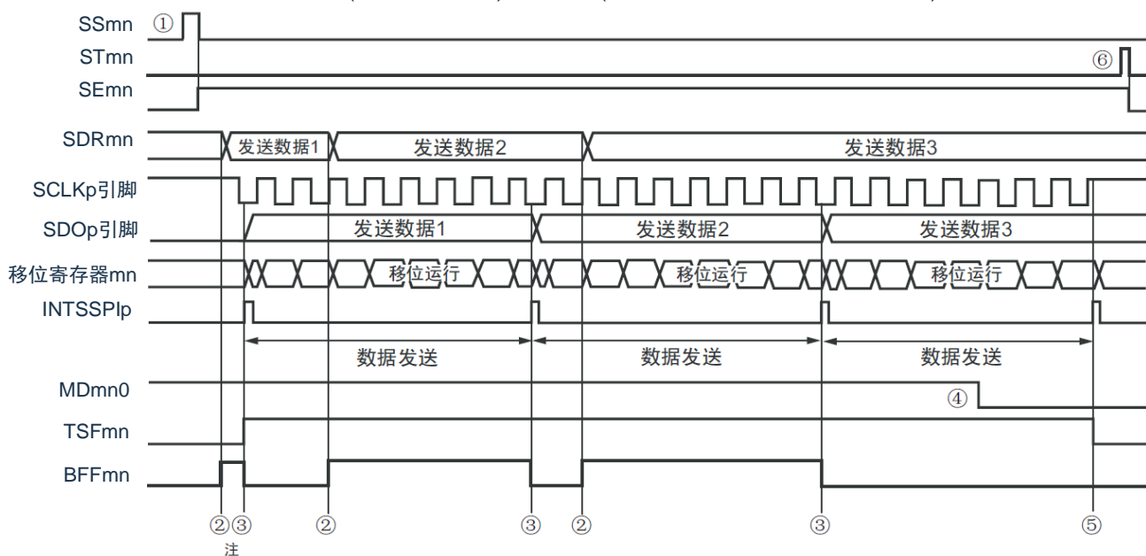
图19-55 从属发送(连续发送模式)的时序图(类型1: DAPmn=0、CKPmn=0)
