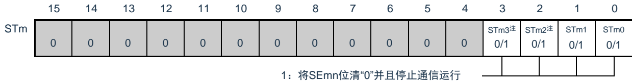
图19-24 按通道停止运行时的各寄存器的设置
