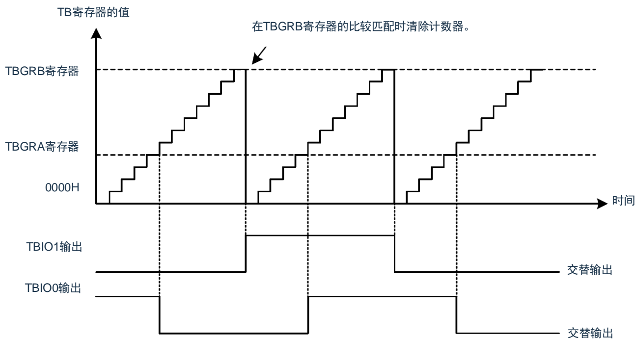
图8-22 交替输出的运行例子
