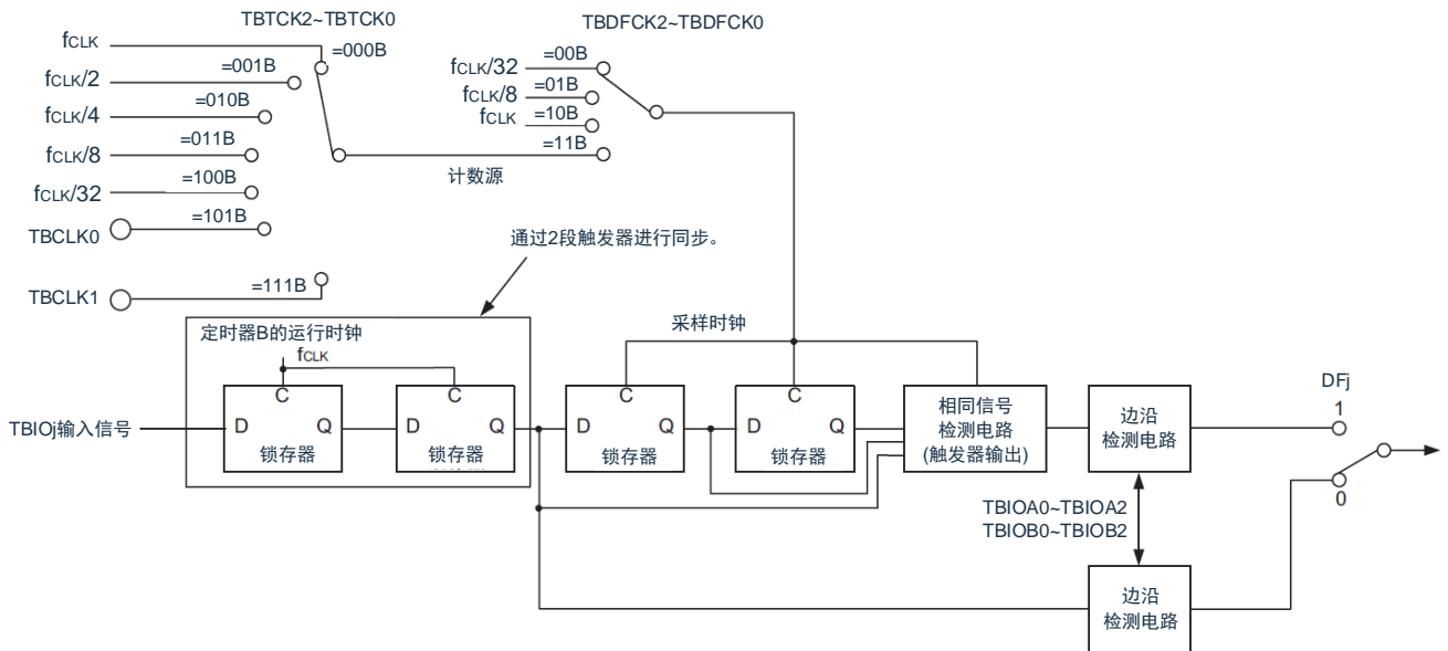
图8-15 数字滤波器的框图
