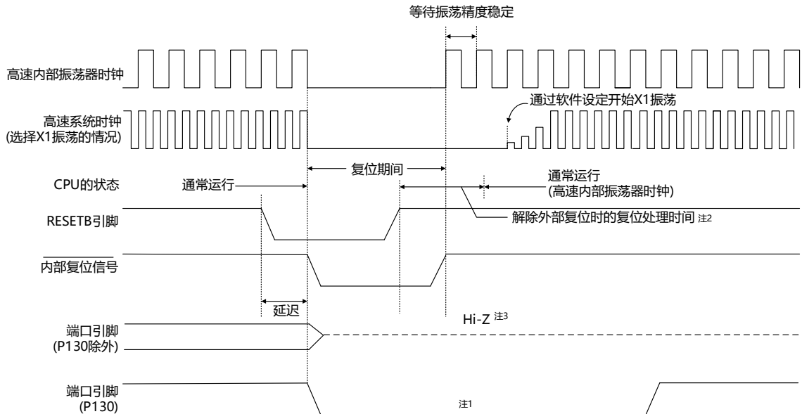
图28-2 RESETB输入的复位时序
