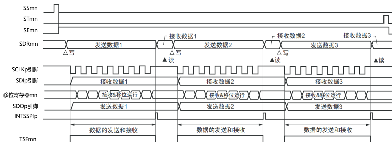
图19-45 主控发送和接收(单次发送和接收模式)的时序图(类型1: DAPmn=0、CKPmn=0)
