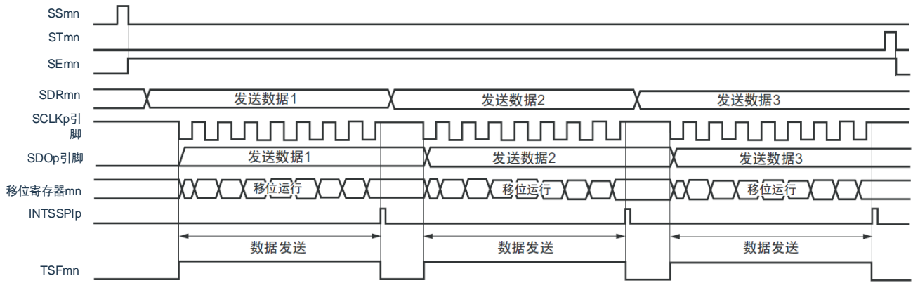
图19-53 从属发送(单次发送模式)的时序图(类型1: DAPmn=0、CKPmn=0)
