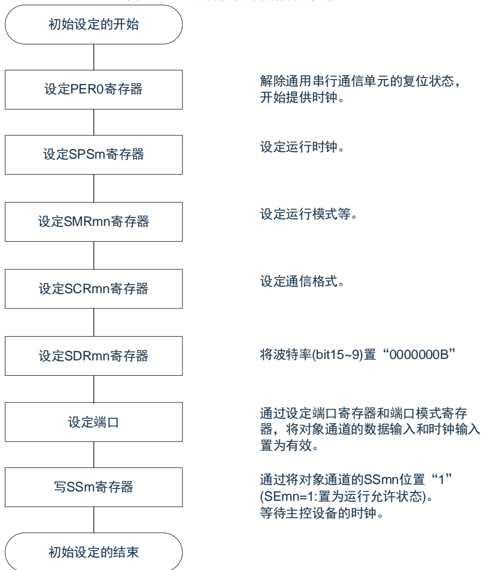
图19-58 从属接收的初始设置步骤
