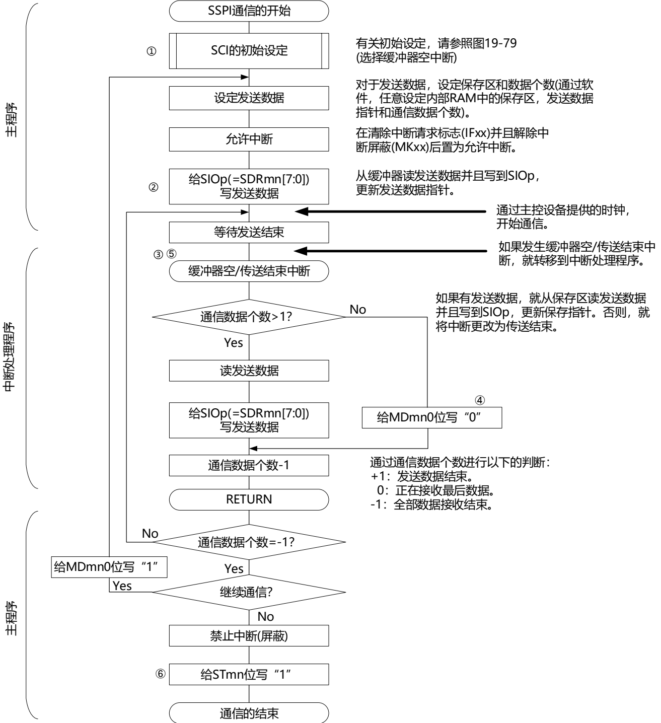
图19-85 从属发送(连续发送模式)的流程图
