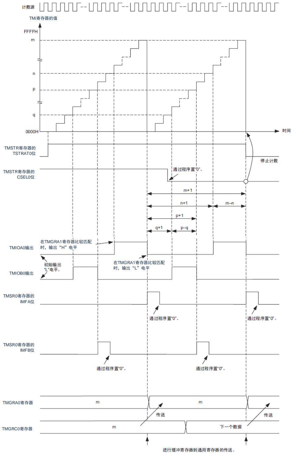
图10-62 PWM3模式的运行例子
