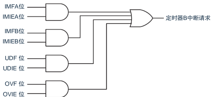
图8-31 定时器B中断的框图
