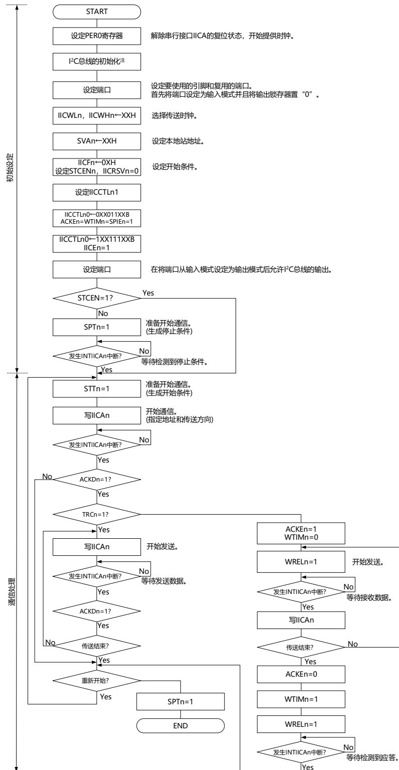
图20-28 单主控系统的主控运行
