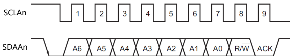
图20-18 应答
