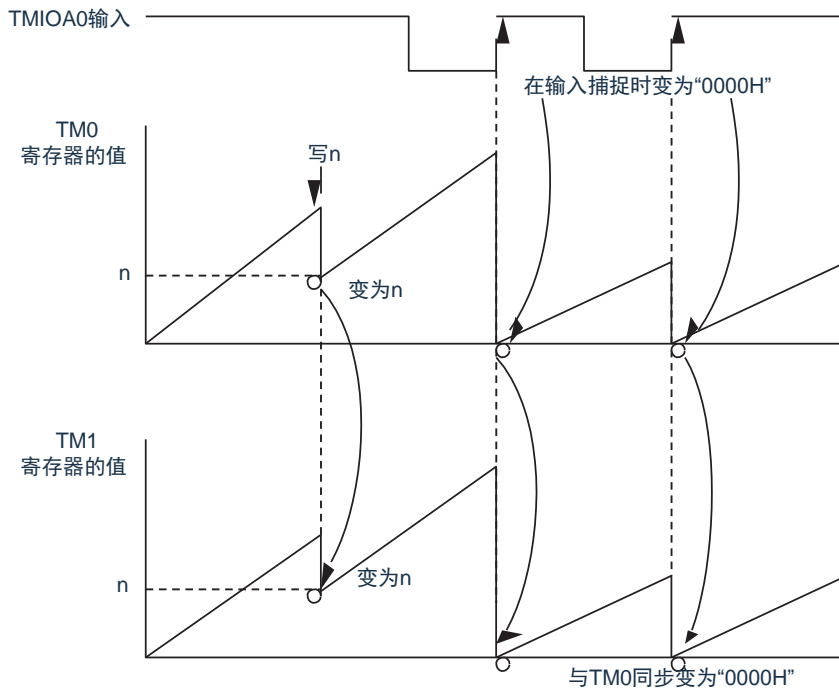
图10-44 同步运行
