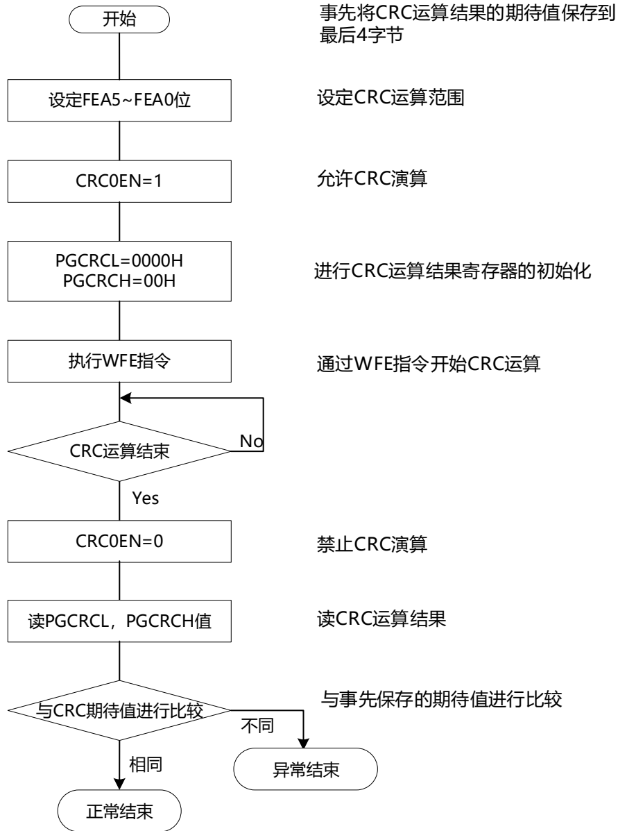
图31-3 闪存CRC运算功能(高速CRC)的流程图
