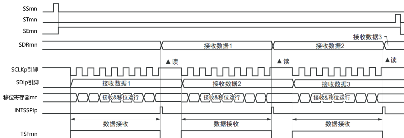
图19-61 从属接收(单次接收模式)的时序图(类型1: DAPmn=0、CKPmn=0)
