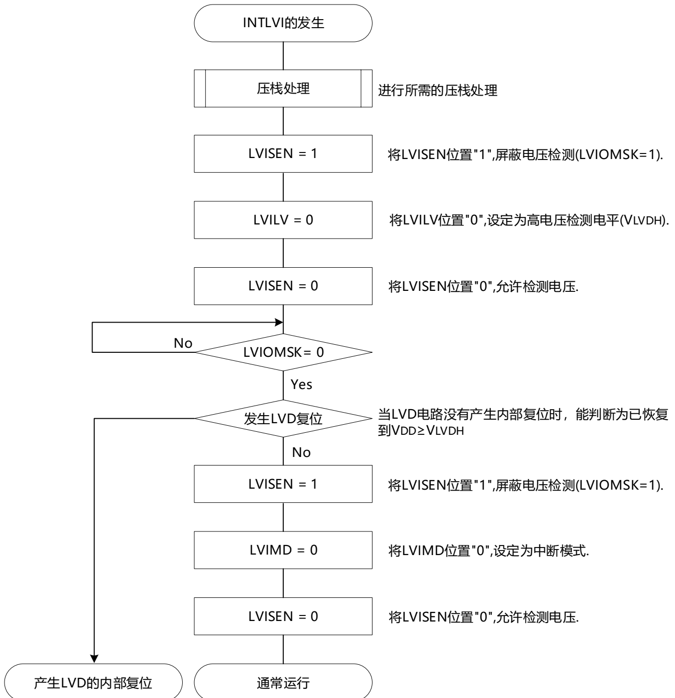
图30-7 工作电压的确认/复位的设置步骤
