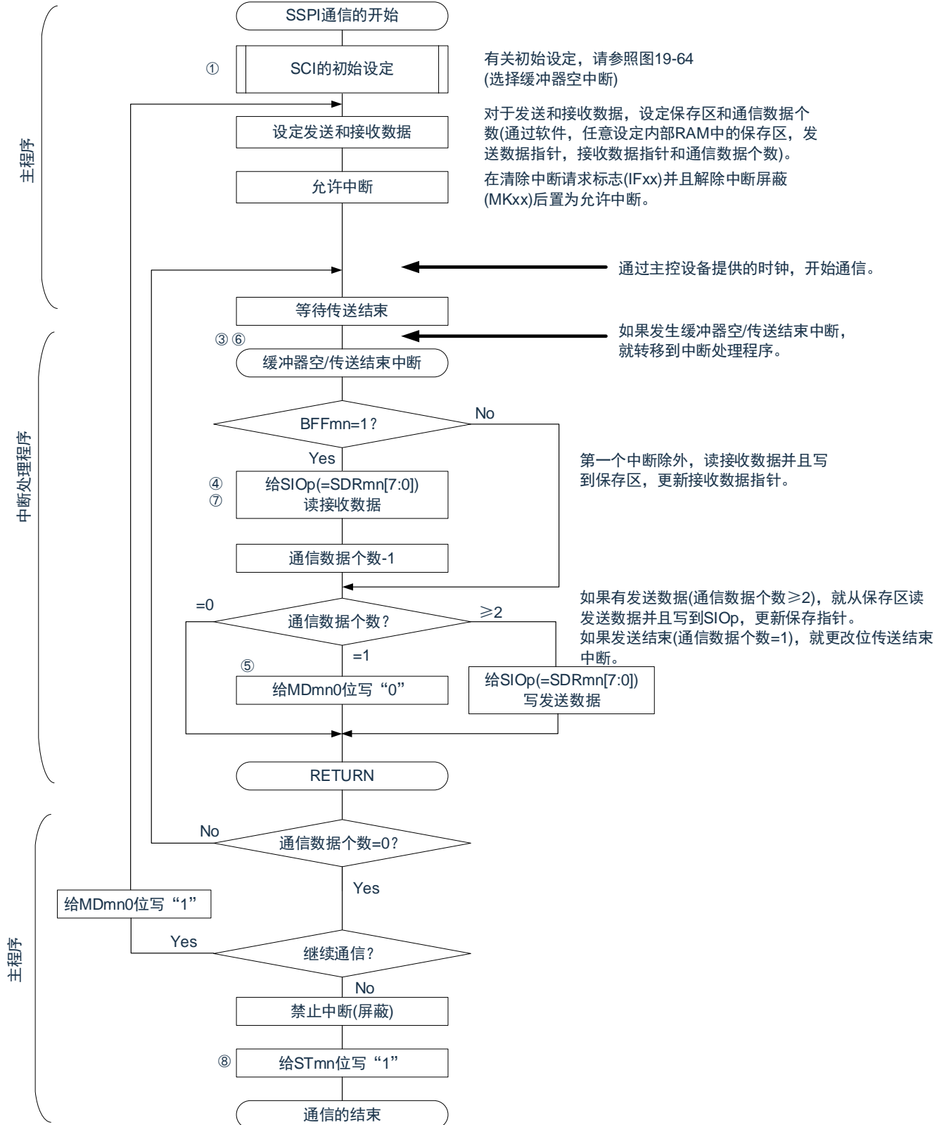
图19-70 从属发送和接收(连续发送和接收模式)的流程图
