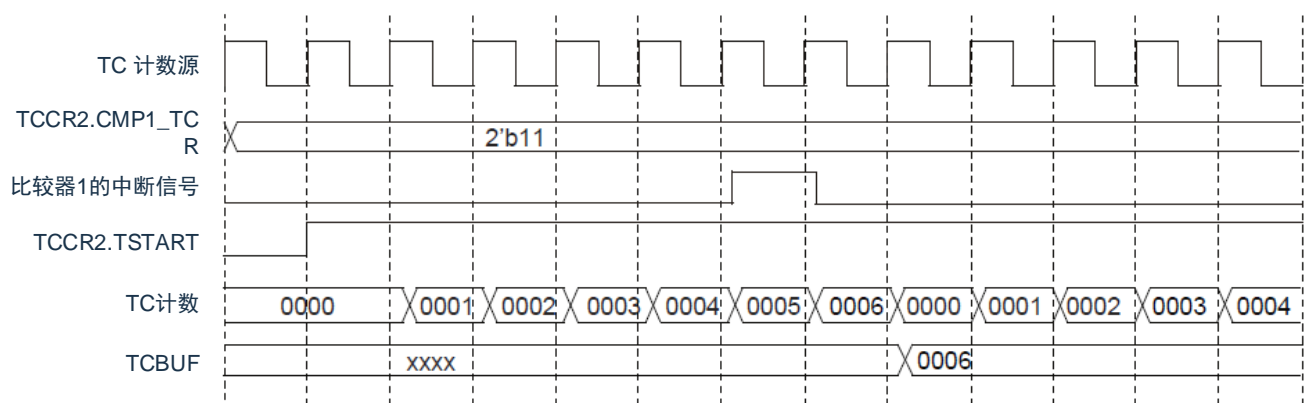
图9-13 输入捕捉的动作例子(同时复位计数值)
