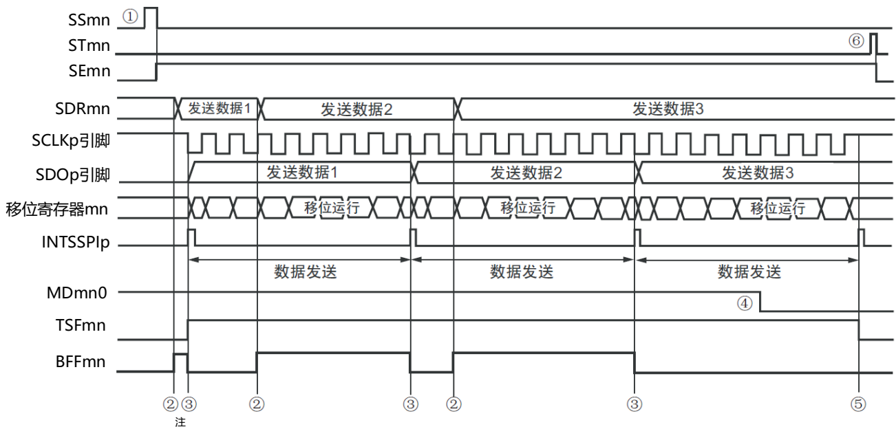
图19-31 主控发送(连续发送模式)的时序图(类型1: DAPmn=0、CKPmn=0)
