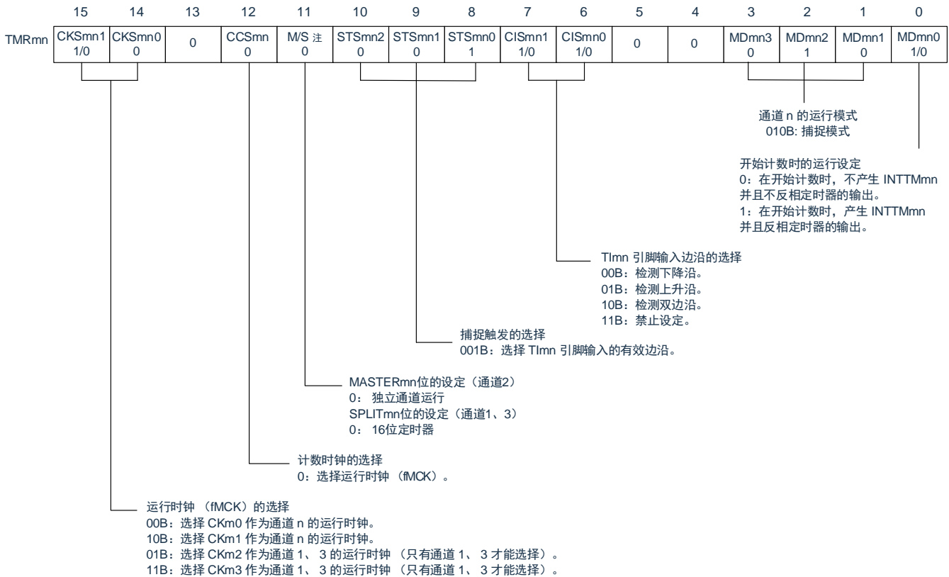
图6-52 测量输入脉冲间隔时的寄存器设置内容例子
