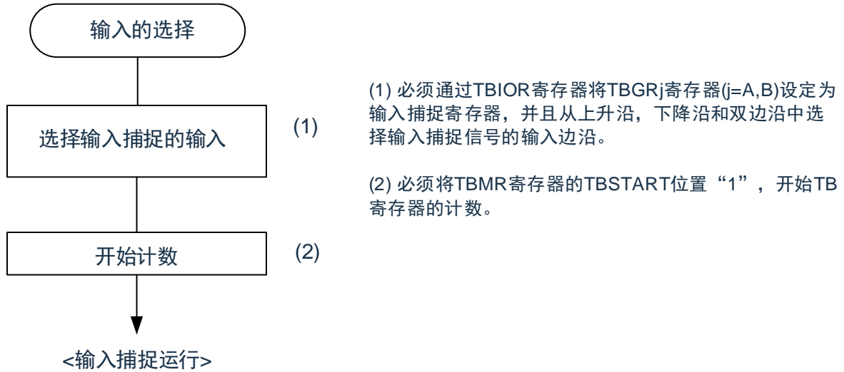
图8-16 输入捕捉运行的设置步骤例子
