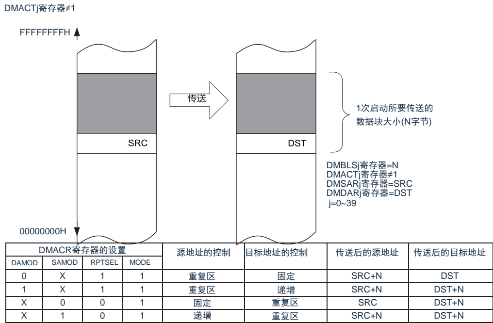
图23-18 重复模式的数据传送
