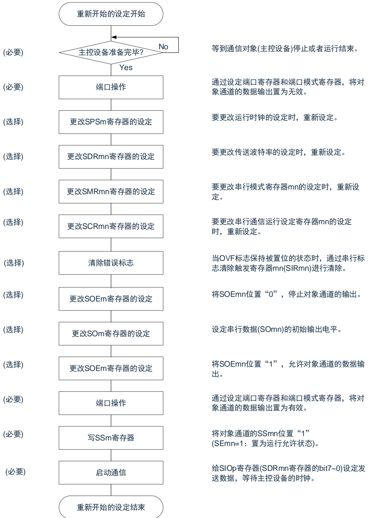
图19-52 重新开始从属发送的设置步骤
