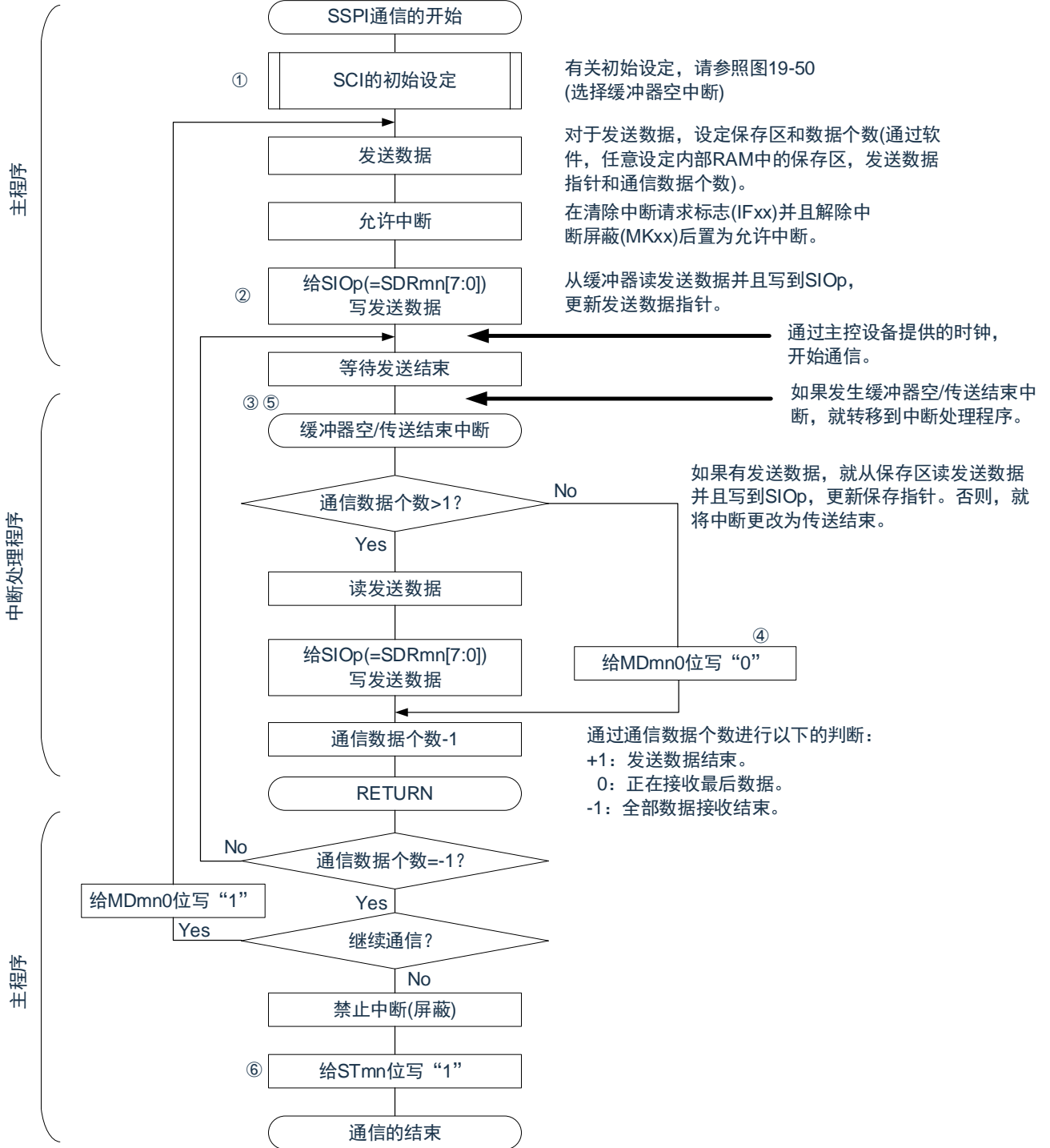
图19-56 从属发送(连续发送模式)的流程图
