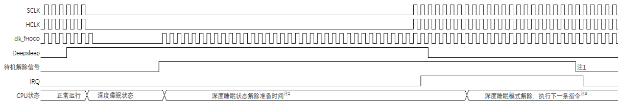
图27-3 通过中断请求解除深度睡眠模式
