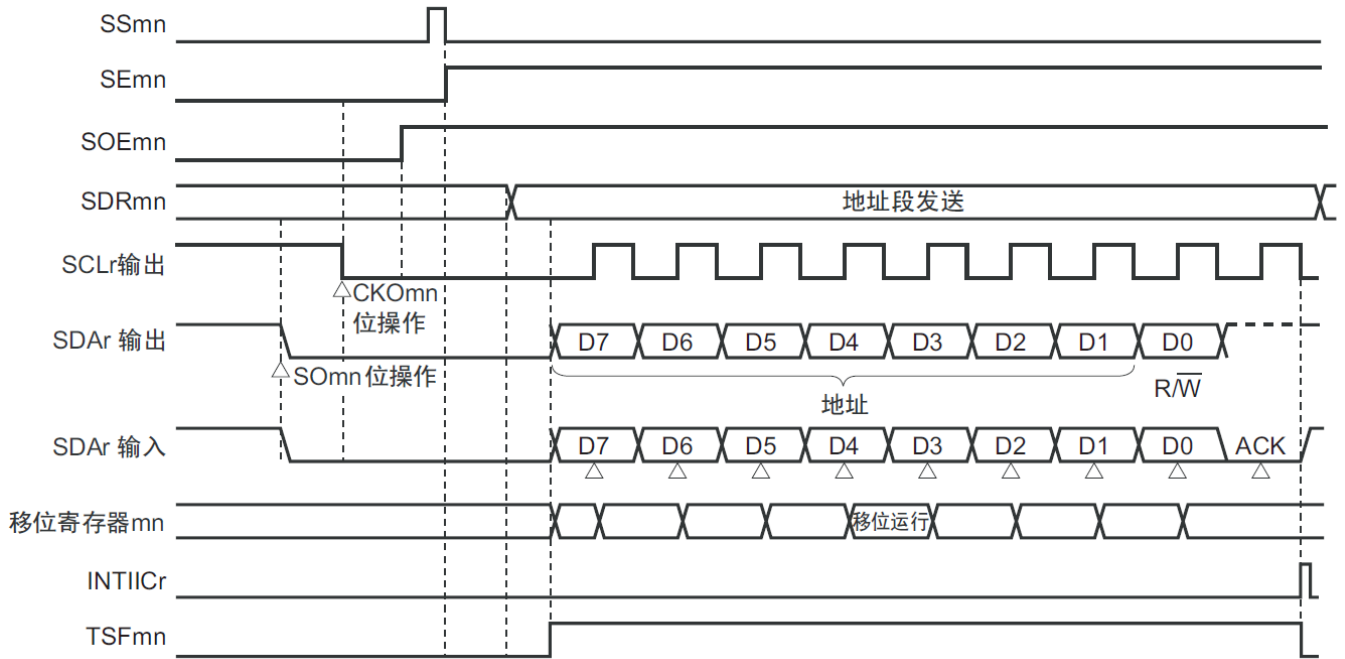
图19-130 地址段发送的时序图
