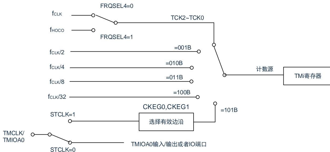
图10-41 计数源的框图
