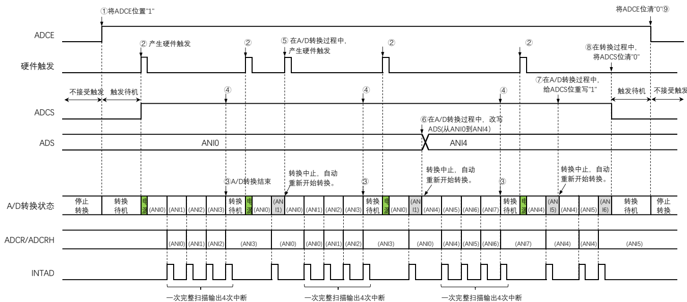
图15-28 硬件触发等待模式(扫描模式、单次转换模式)的运行时序例子
