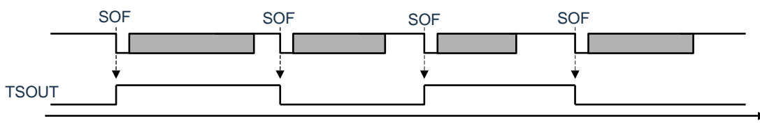
图21-61. 捕获信号 TSOUT 的时序图
