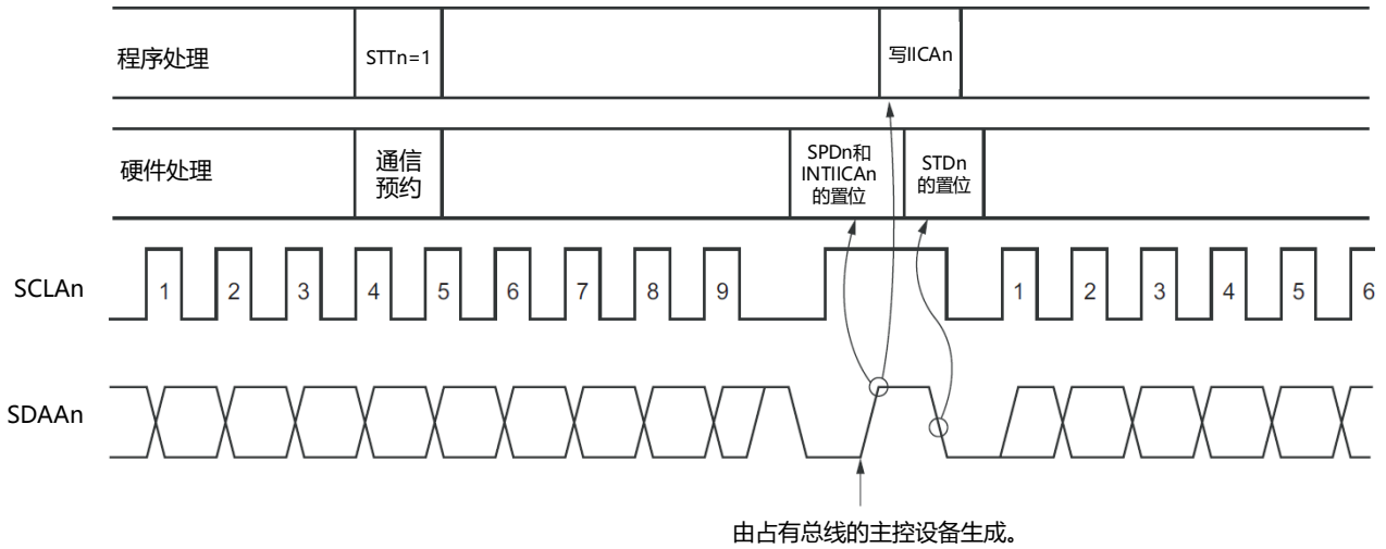
图20-25 通信预约的时序
