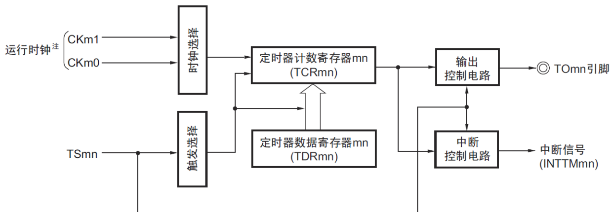
图6-41 作为间隔定时器/方波输出运行的基本时序例子(MDmn0=1)
