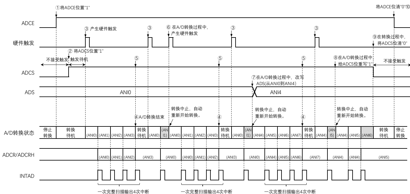
图15-24 硬件触发无等待模式(扫描模式、单次转换模式)的运行时序例子
