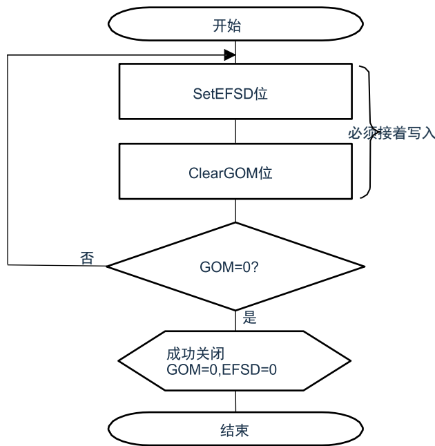
图21-85. 强制关闭处理
