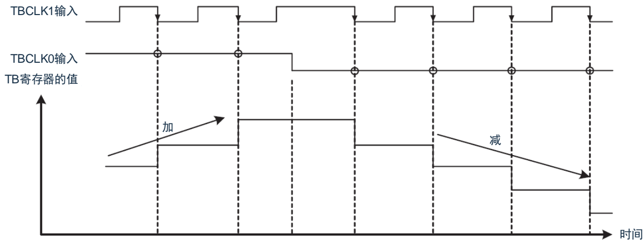
图8-29 相位计数模式的运行例子3
