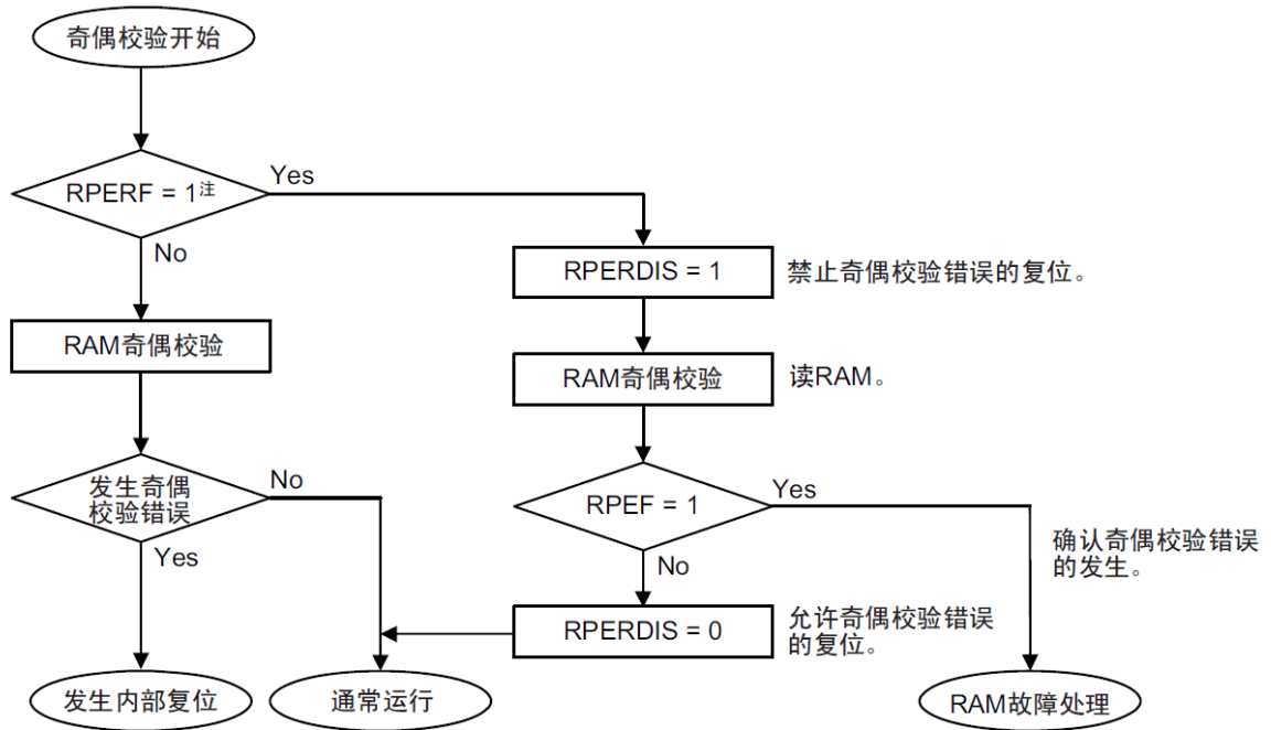
图31-8 RAM奇偶校验的流程
