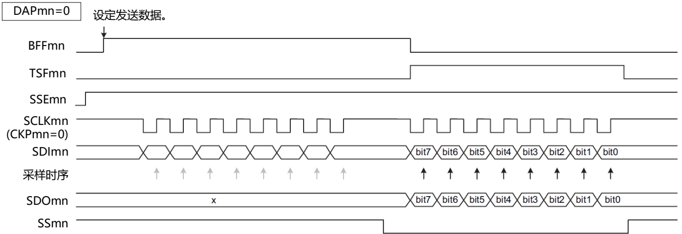
图19-77 从属选择输入功能的时序图
