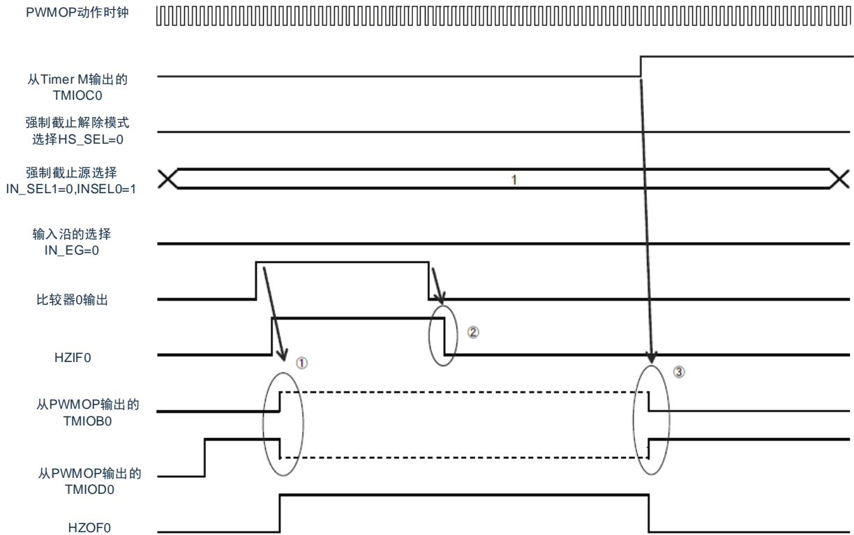
图10-78 硬件解除强制截止的例子(以TMIOB0, TMIOD0为例)
