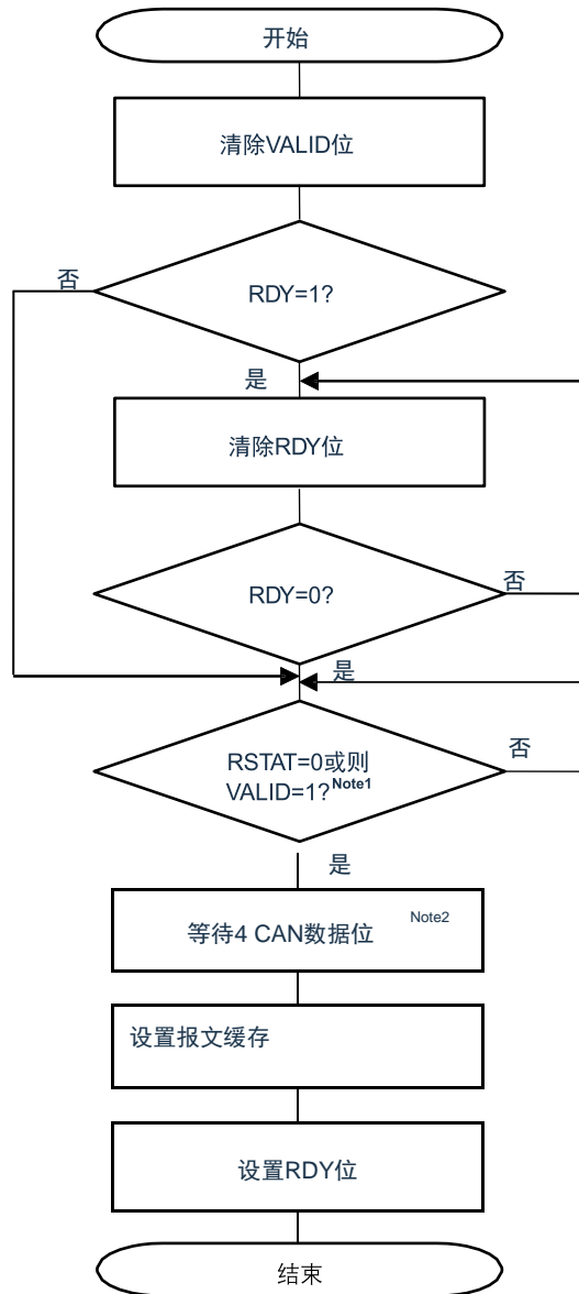
图21-66. 报文缓存重定义
