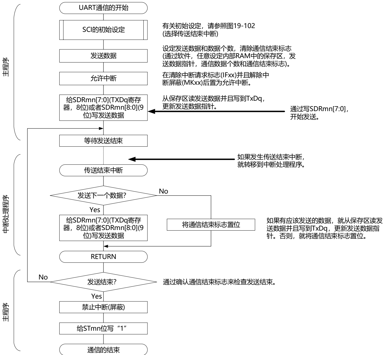
图19-106 UART发送(单次发送模式)的流程图
