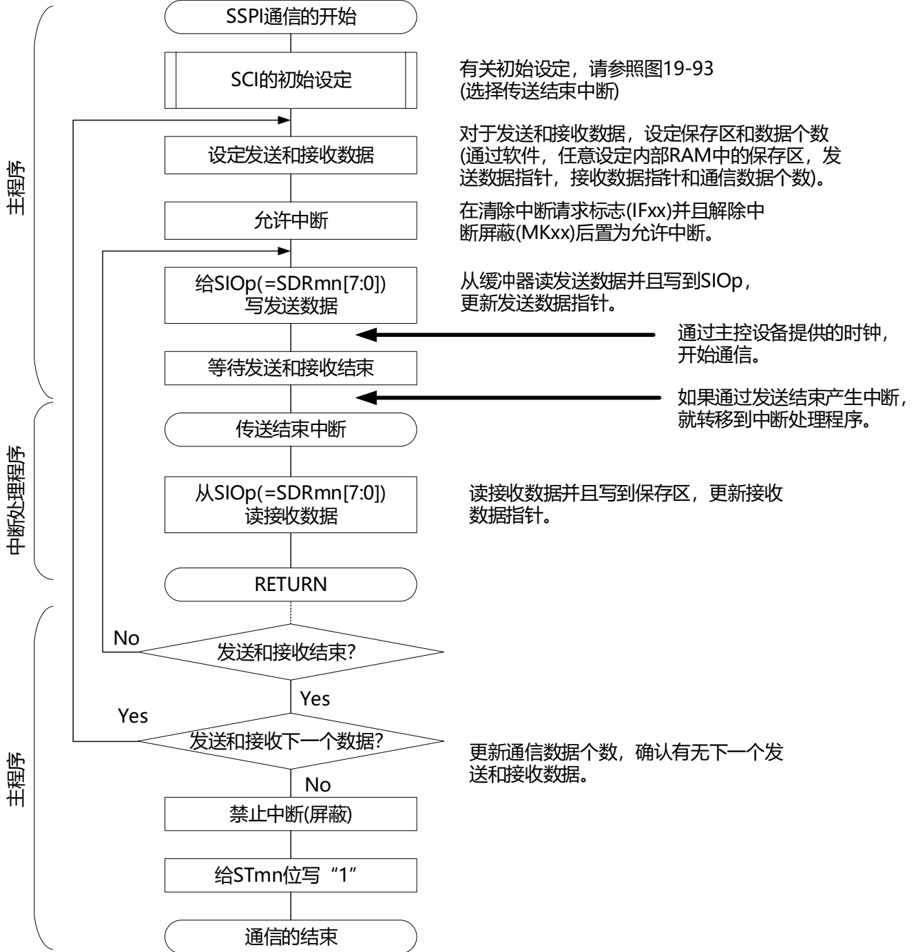
图19-97 从属发送和接收(单次发送和接收模式)的流程图
