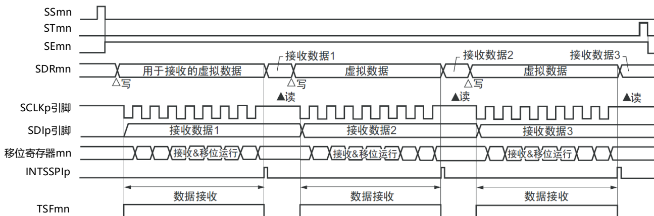
图19-37 主控接收(单次接收模式)的时序图(类型1: DAPmn=0、CKPmn=0)
