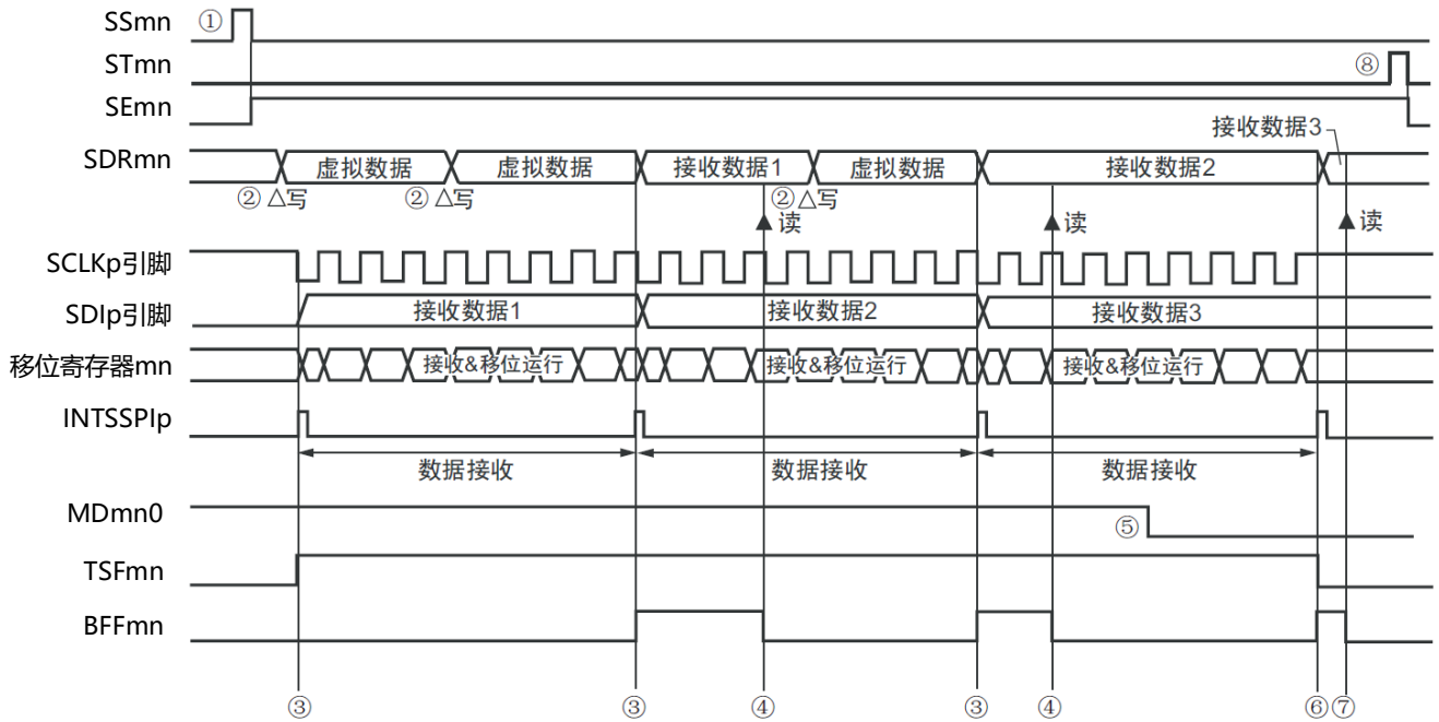
图19-39 主控接收(连续接收模式)的时序图(类型1: DAPmn=0、CKPmn=0)
