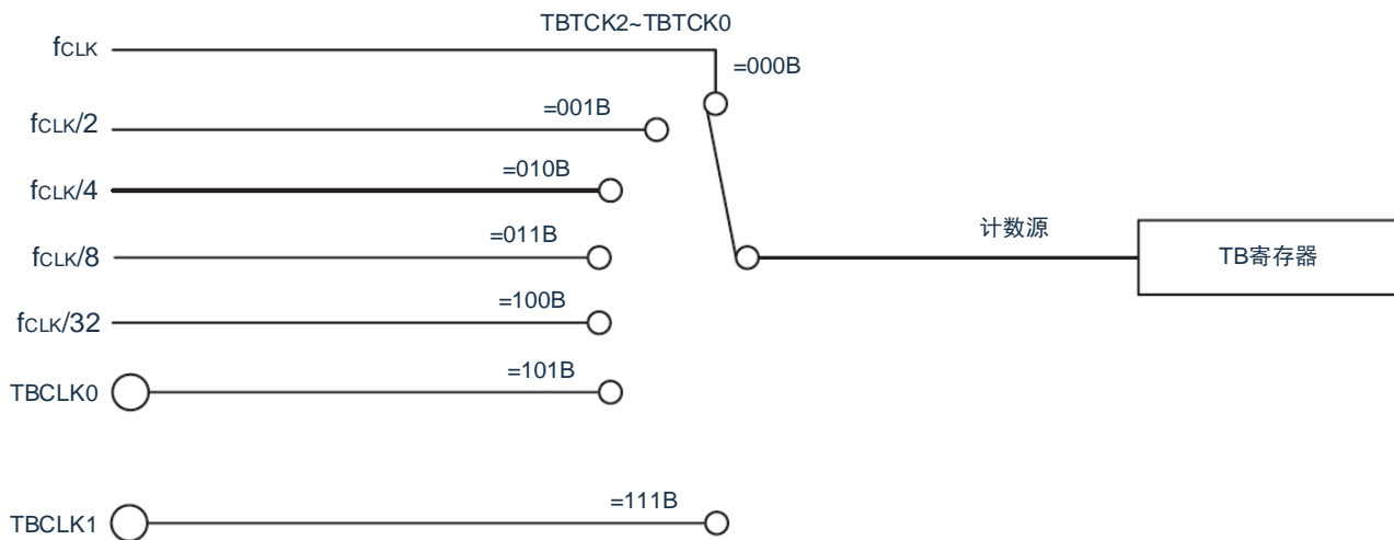
图8-12 计数源的框图
