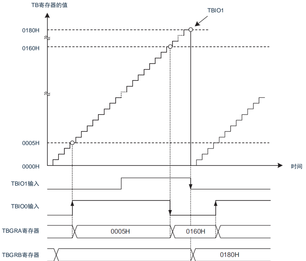
图8-18 输入捕捉的运行例子
