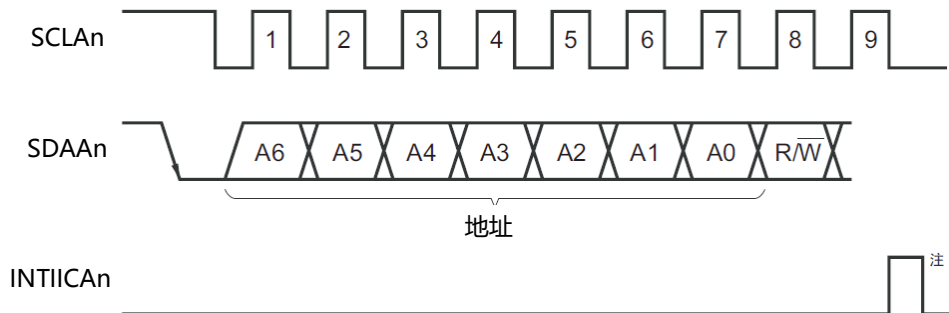
图20-16 地址
