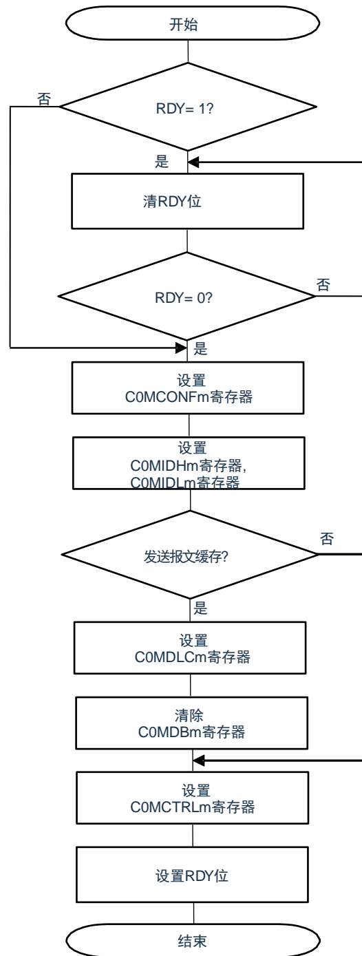
图21-65. 报文缓存初始化
