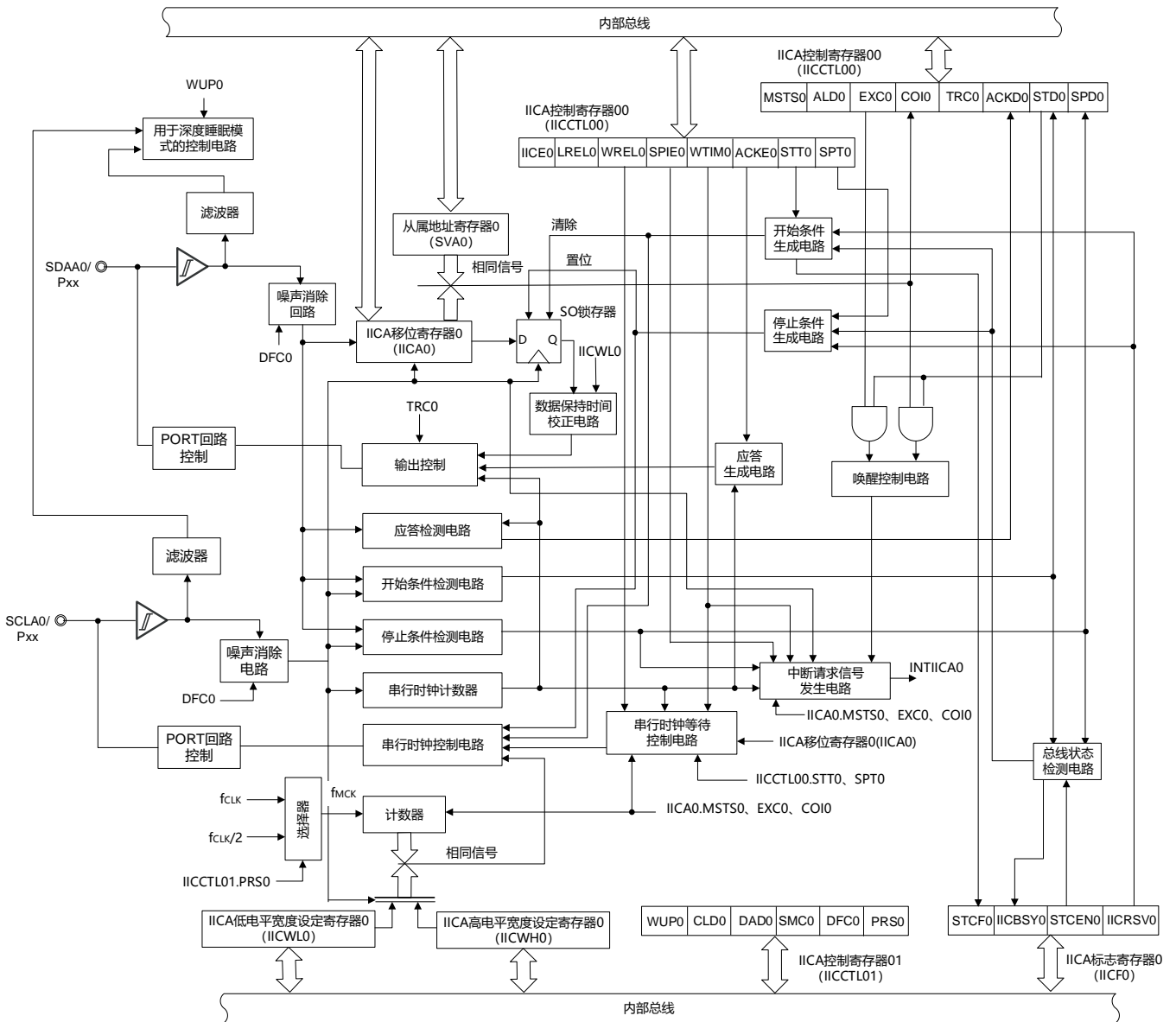
图20-1 串行接口IICA的框图
