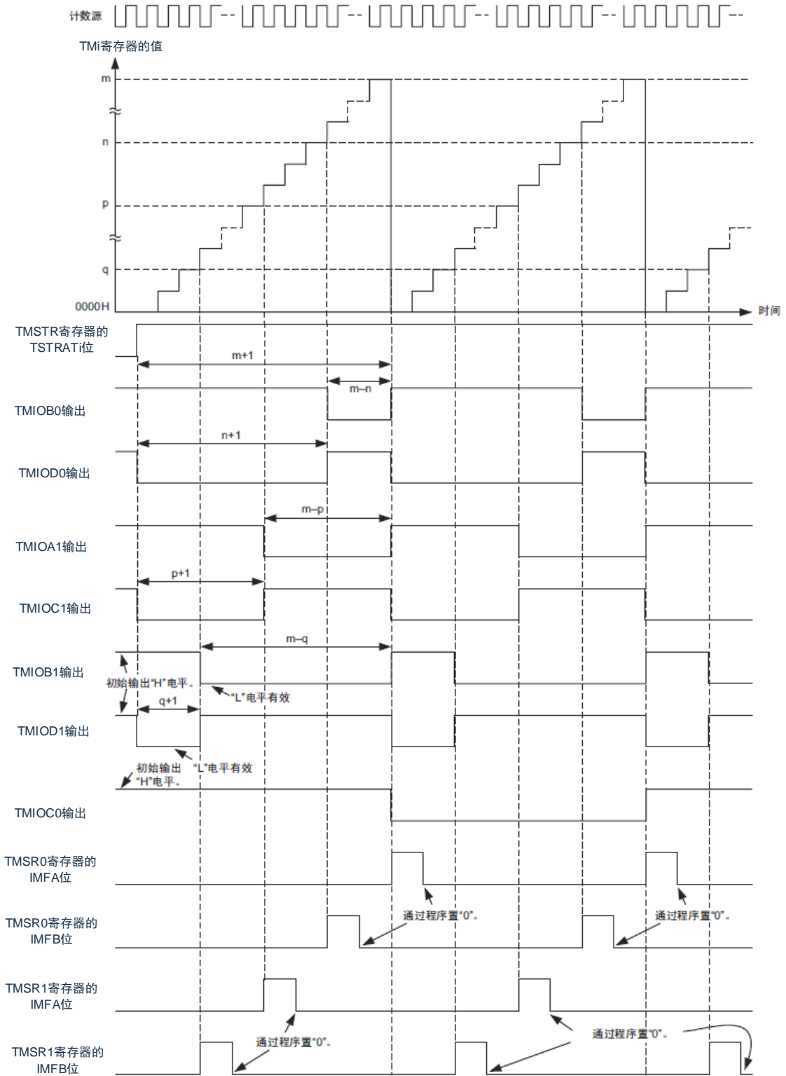
图10-57 复位同步PWM模式的运行例子
