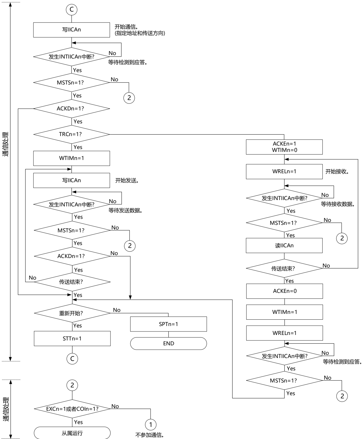
图20-29 多主控系统的主控运行(3/3)
