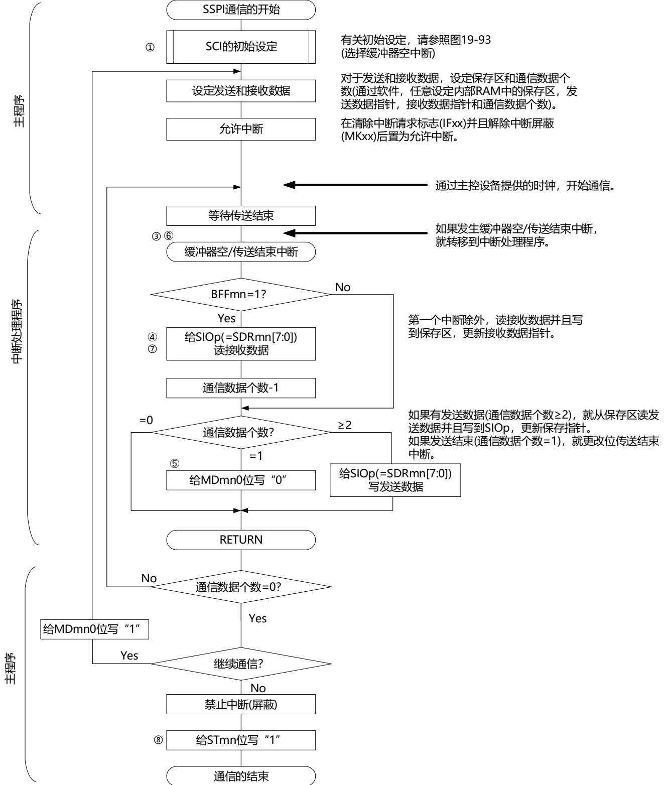
图19-99 从属发送和接收(连续发送和接收模式)的流程图
