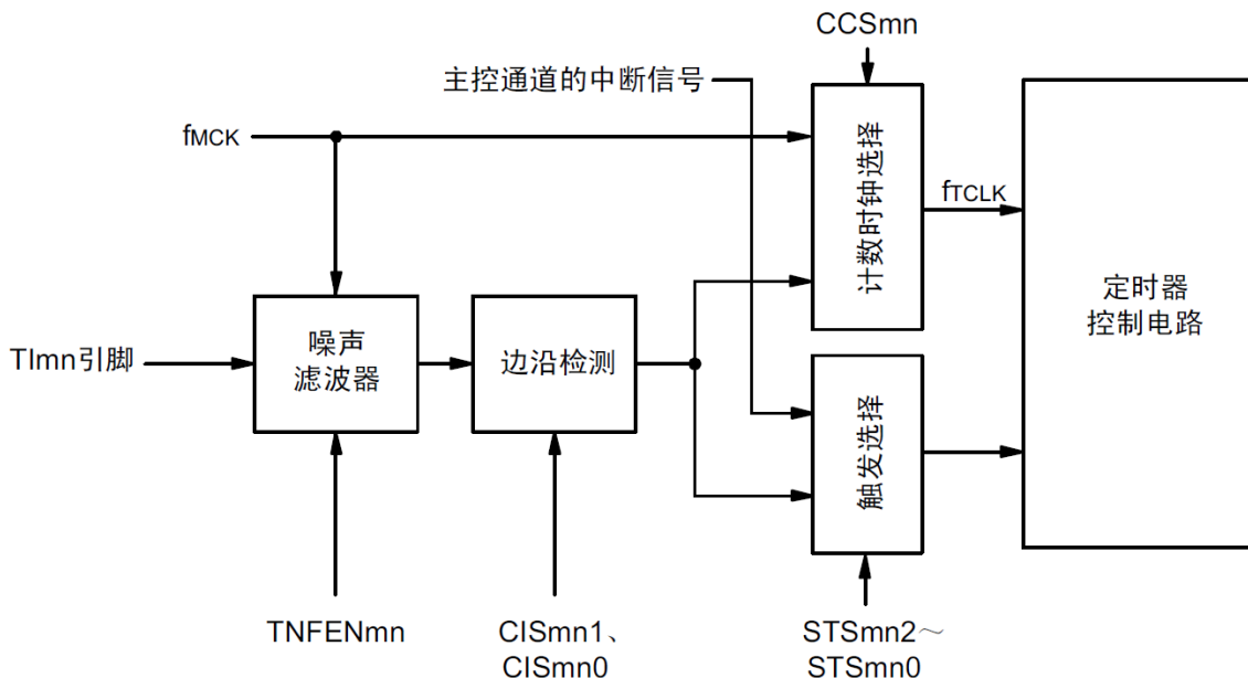
图6-40 输入电路的结构
