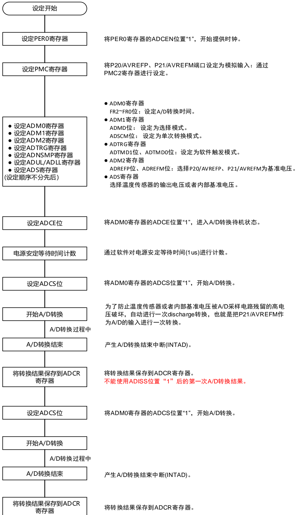
图15-33 选择温度传感器的输出电压/内部基准电压时的设置
