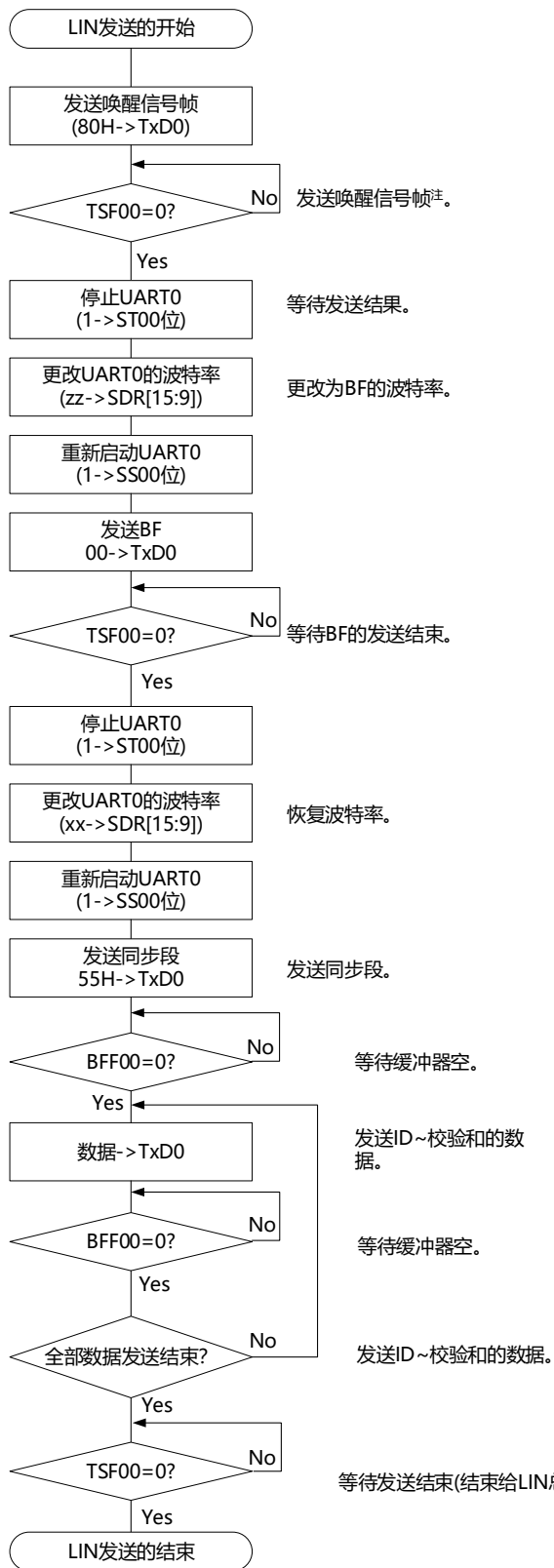
图19-124 LIN发送的流程图
