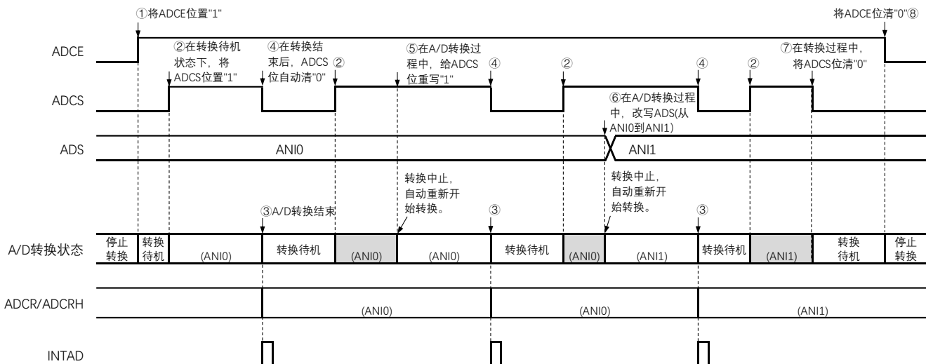
图15-18 软件触发模式(选择模式、单次转换模式)的运行时序例子
