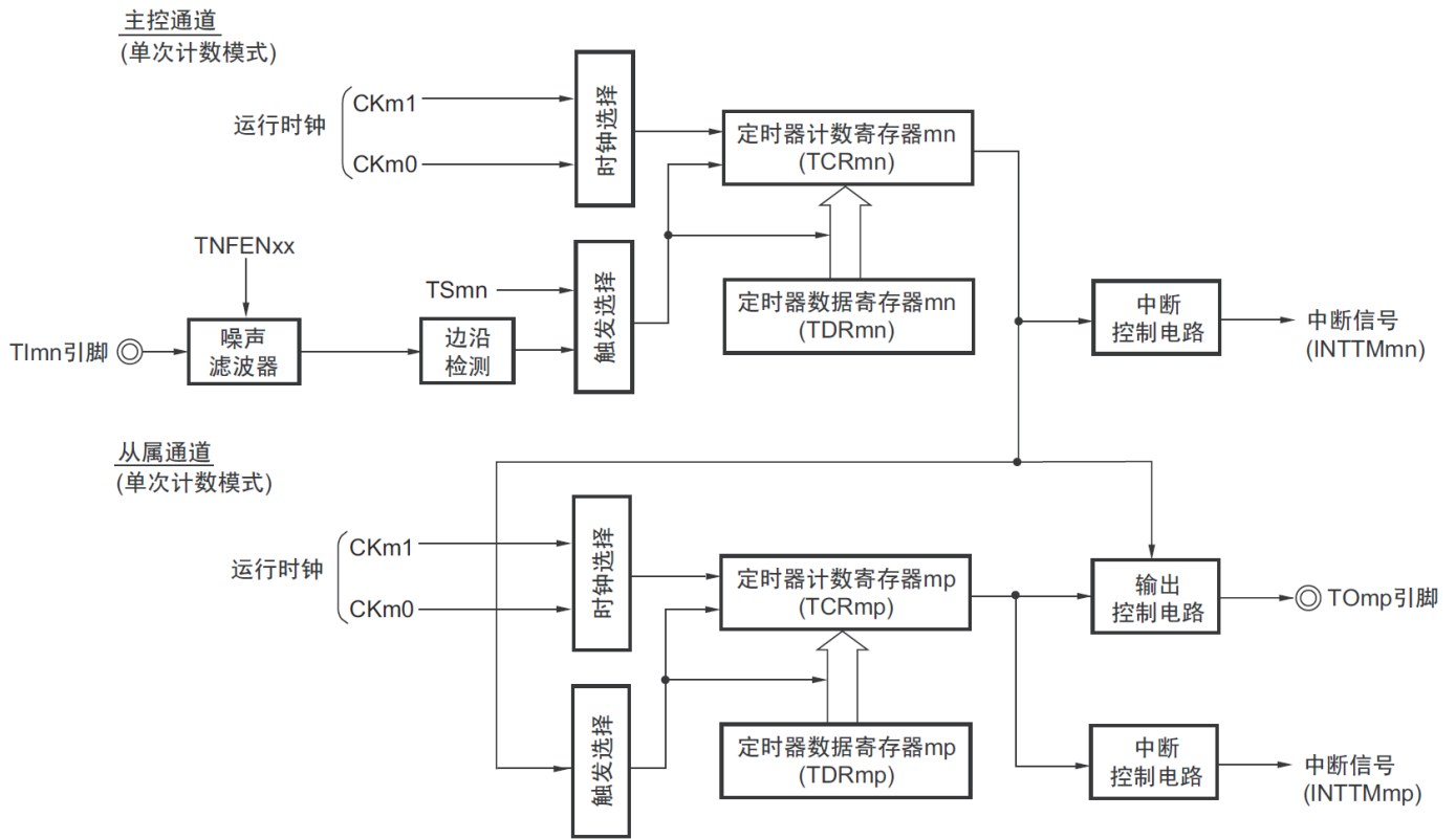
图6-60 作为单触发脉冲输出功能运行的框图
