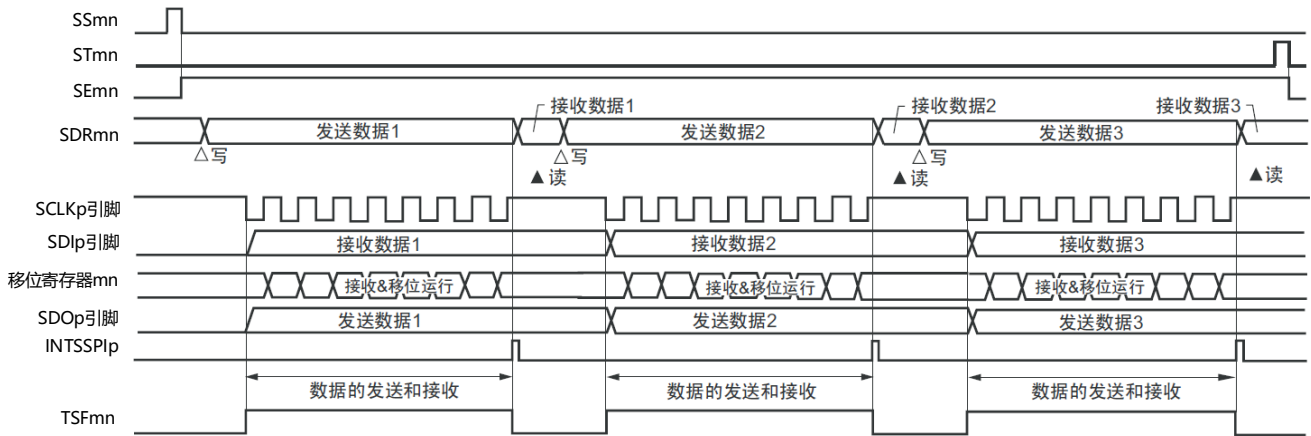
图19-67 从属发送和接收(单次发送和接收模式)的时序图(类型1: DAPmn=0、CKPmn=0)
