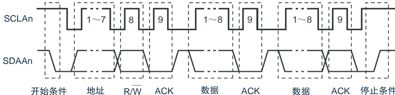
图20-14 I 2 C总线的串行数据传送时序
