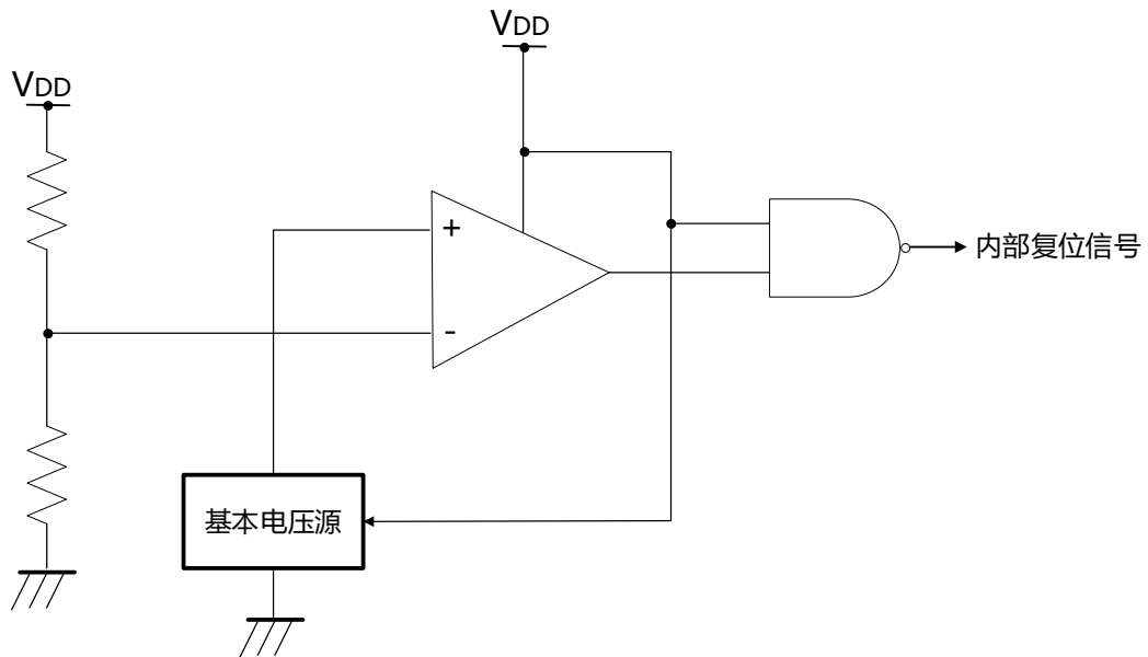
图29-1 上电复位电路的框图
