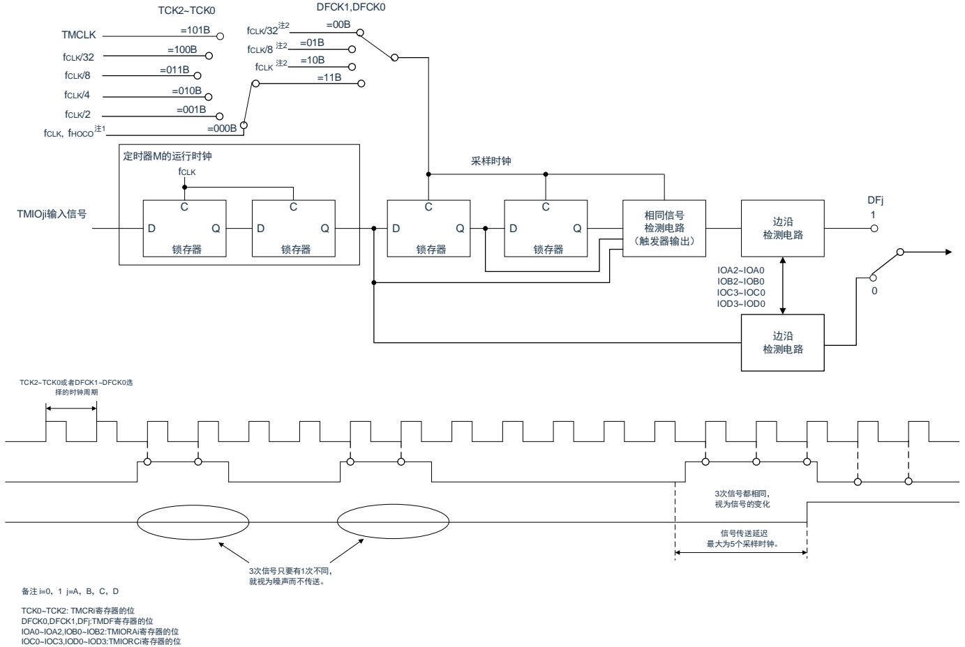
图 10-48 数字滤波器的框图
