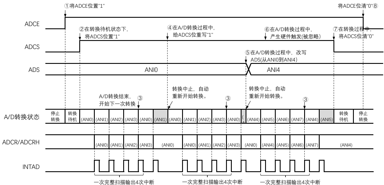
图15-19 软件触发模式(扫描模式、连续转换模式)的运行时序例子
