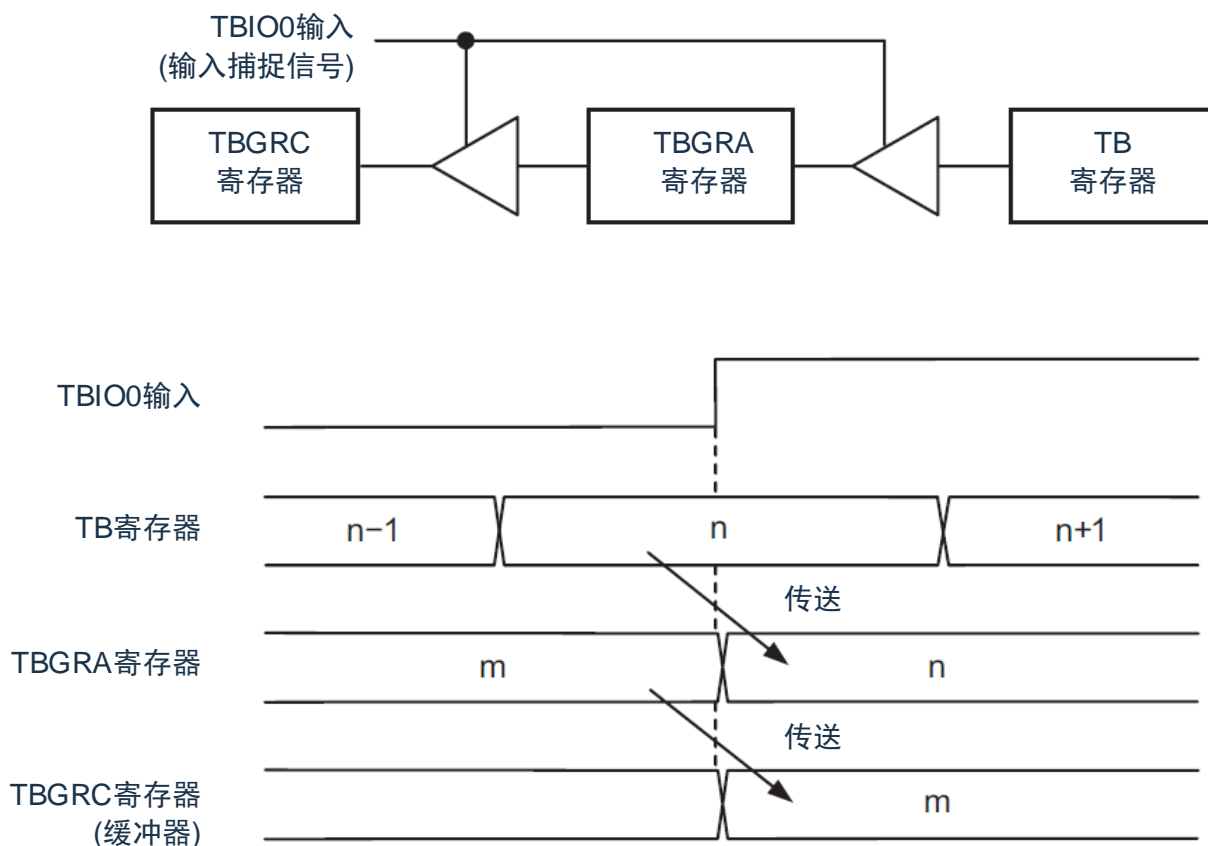
图8-13 输入捕捉功能的缓冲器运行
