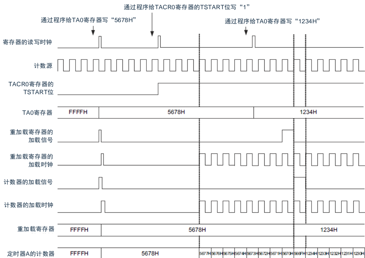
图7-9 由TSTART位的值决定的改写时序图
