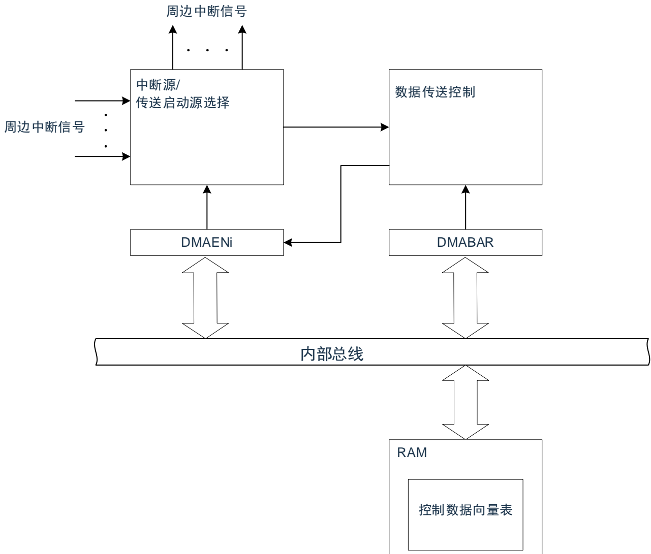
图23-1 DMA的框图
