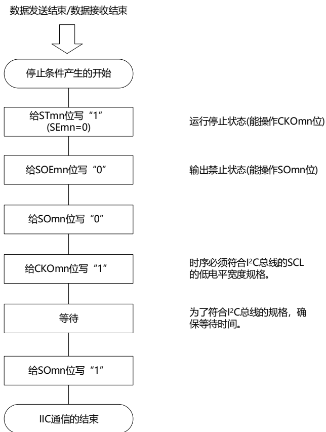
图19-139 产生停止条件的流程图
