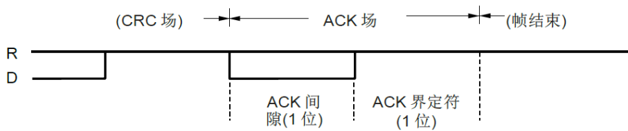
图21-11. 应答场
