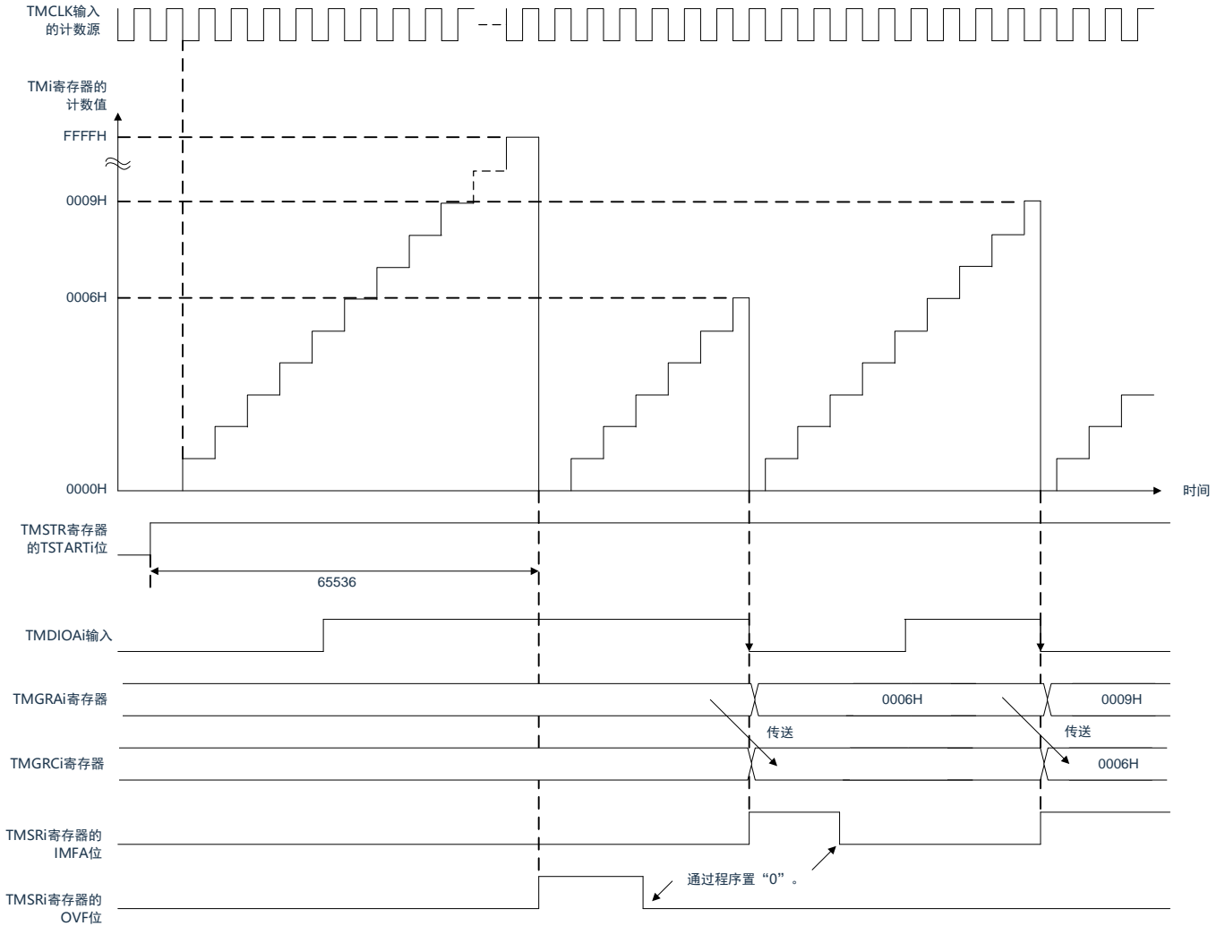
图10-47 输入捕捉功能的运行例子
