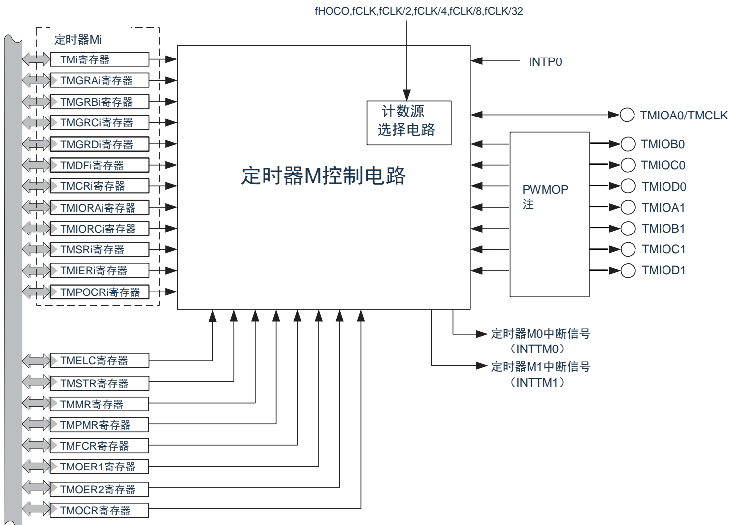
图10-1 定时器M的框图
