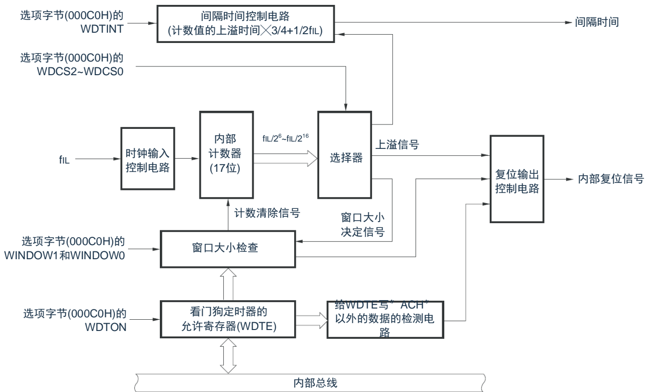
图14-1 看门狗定时器的框图
