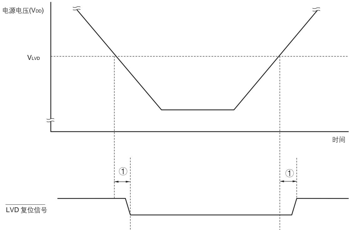
图30-10 从产生LVD复位源到产生或者解除LVD复位的延迟
