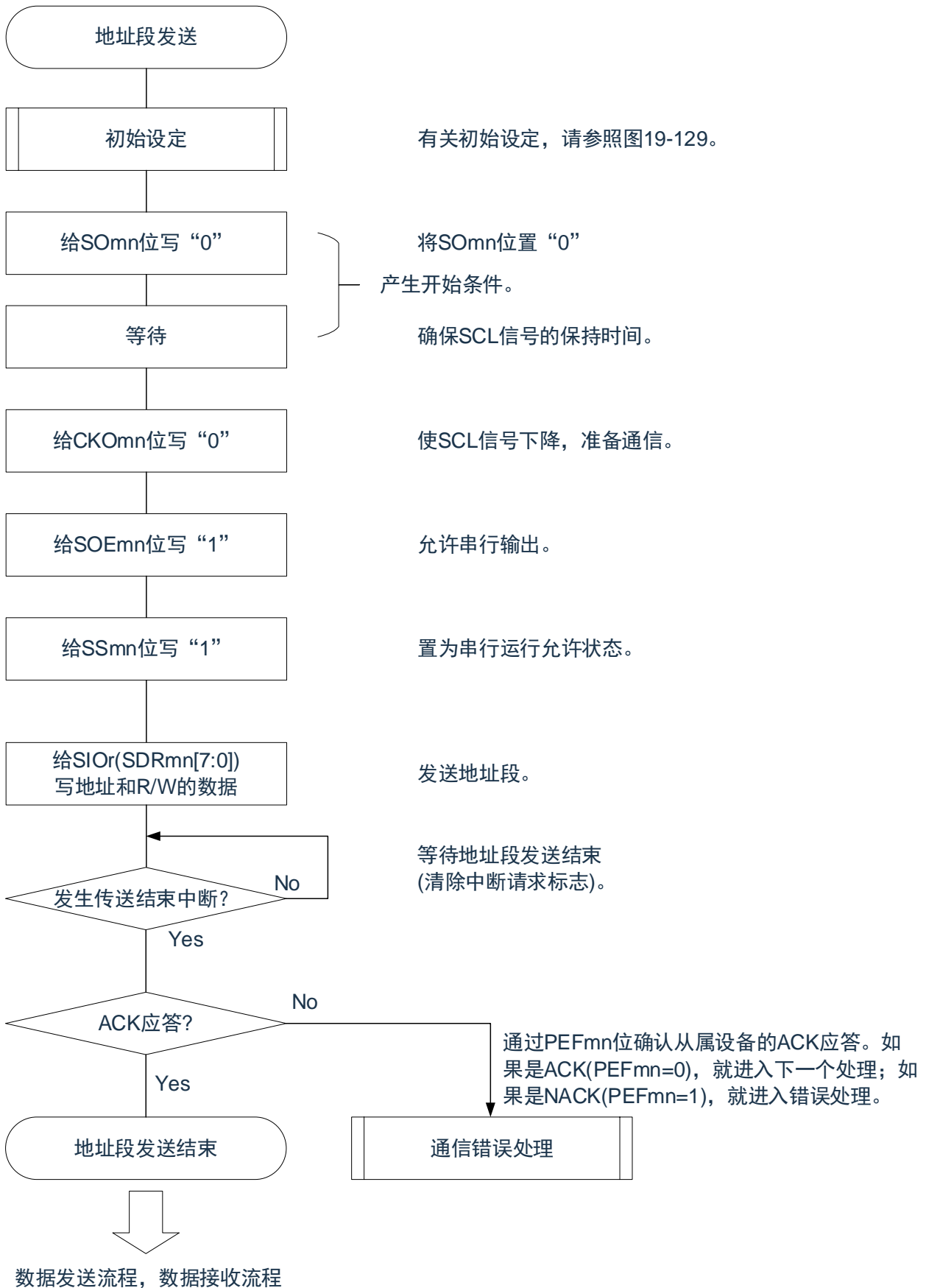
图19-131 地址段发送的流程图
