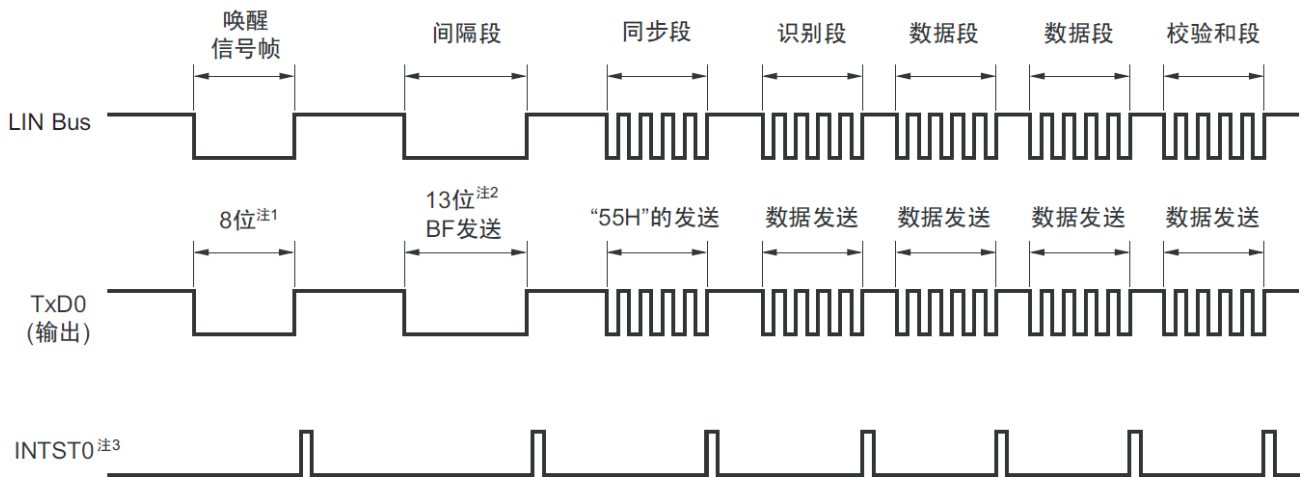
图19-123 LIN的发送操作
