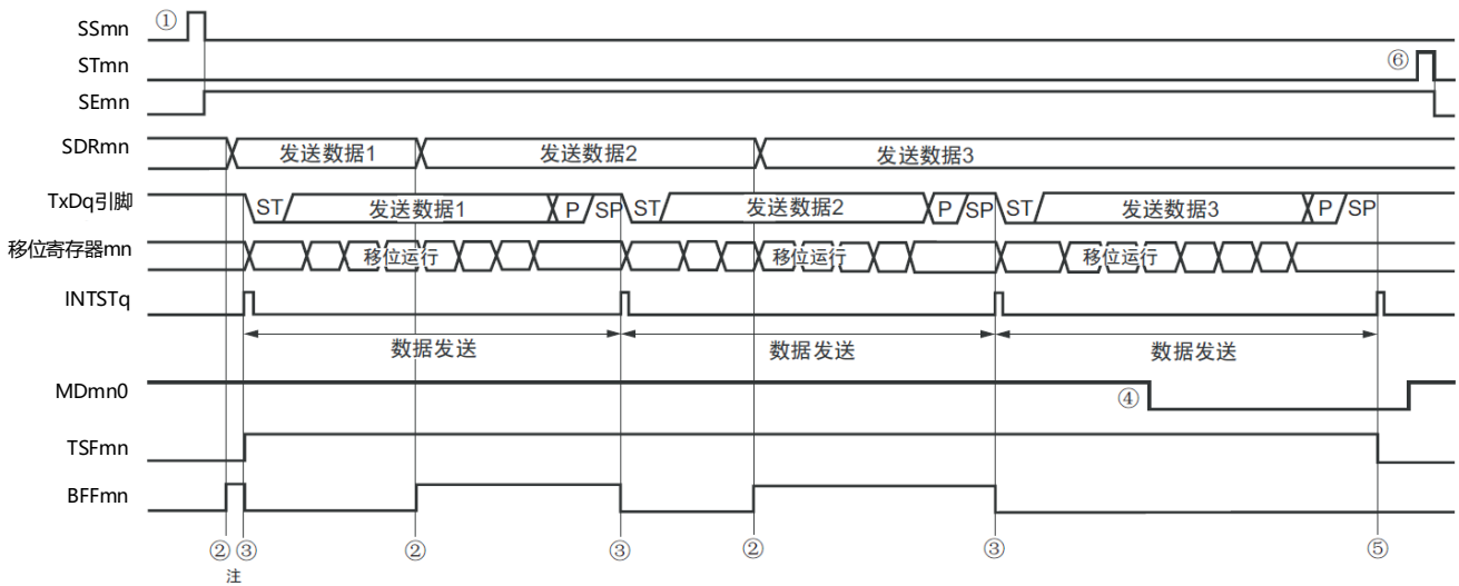
图19-107 UART发送(连续发送模式)的时序图
