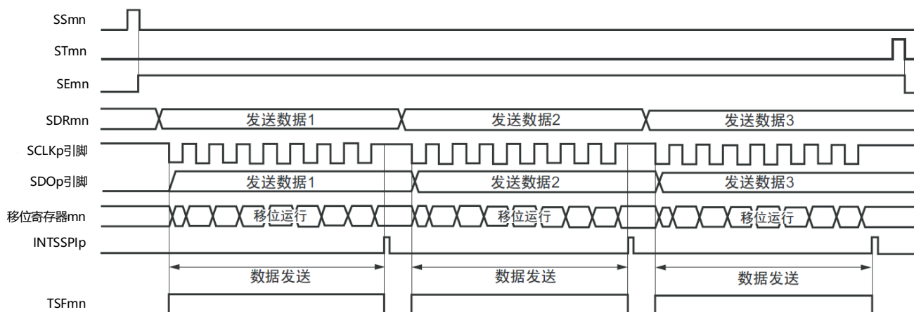
图19-29 主控发送(单次发送模式)的时序图(类型1: DAPmn=0、CKPmn=0)
