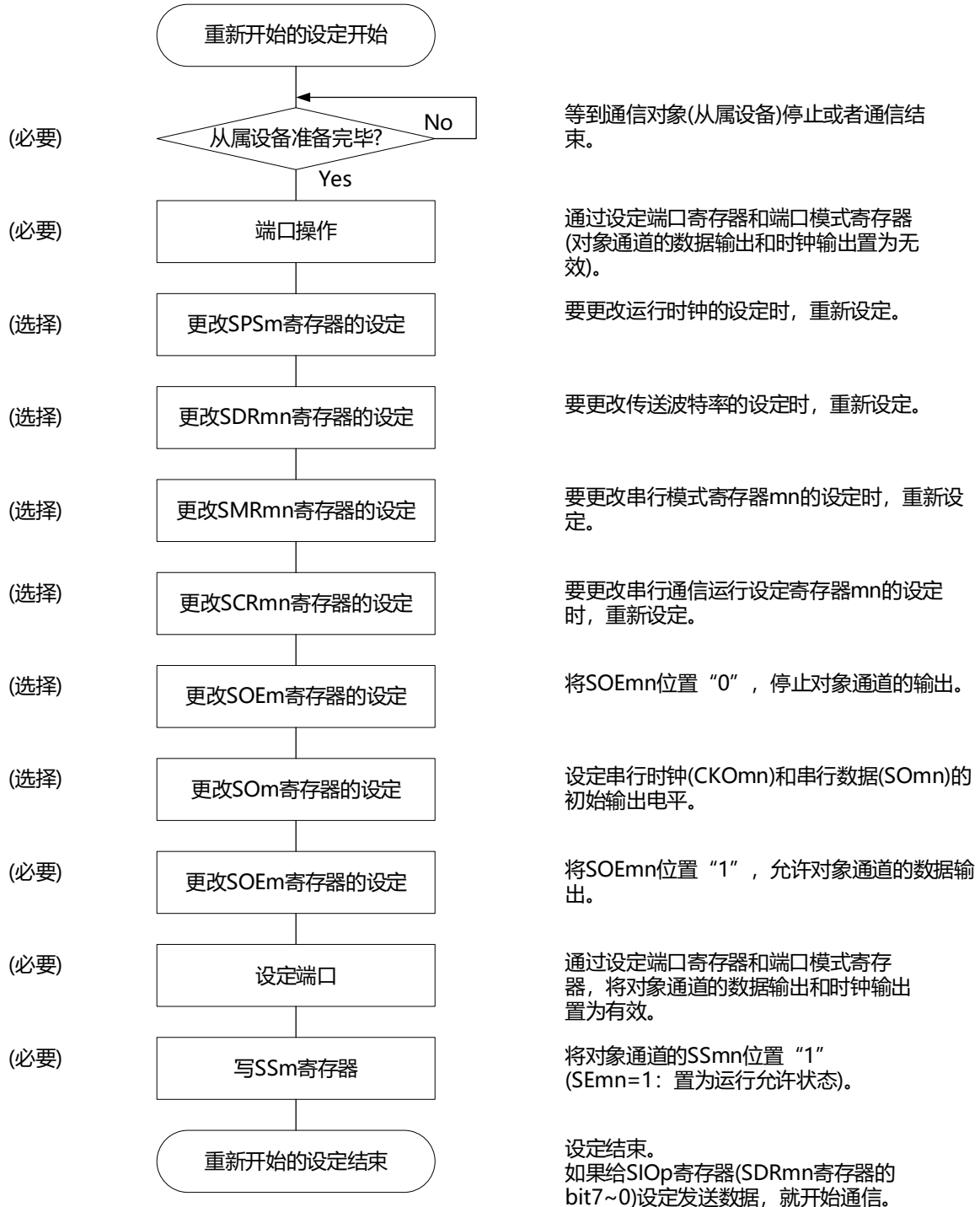
图19-28 重新开始主控发送的设置步骤
