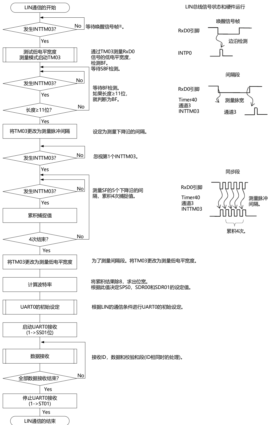
图19-126 LIN接收的流程图
