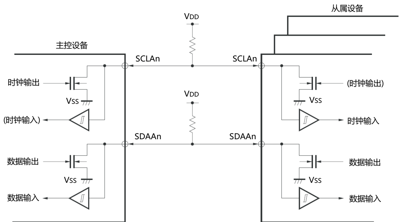
图20-13 引脚结构图
