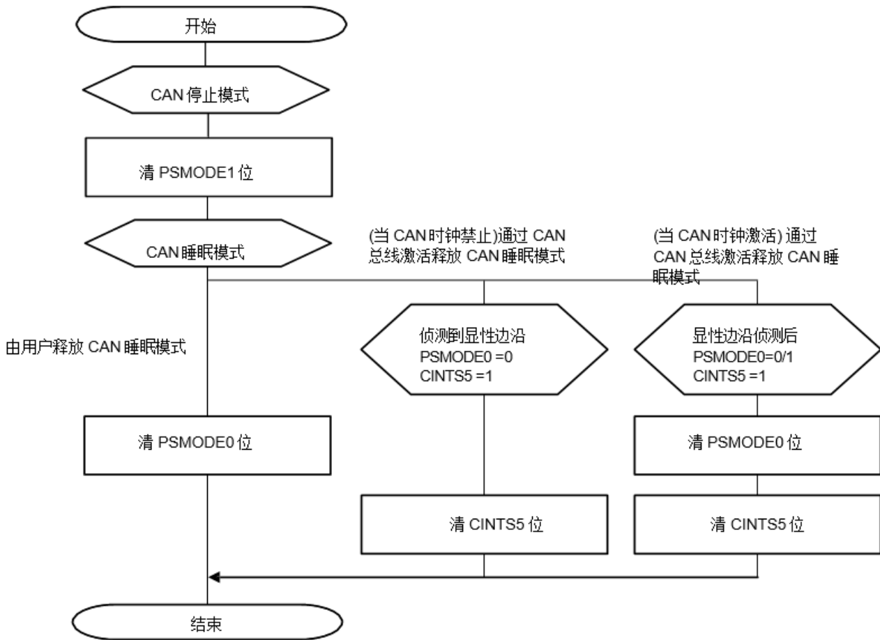
图21-81. 清CAN睡眠/停止模式
