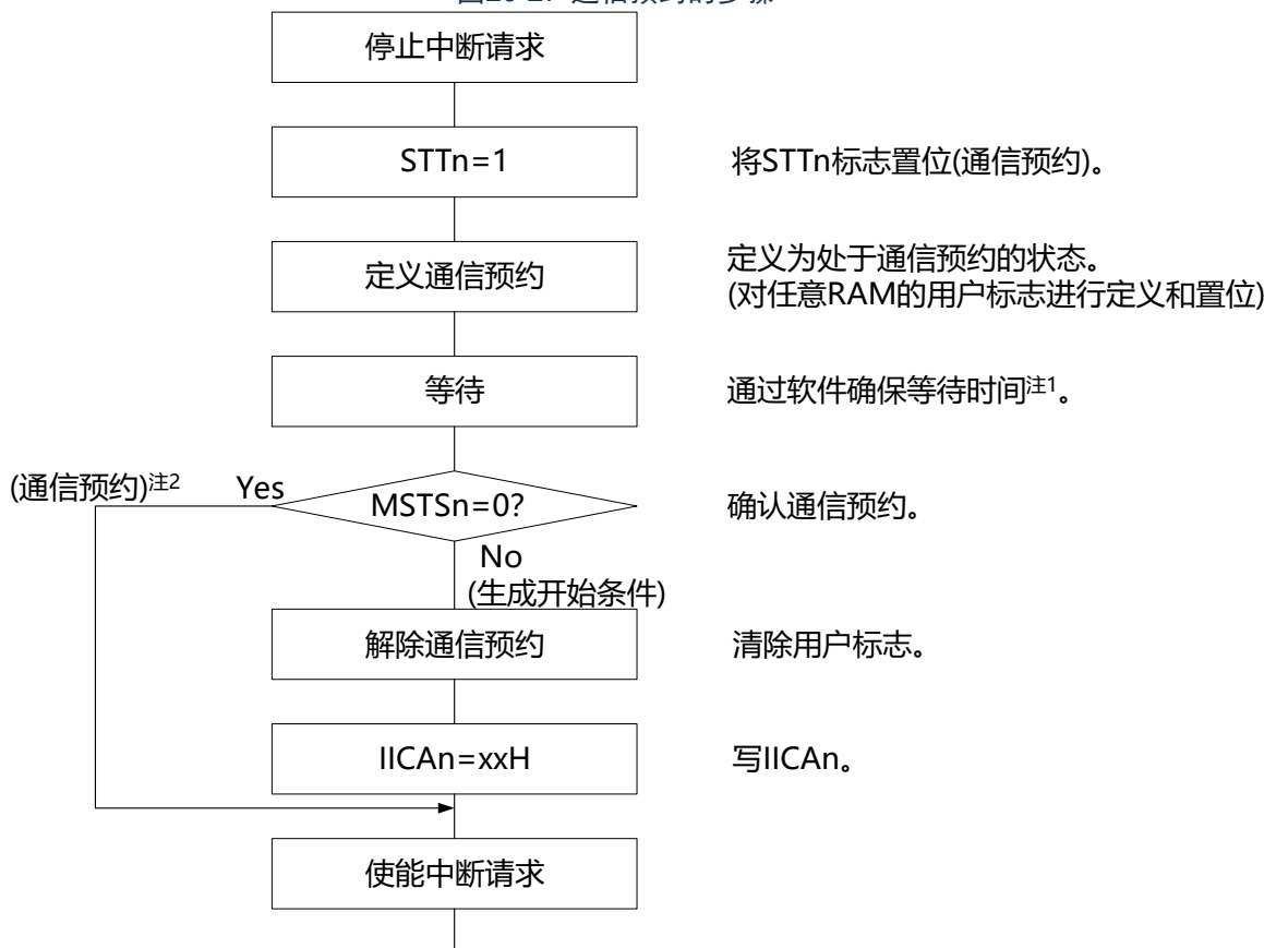
图20-27 通信预约的步骤
