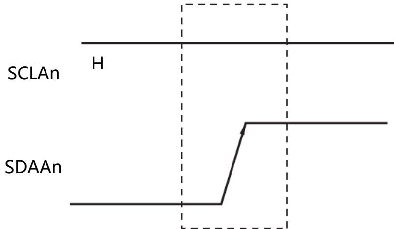
图20-19 停止条件
