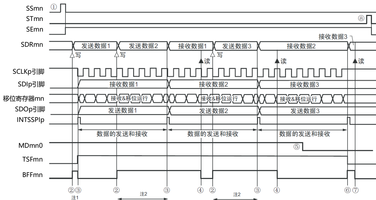
图19-47 主控发送和接收(连续发送和接收模式)的时序图(类型1: DAPmn=0、CKPmn=0)
