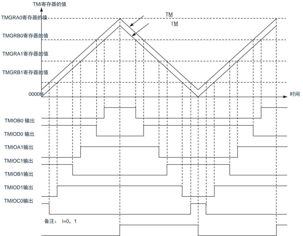
图10-59 互补PWM模式的输出模型
