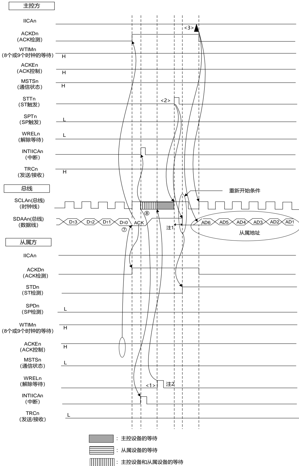
图20-32 主控设备→从属设备的通信例子
