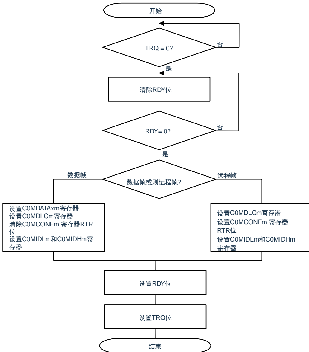
图21-68. 报文发送处理
