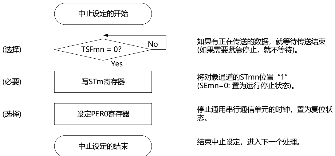
图19-111 UART接收的中止步骤
