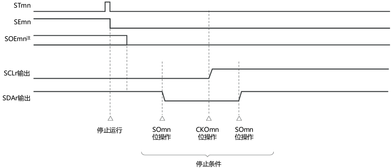
图19-138 产生停止条件的时序图
