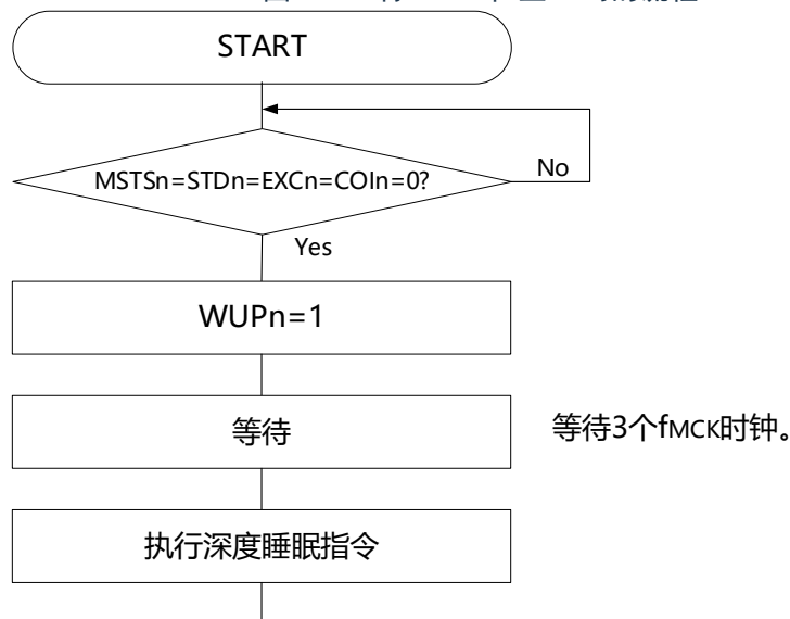
图20-22 将WUPn位置“1”时的流程
