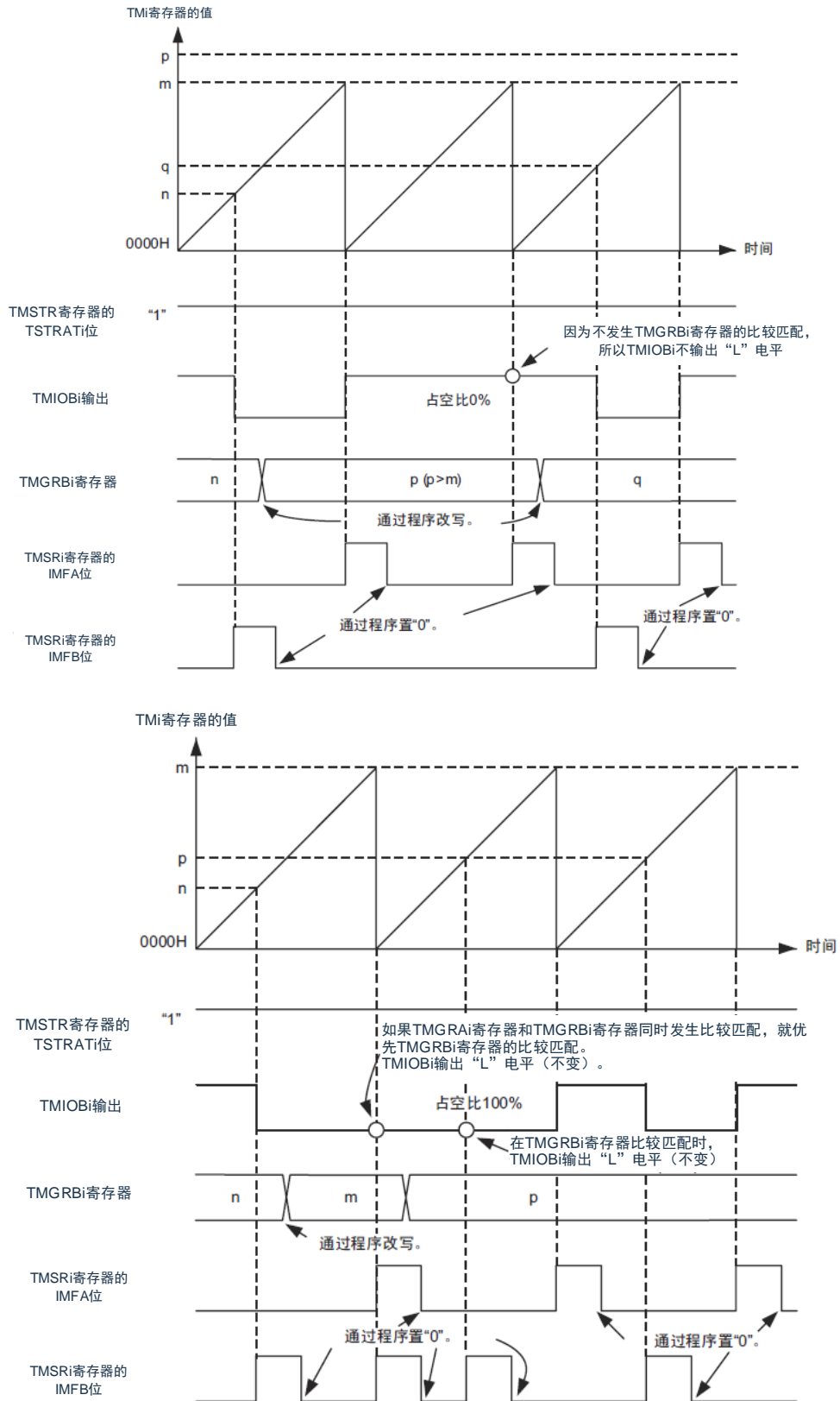
图 10-55 PWM功能的运行例子(占空比为0%和100%)
