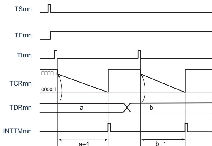
图6-57 作为延迟计数器的运行基本时序例子
