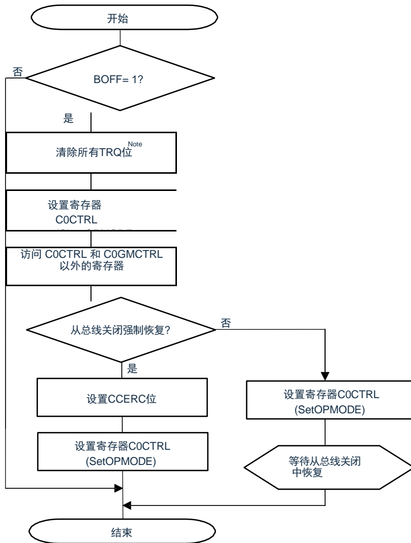
图21-82. 总线关闭恢复 (正常操作模式伴ABT)
