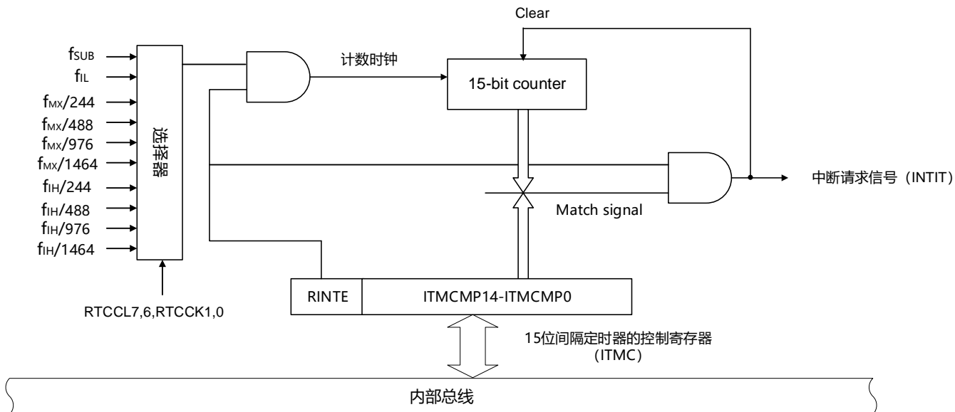
图12-1 15位间隔定时器的框图
