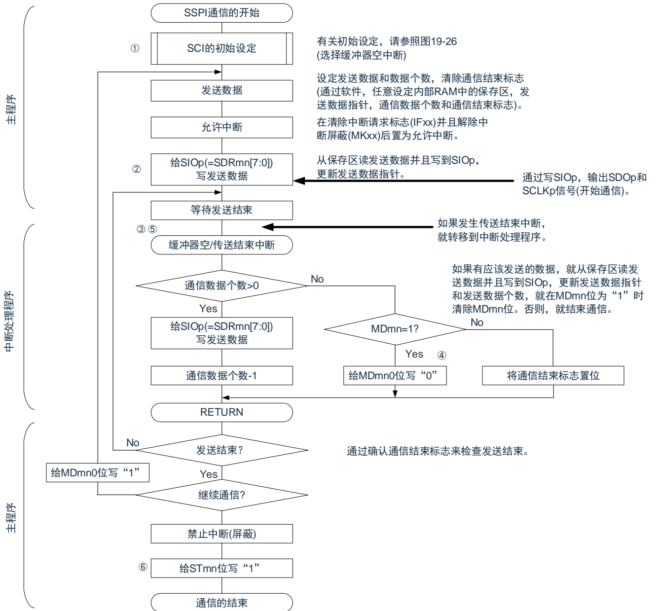
图19-32 主控发送(连续发送模式)的流程图
