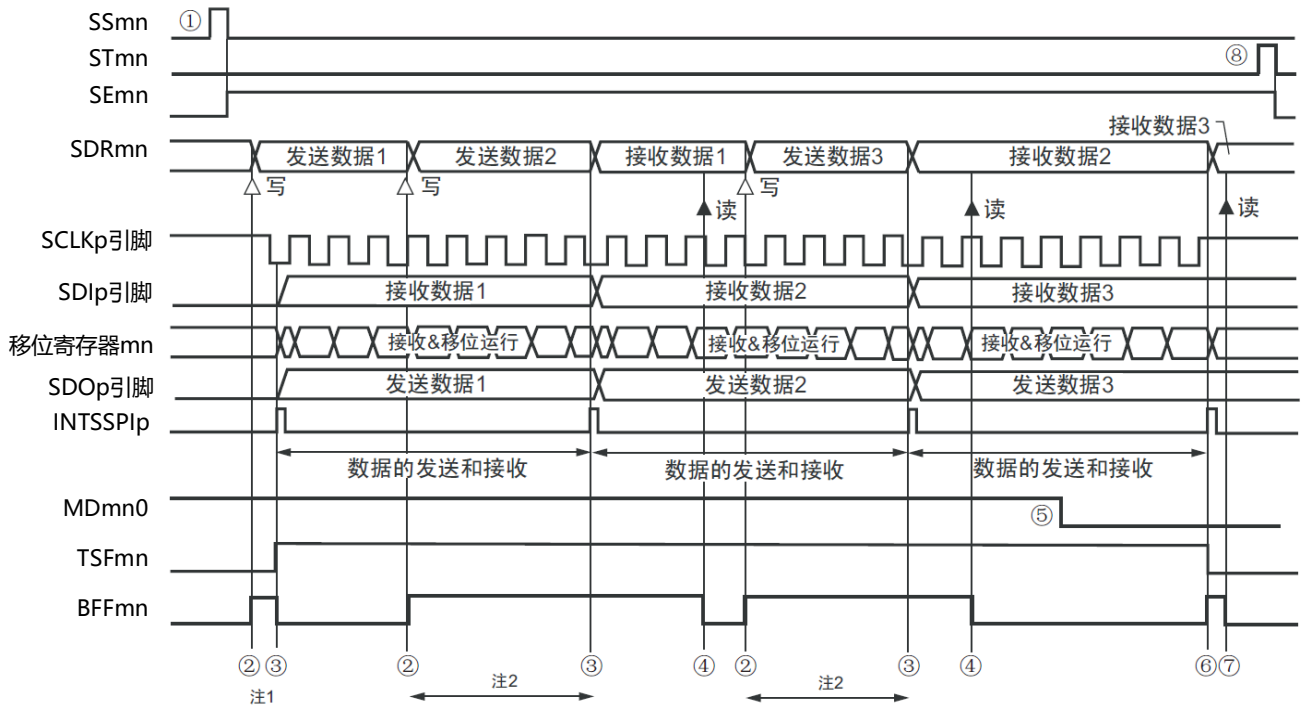
图19-69 从属发送和接收(连续发送和接收模式)的时序图(类型1: DAPmn=0、CKPmn=0)
