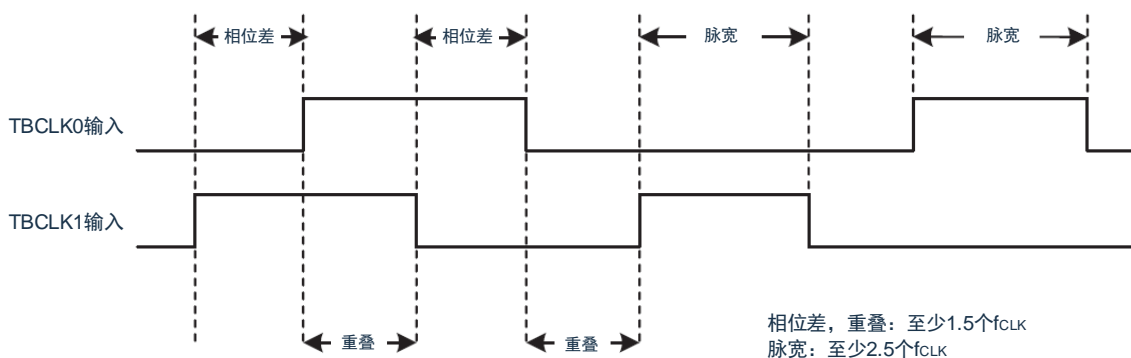
图8-32 相位计数模式中的相位差、重叠和脉宽
