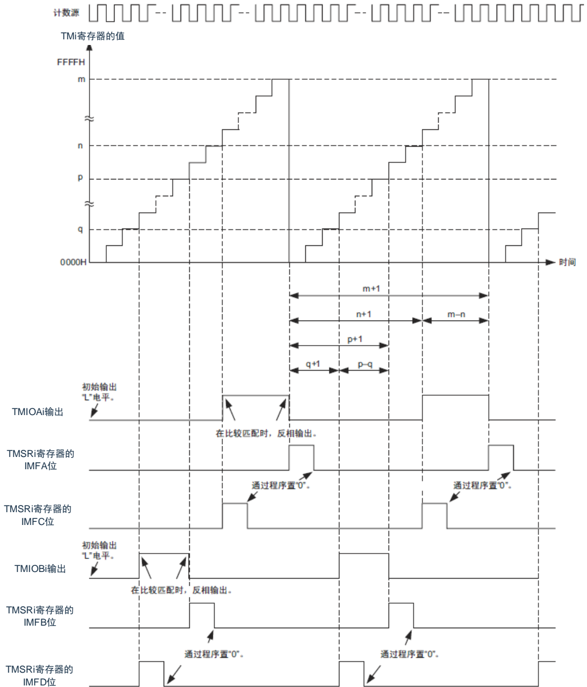
图10-52 将TMGRCi和TMGRDi分别用于TMIOAi引脚和TMIOBi引脚的输出控制时的运行例子
