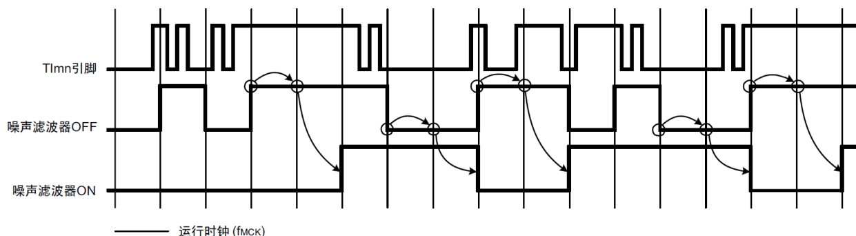
图6-40 TImn输入引脚在噪声滤波器ON或者OFF情况下的采样波形
