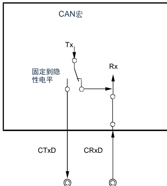
图21-59. CAN模式仅接收模式下的终端连接
