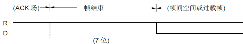
图21-12. 帧结束(EOF)
