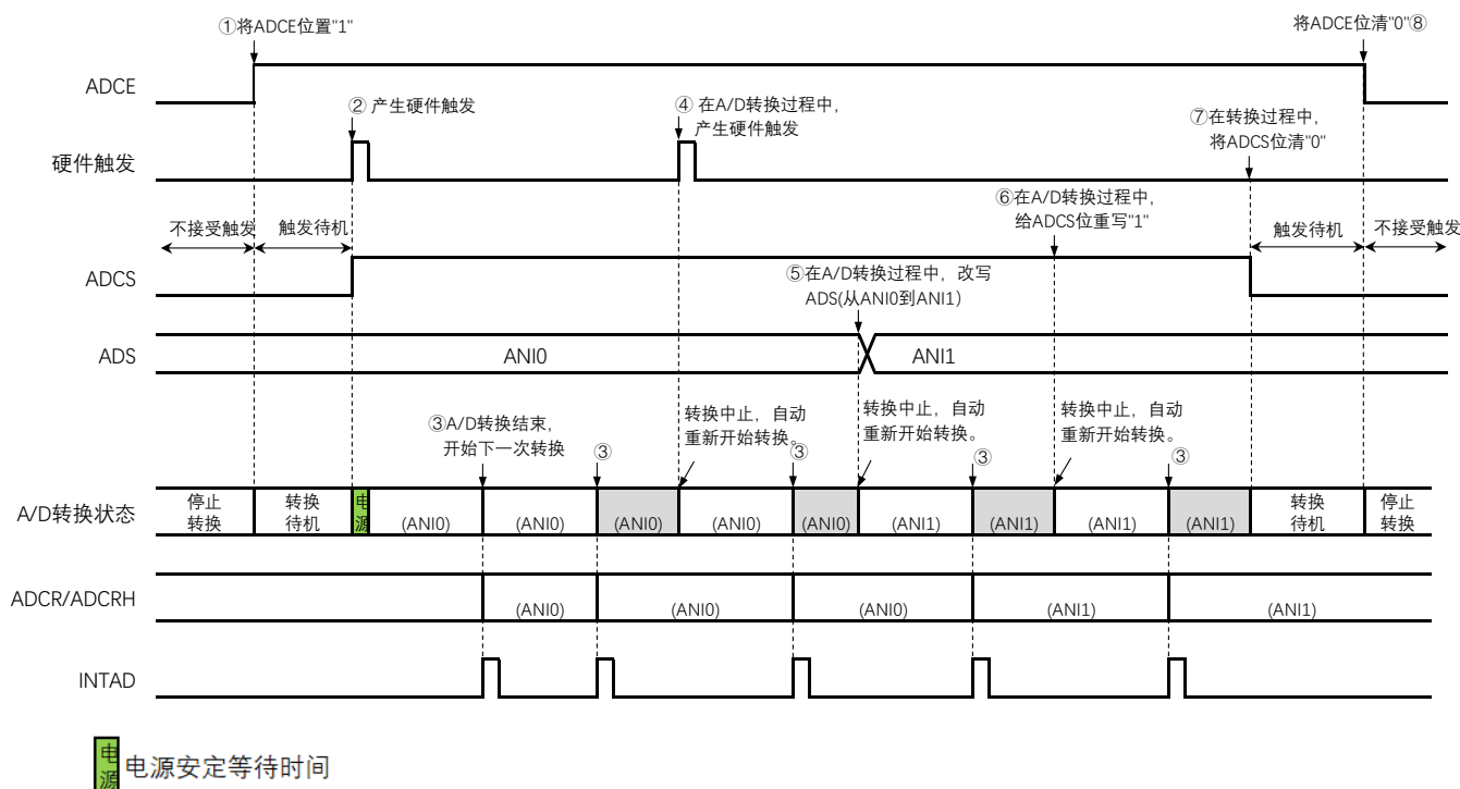
图15-25 硬件触发等待模式(选择模式、连续转换模式)的运行时序例子
