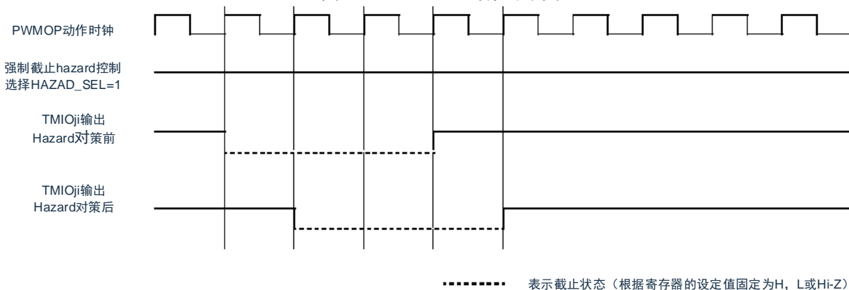
图10-89 Hazard对策时序图
