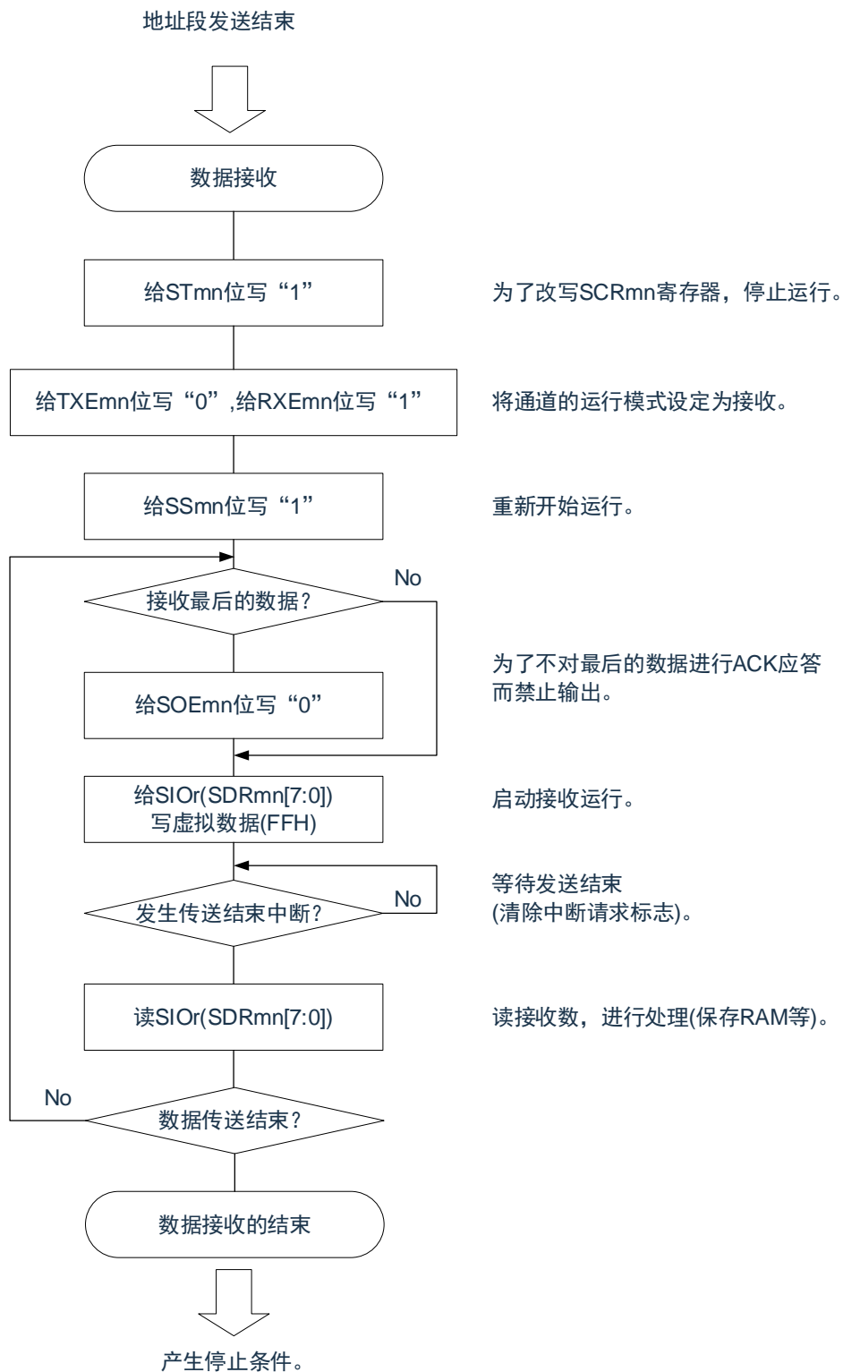
图19-137 数据接收的流程图
