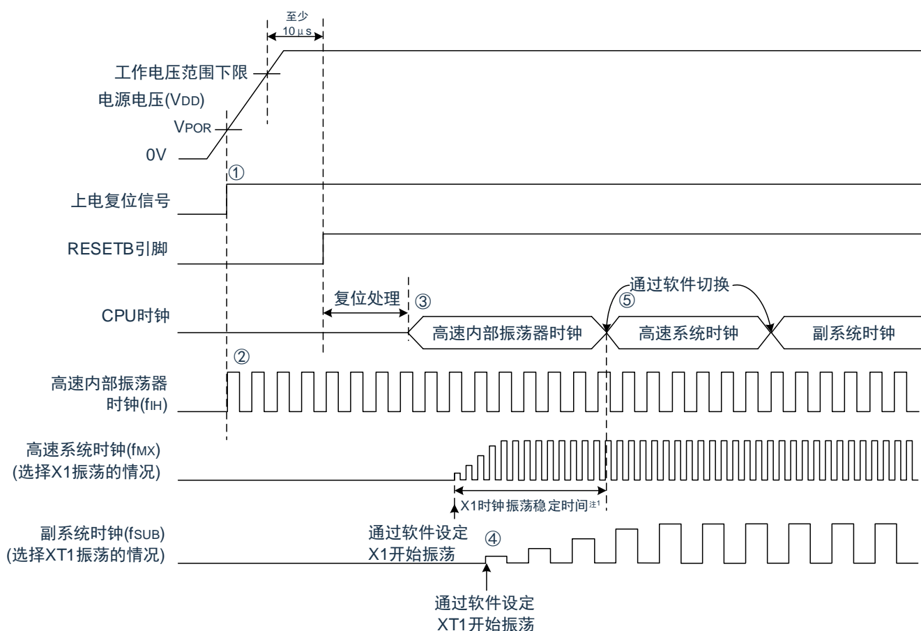
图4-15 接通电源时的时钟发生电路的运行
