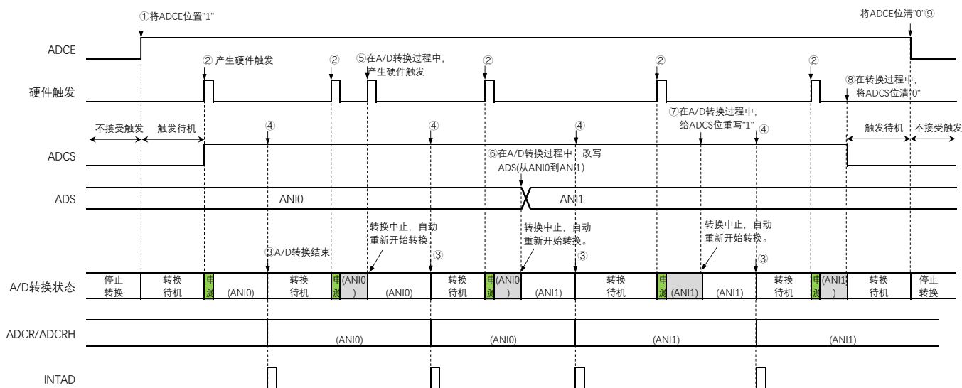
图15-26 硬件触发等待模式(选择模式、单次转换模式)的运行时序例子
