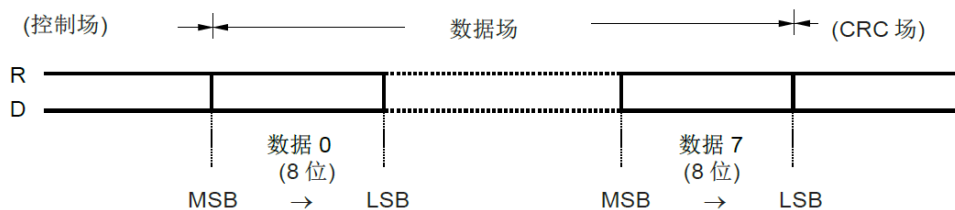
图21-9. 数据场
