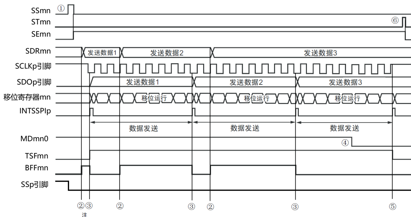
图19-84 从属发送(连续发送模式)的时序图(类型1: DAPmn=0、CKPmn=0)
