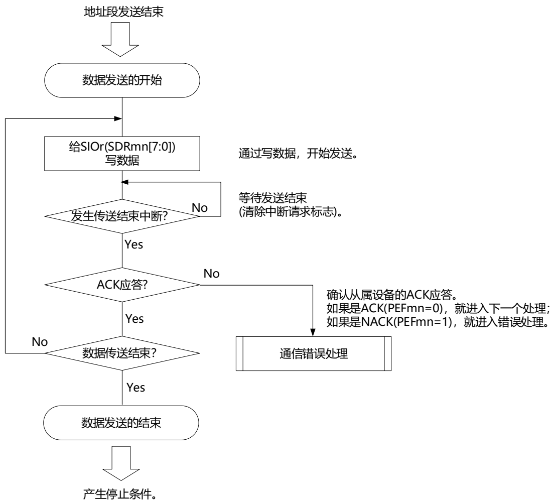
图19-134 数据发送的流程图
