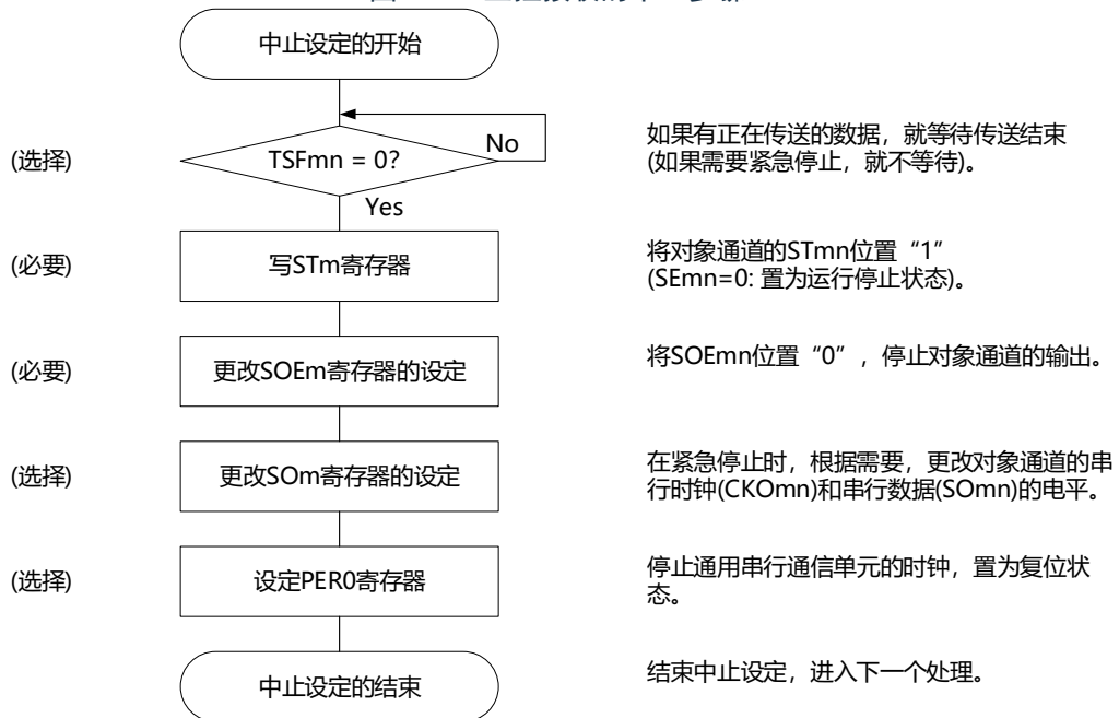
图19-35 主控接收的中止步骤
