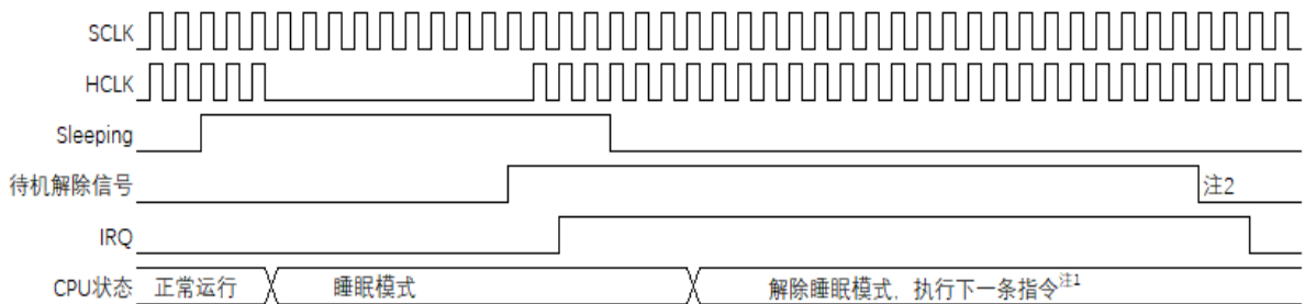
图27-1通过中断请求解除睡眠模式
