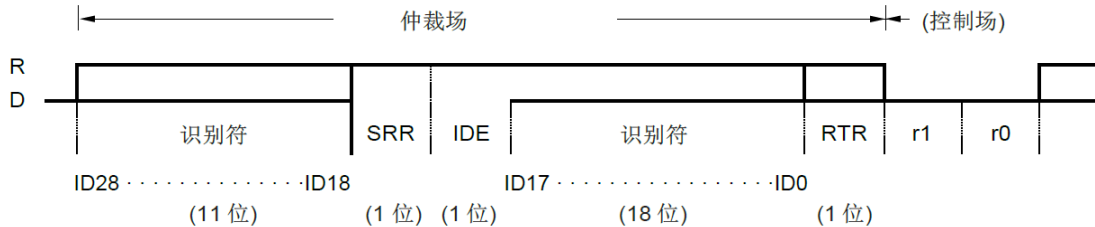
图21-7. 仲裁场 (在扩展帧模式)
