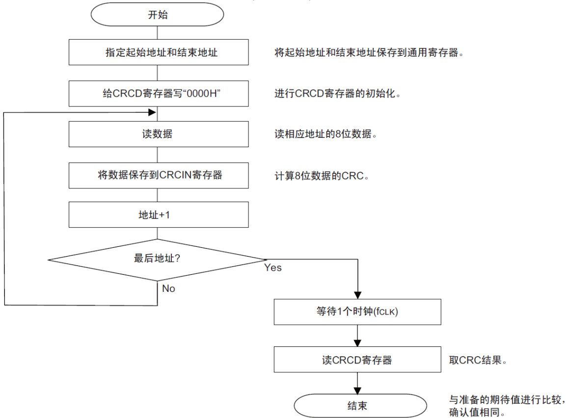
图31-6 CRC运算功能(通用CRC)的流程图
