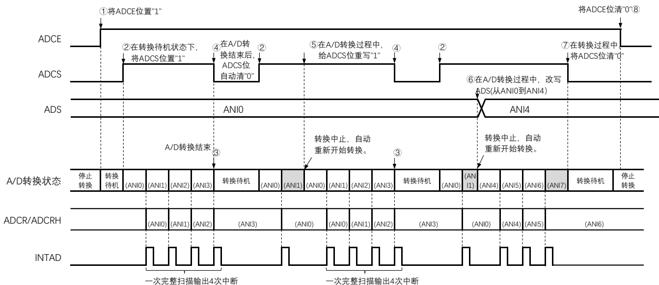
图15-20 软件触发模式(扫描模式、单次转换模式)的运行时序例子
