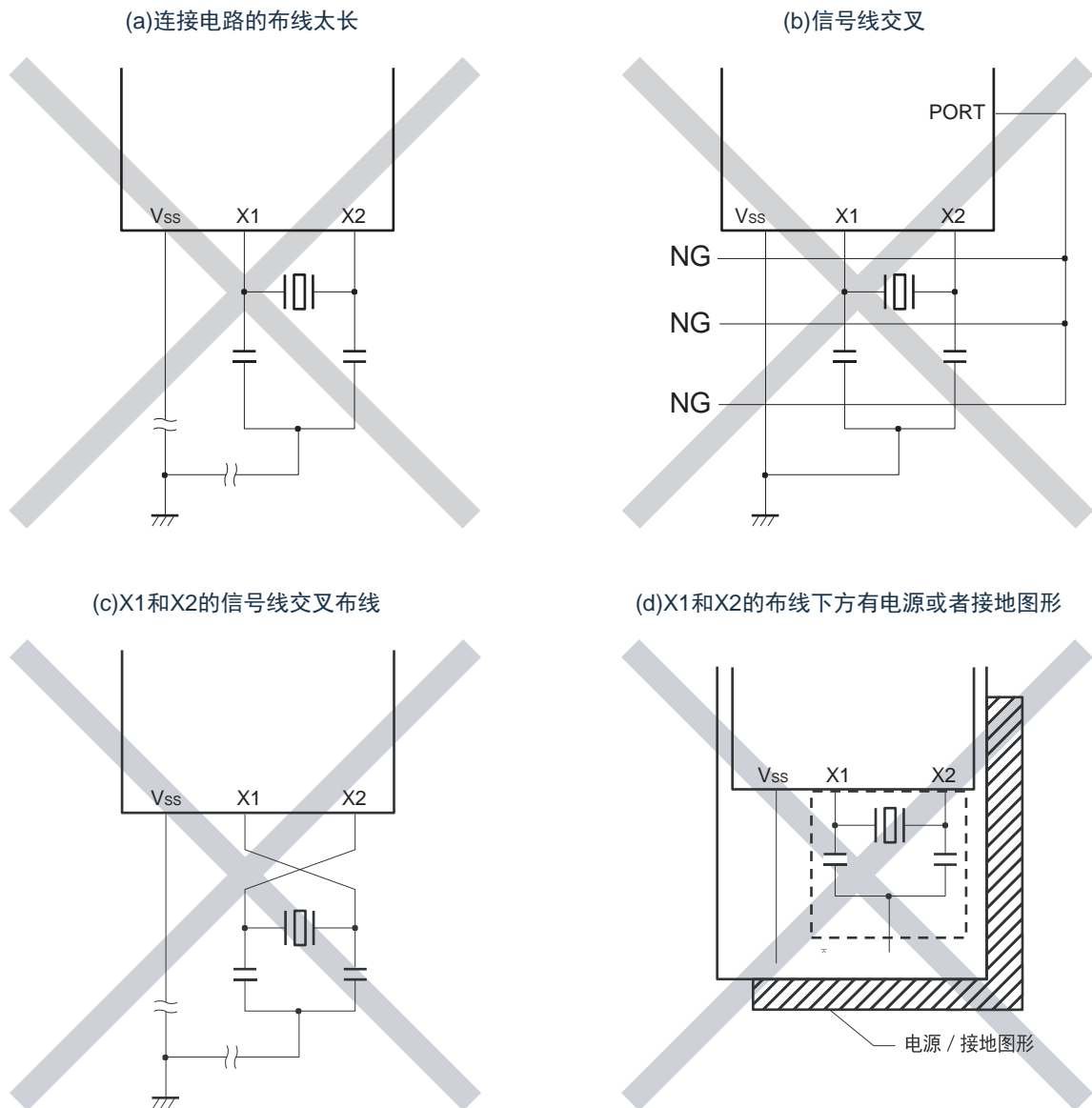
图4-14 不正确的谐振器连接例子(1/2)
