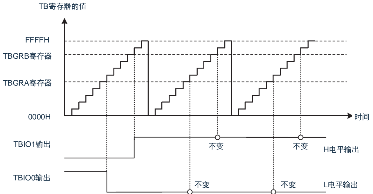
图8-21 “L”电平输出和“H”电平输出的运行例子
