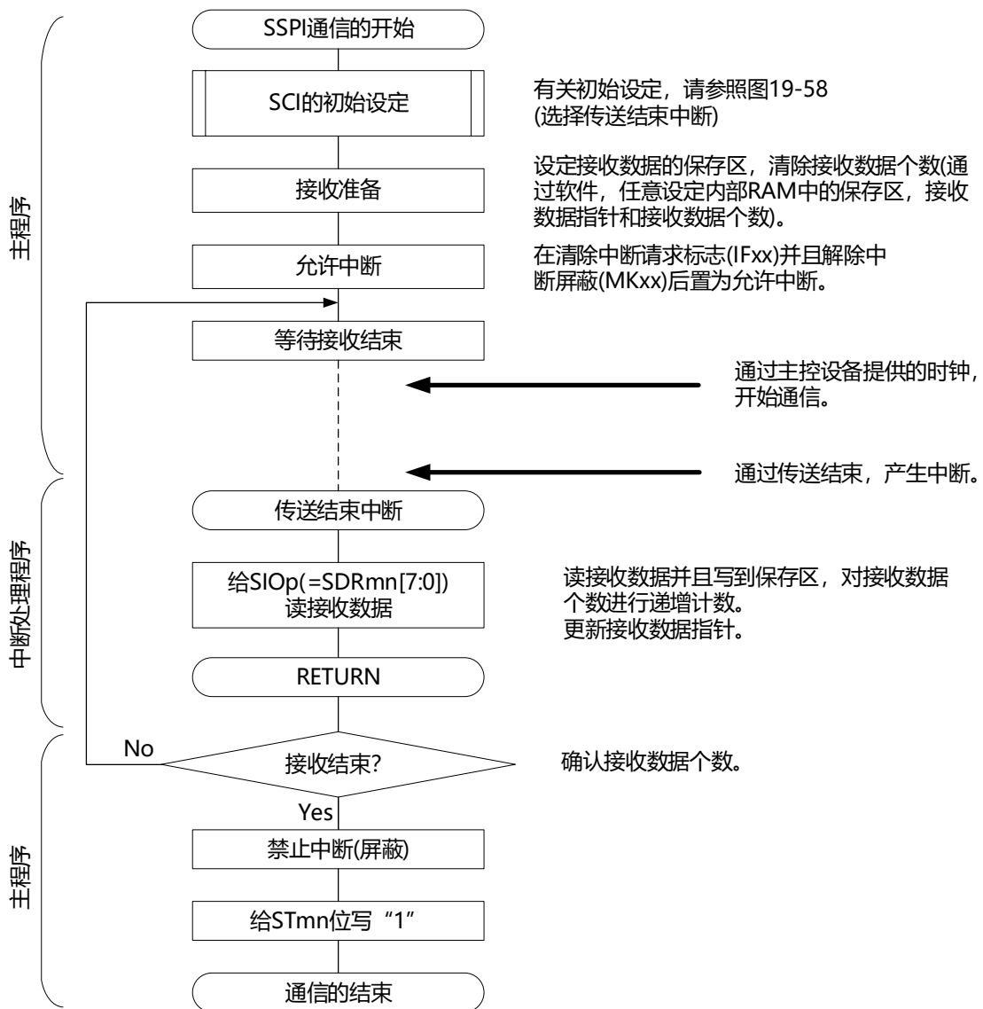
图19-91 从属接收(单次接收模式)的流程图
