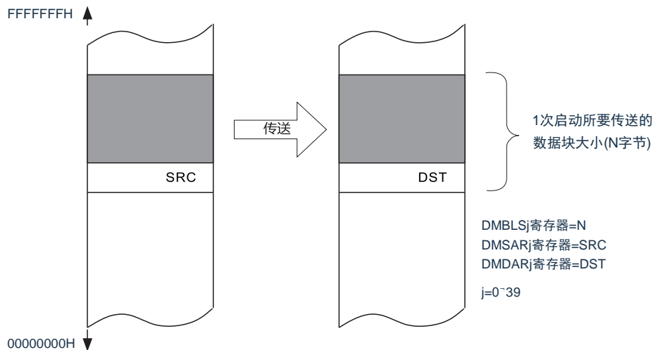
图23-15 正常模式的数据传送
