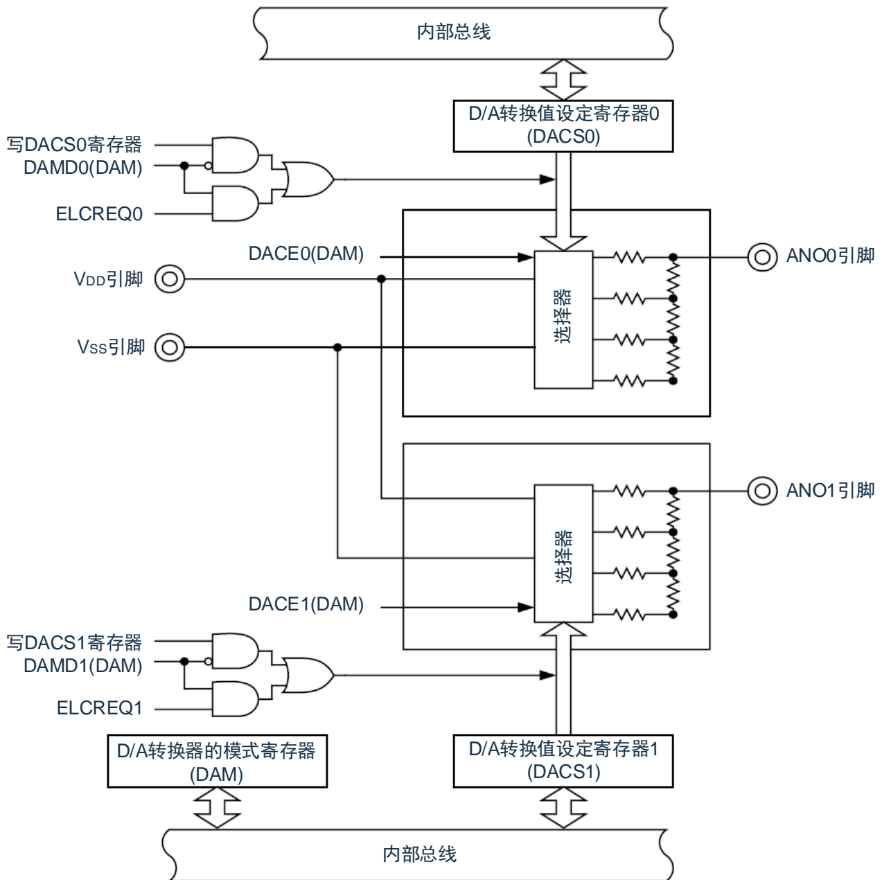
图16-1 D/A转换器的框图
