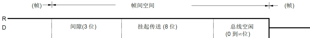
图21-14. 帧间空间(错误主动节点)
