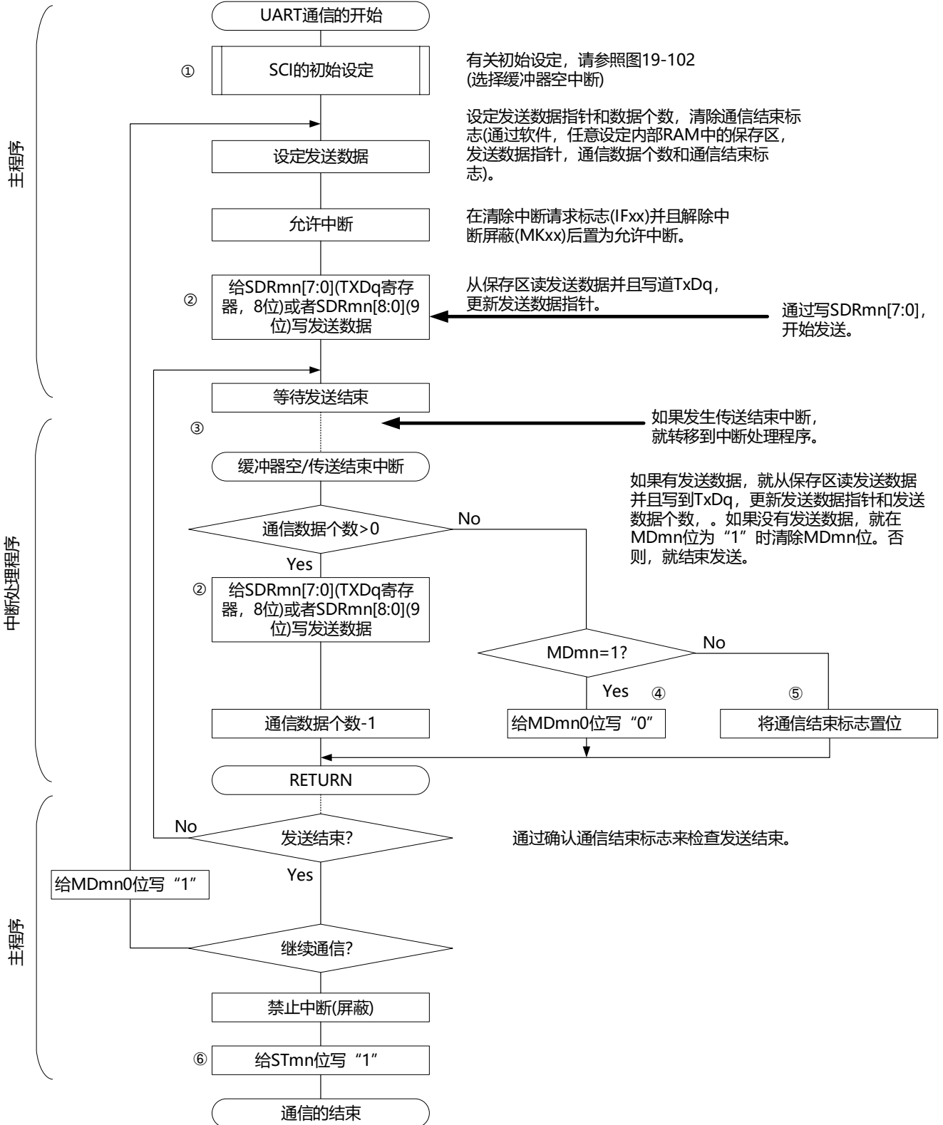
图19-108 UART发送(连续发送模式)的流程图
