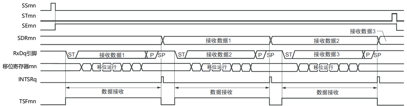
图19-113 UART接收的时序图
