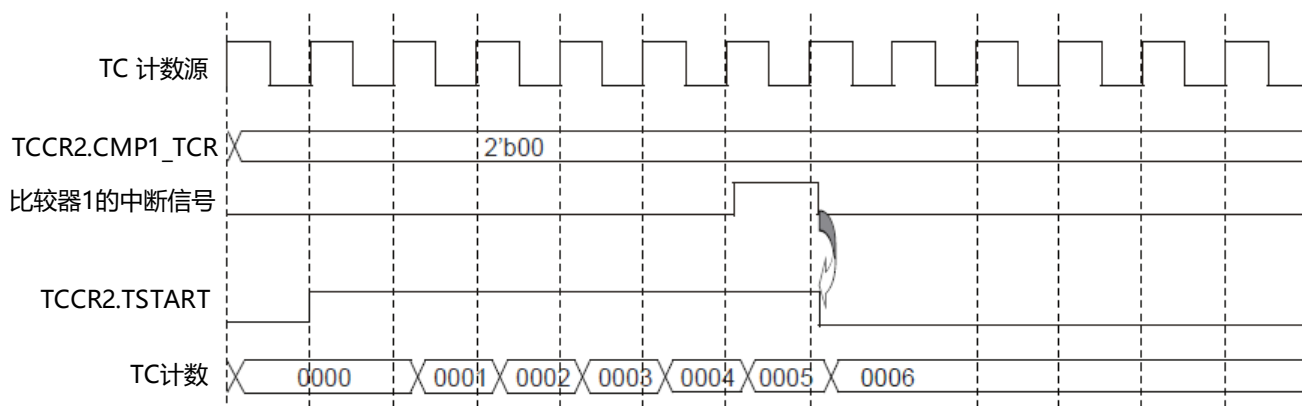
图9-11 选择比较器1触发Timer C停止的例子
