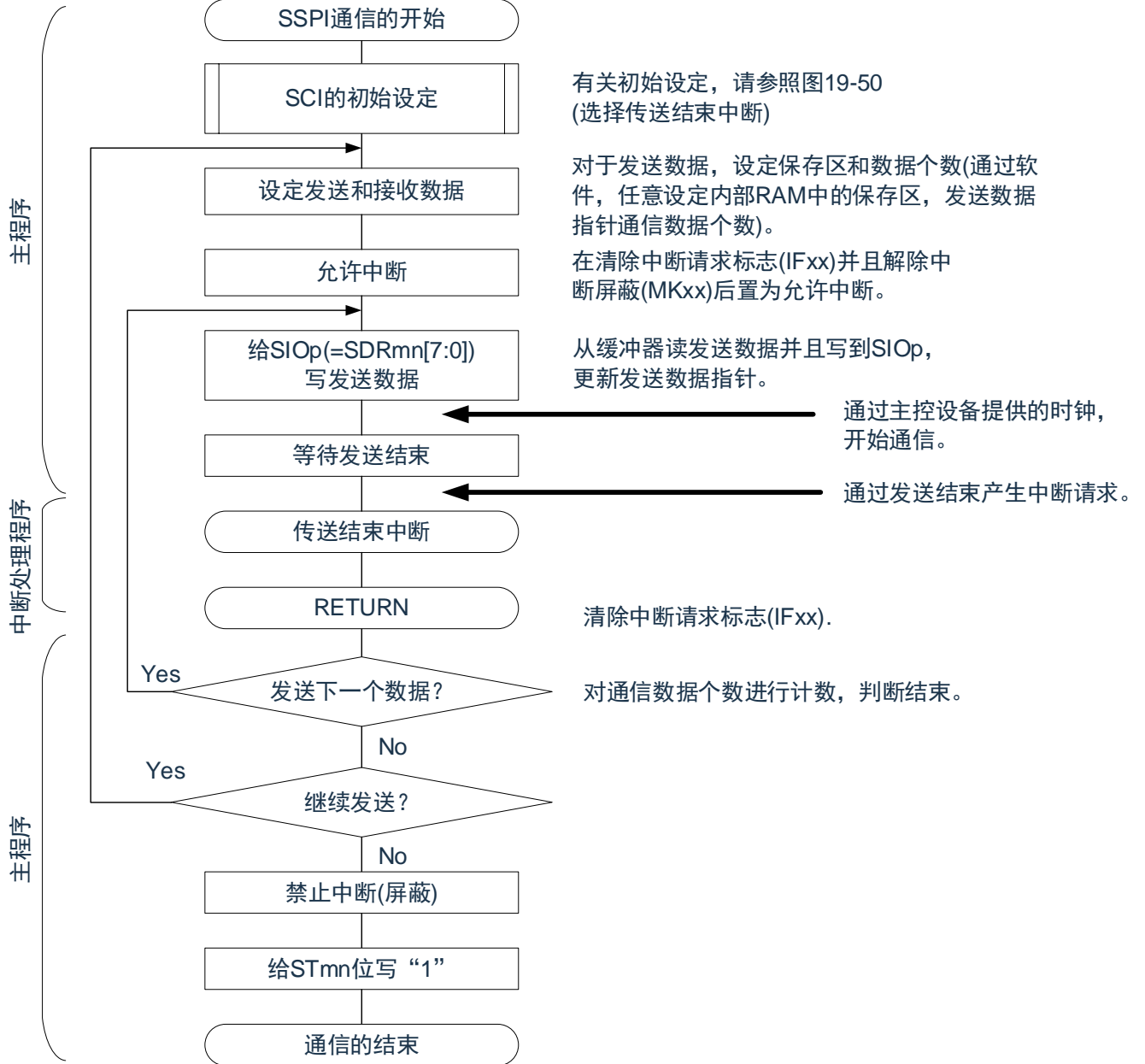
图19-54 从属发送(单次发送模式)的流程图
