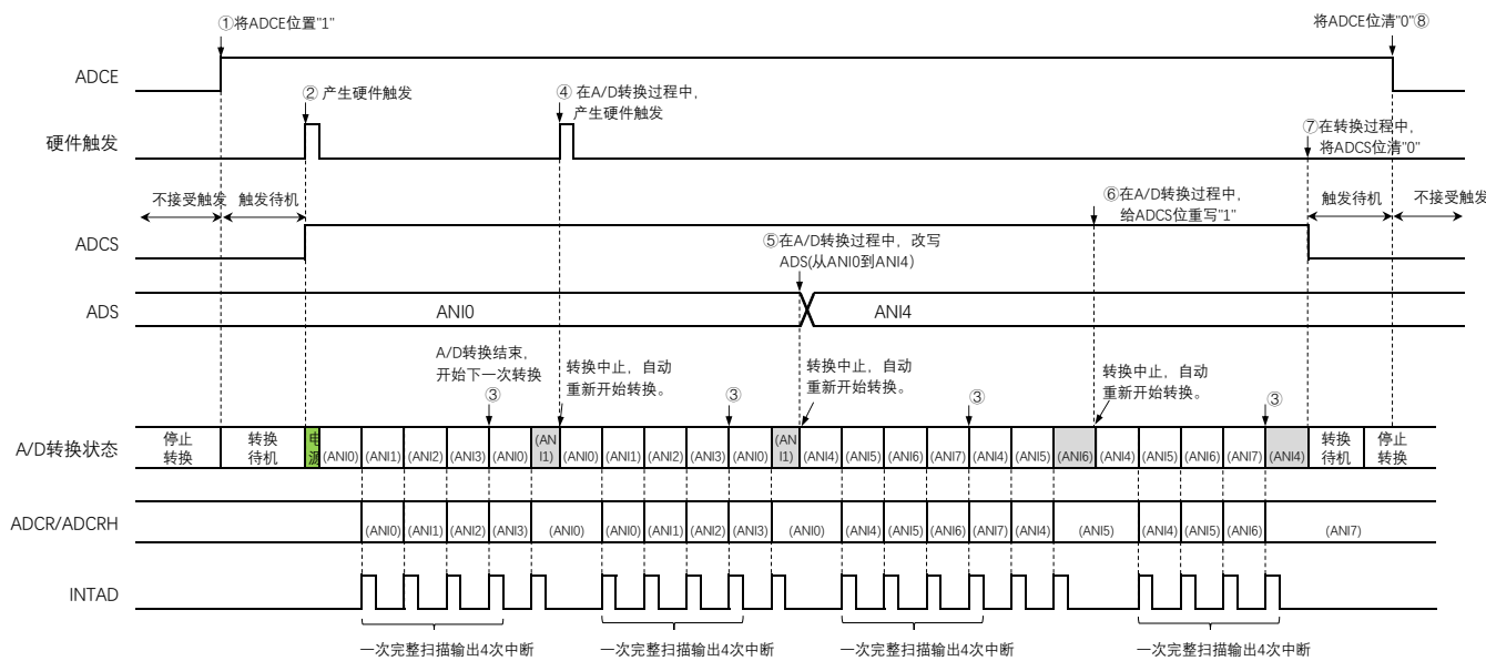
图15-27 硬件触发等待模式(扫描模式、连续转换模式)的运行时序例子
