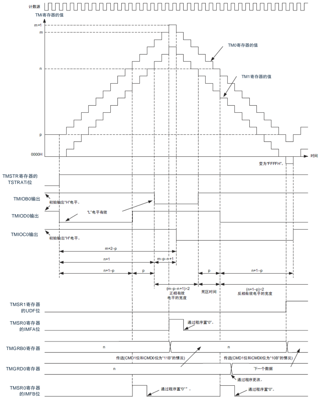
图10-60 互补PWM模式的运行例子
