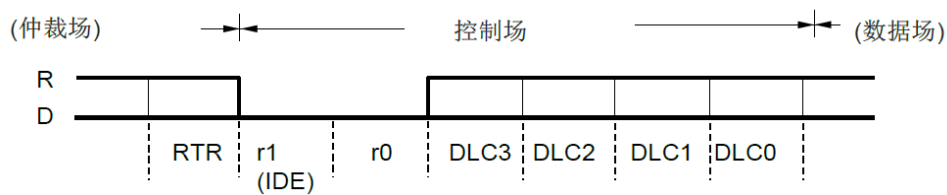
图21-8. 控制场
