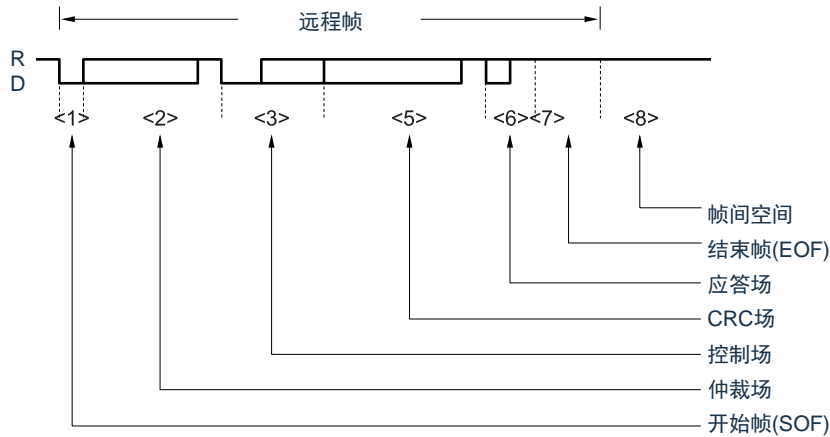
图21-4. 远程帧
