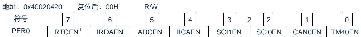
图6-5 外围允许寄存器0(PER0)的表格
