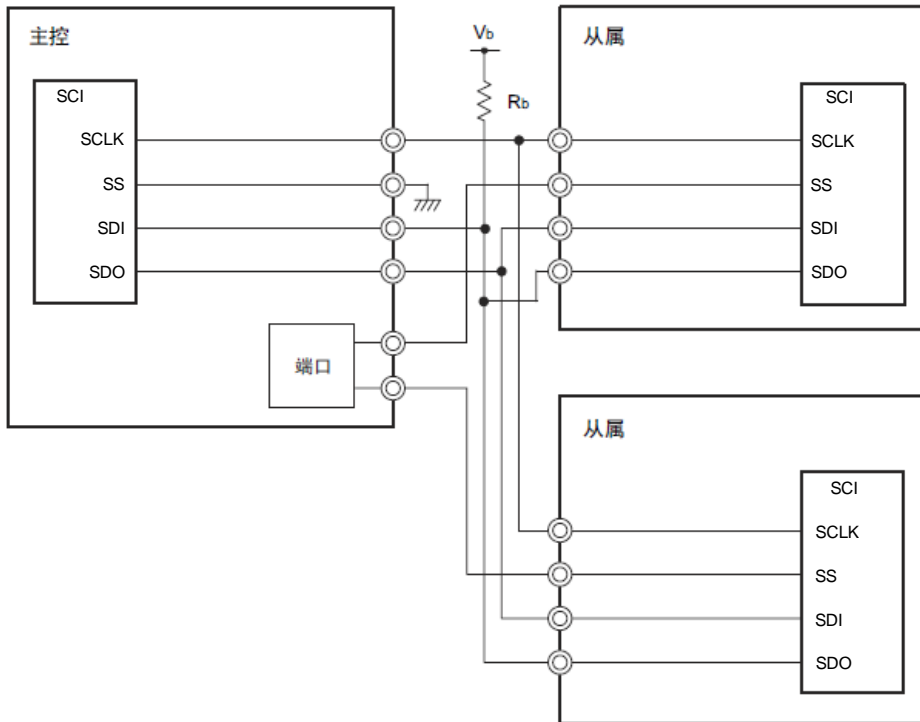
图19-76 从属选择输入功能的结构例子
