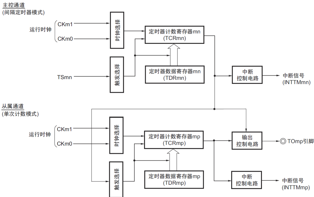
图6-66 作为PWM功能运行的框图
