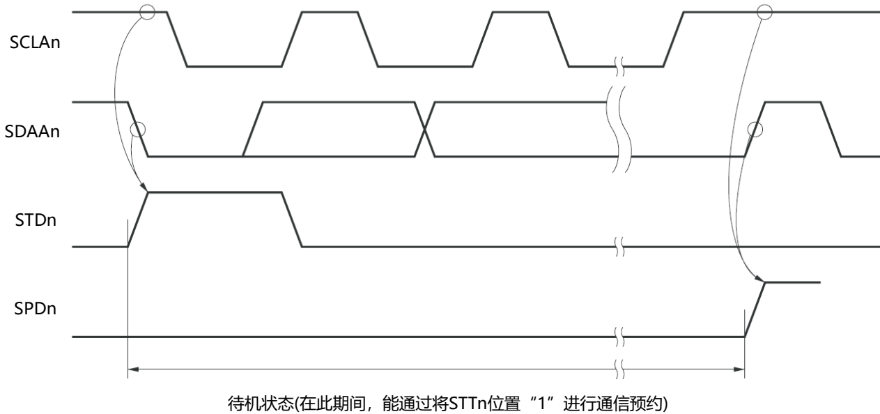
图20-26 通信预约的接受时序
