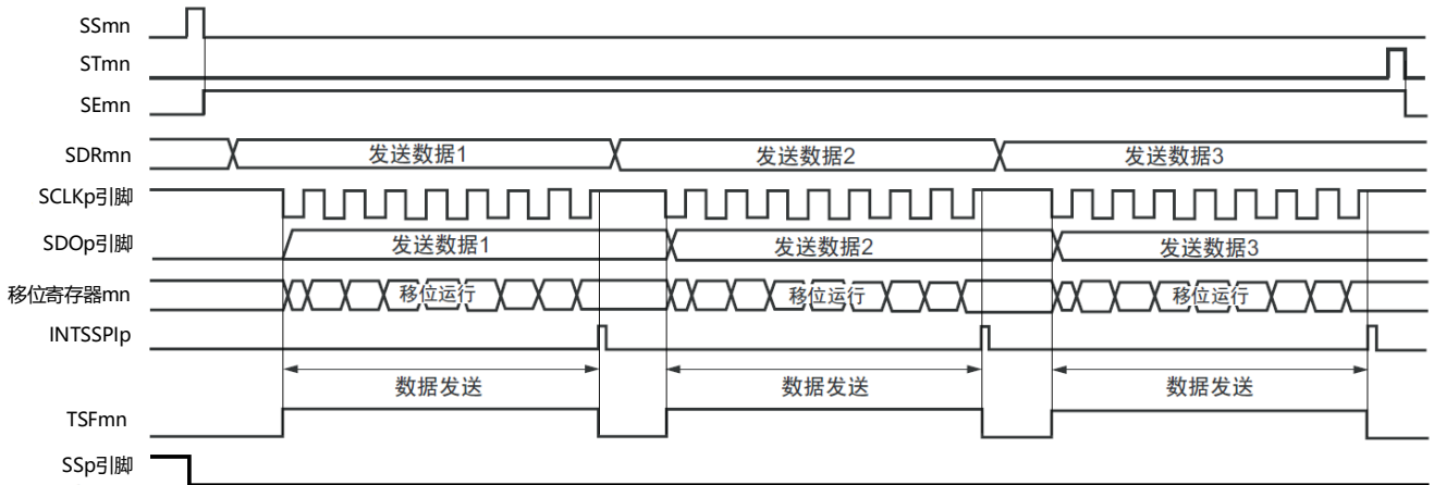
图19-82 从属发送(单次发送模式)的时序图(类型1: DAPmn=0、CKPmn=0)
