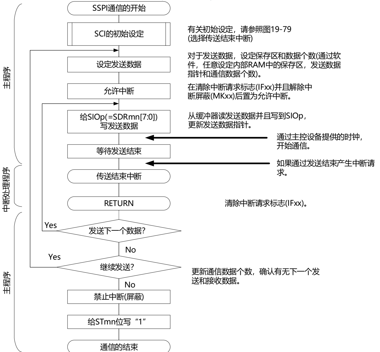
图19-83 从属发送(单次发送模式)的流程图
