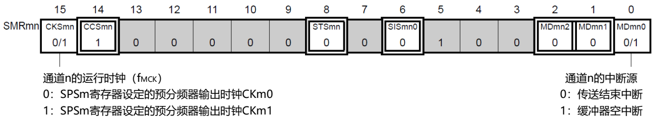
图19-63 3线串行I/O(SSPI00、SSPI01、SSPI10、SSPI11、SSPI20、SSPI21) 从属发送和接收时的寄存器设置内容例子
