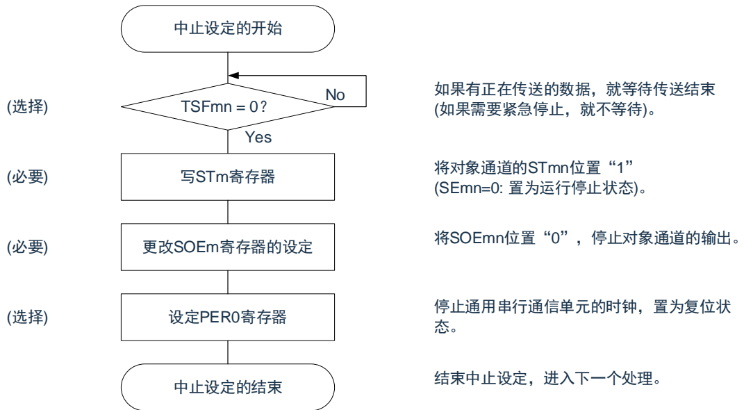
图19-59 从属接收的中止步骤
