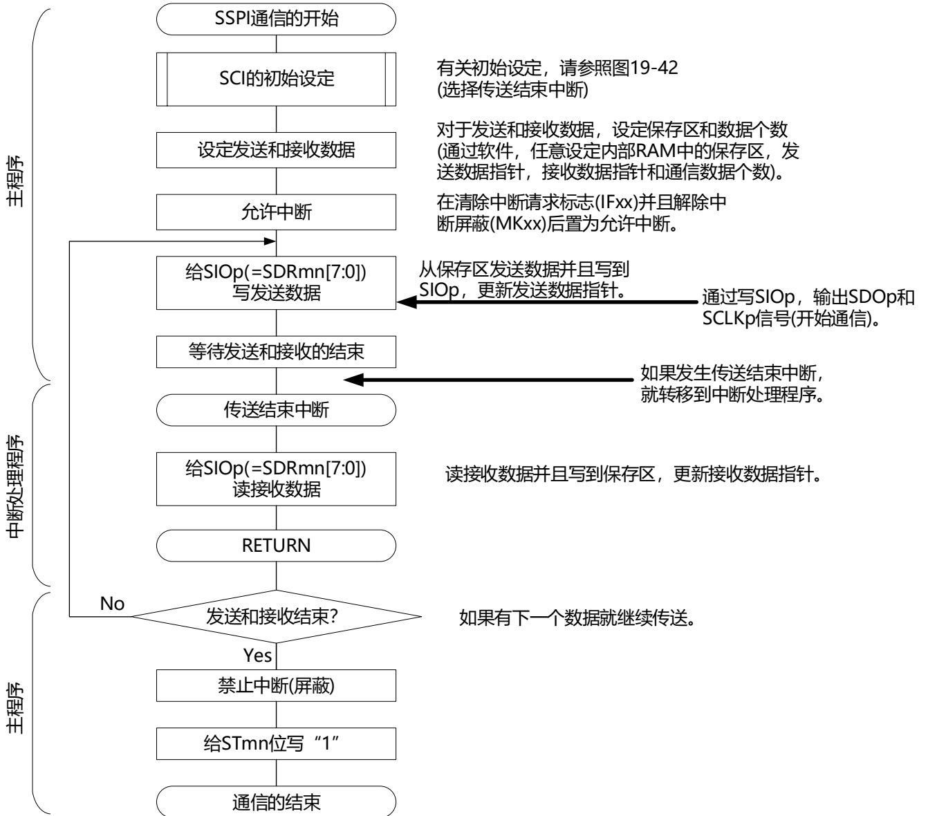
图19-46 主控发送和接收(单次发送和接收模式)的流程图
