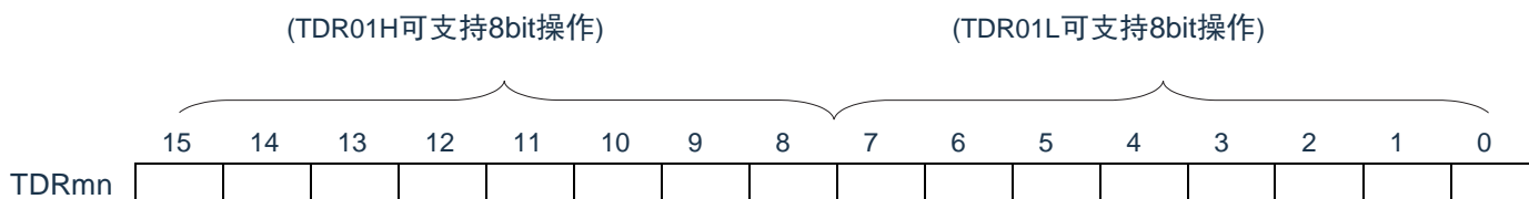
图6-4 定时器数据寄存器mn(TDRmn)(n=1、3)的表格
