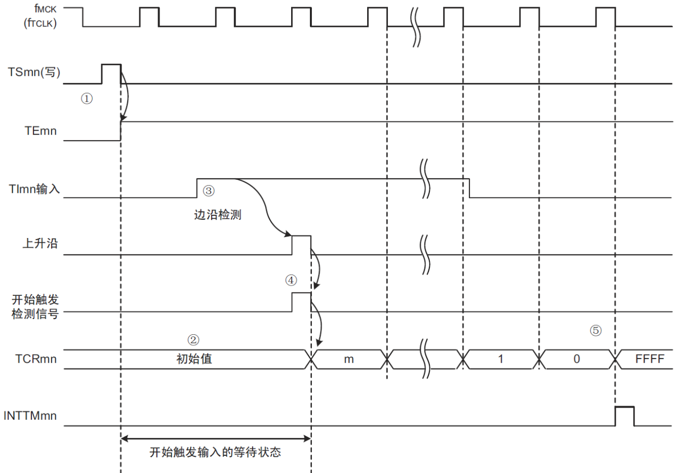
图6-29 运行时序(单次计数模式)
