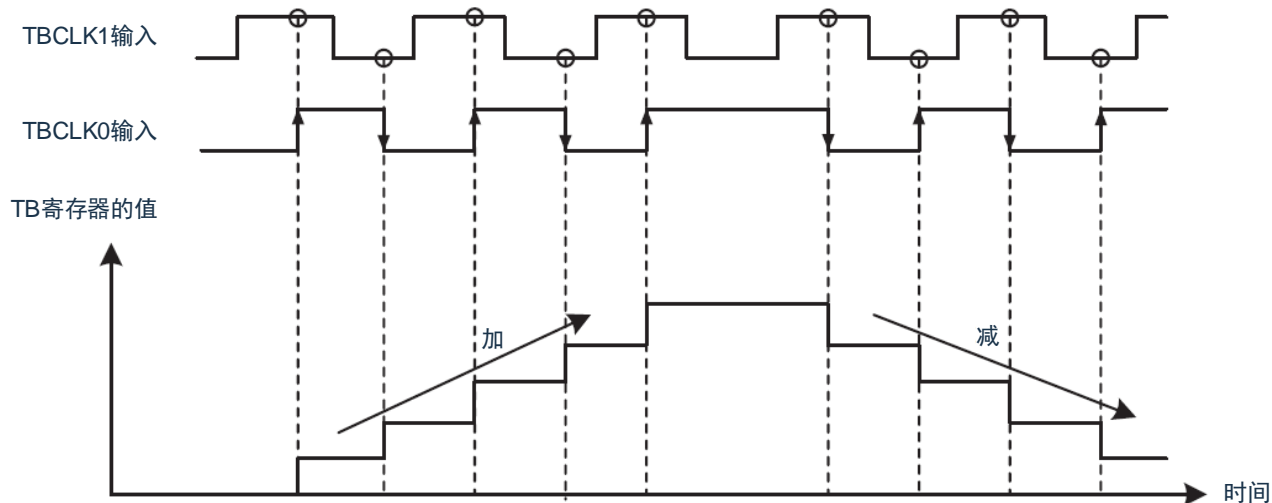
图8-30 相位计数模式的运行例子4
