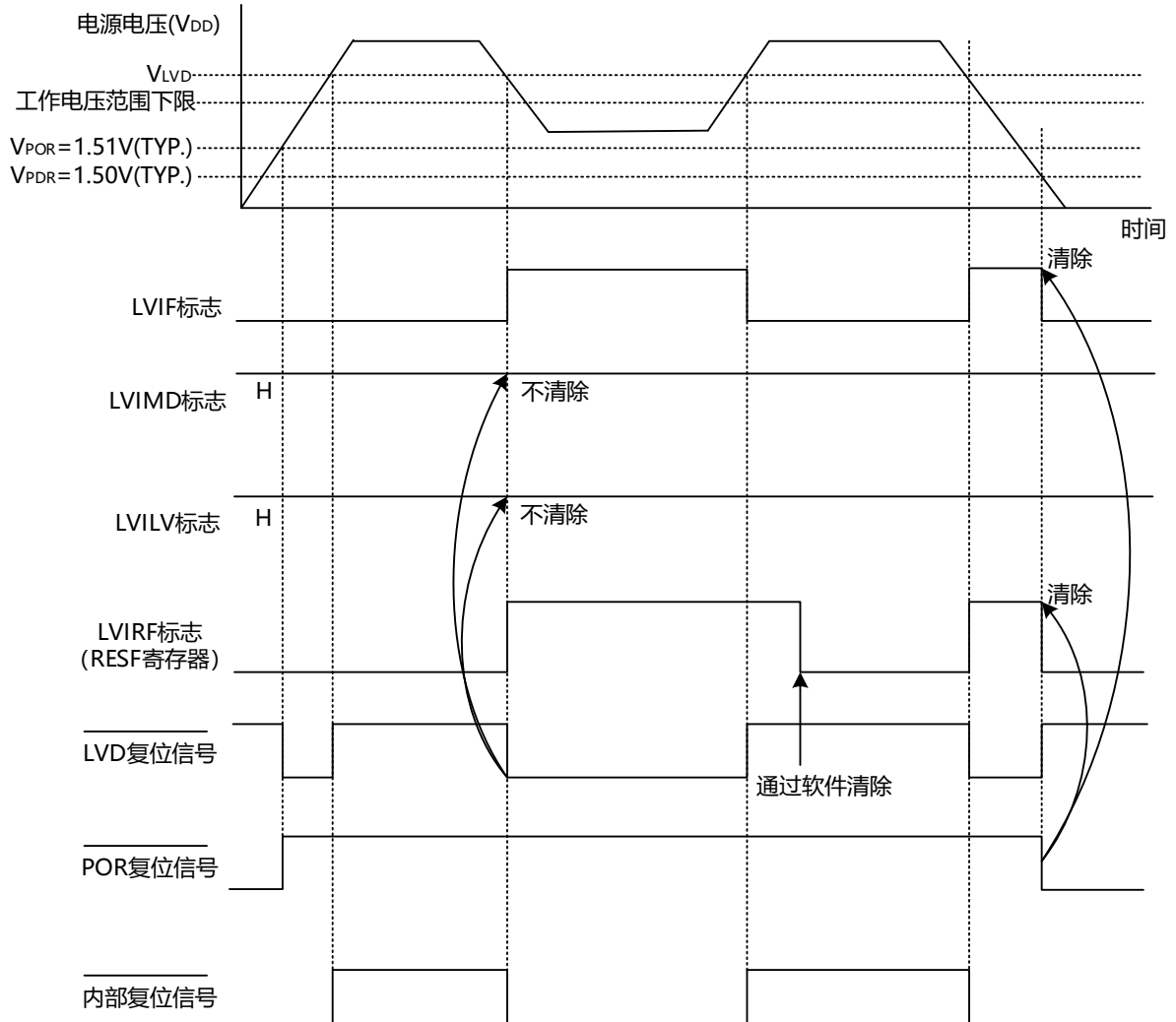
图30-4 内部复位信号的产生时序(选项字节的LVIMDS1、LVIMDS0=1、1)
