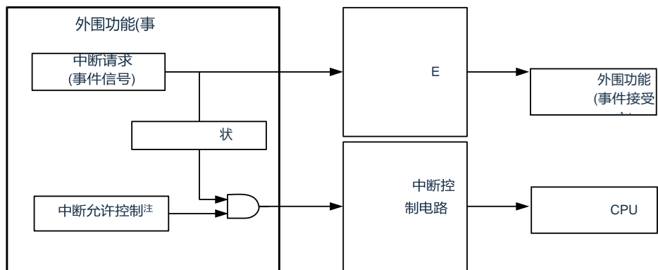
图24-3 中断处理和EVENTC的关系
