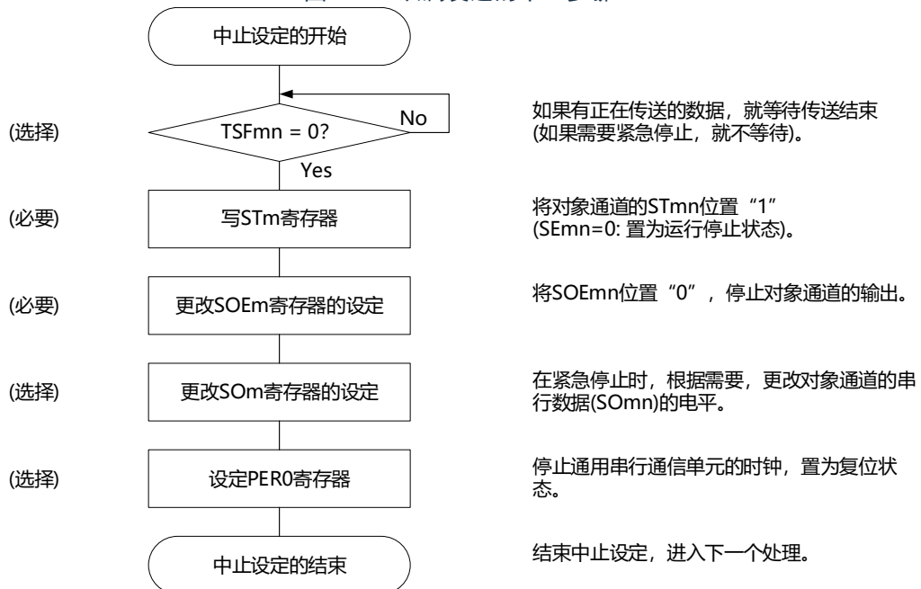
图19-51 从属发送的中止步骤
