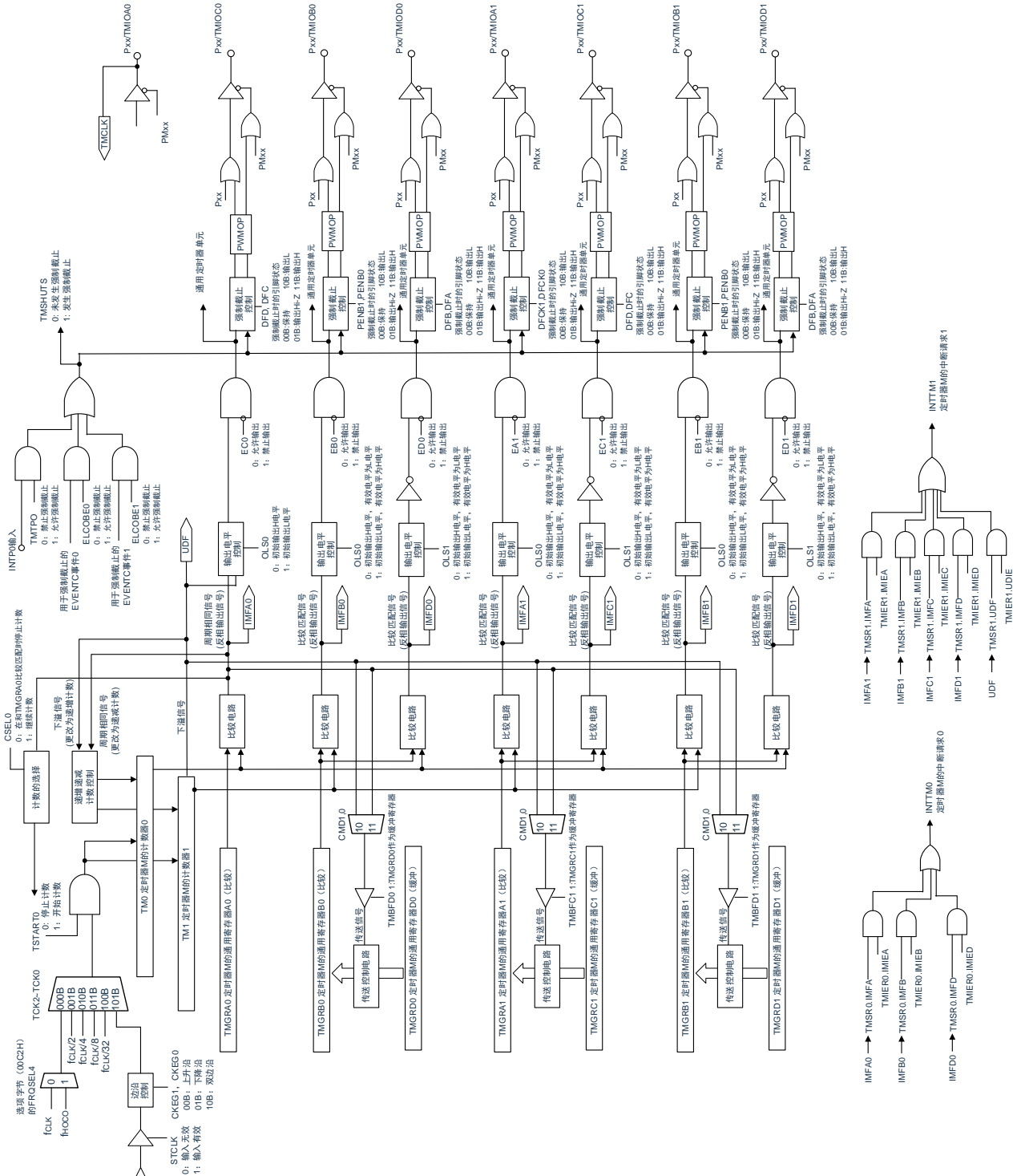
图10-58互补PWM模式的框图
