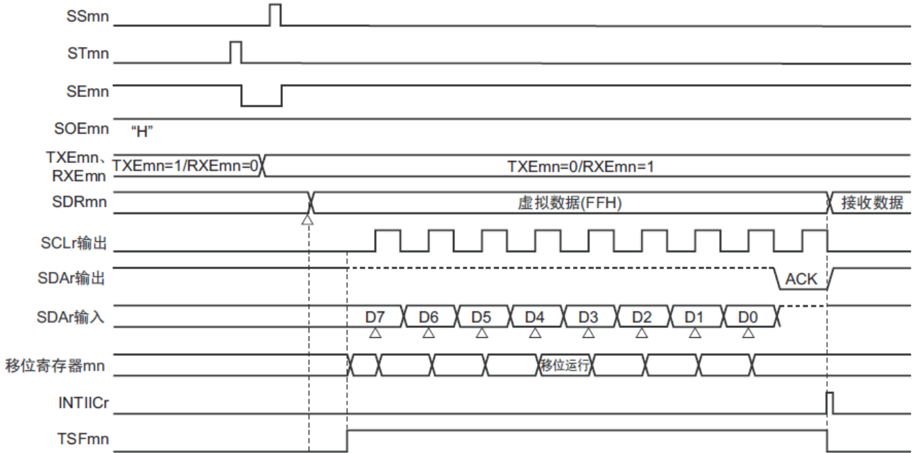
图19-136 数据接收的时序图
