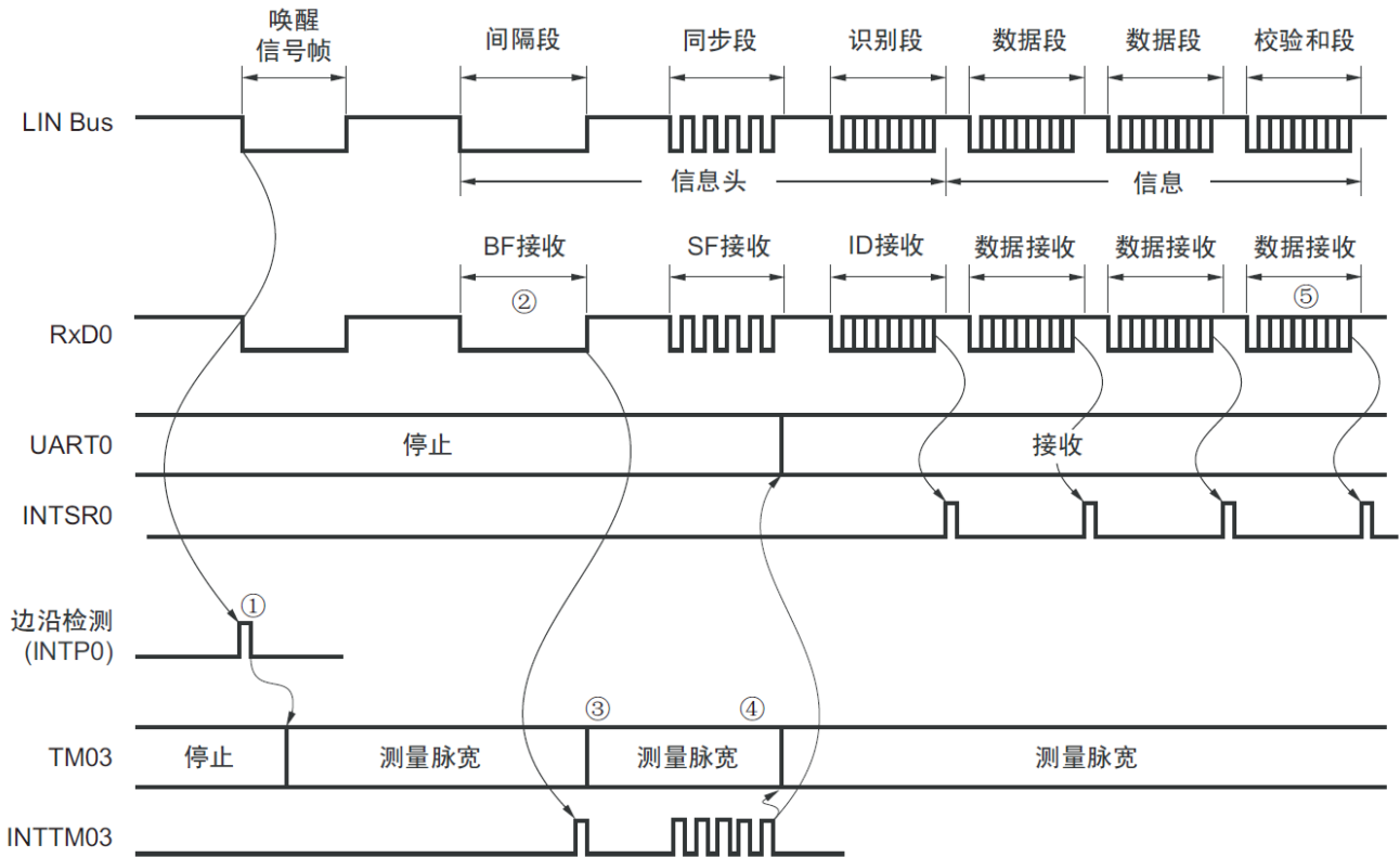
图19-125 LIN的接收操作
