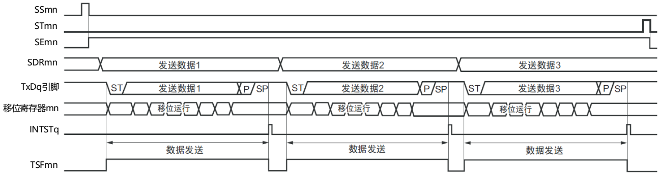
图19-105 UART发送(单次发送模式)的时序图
