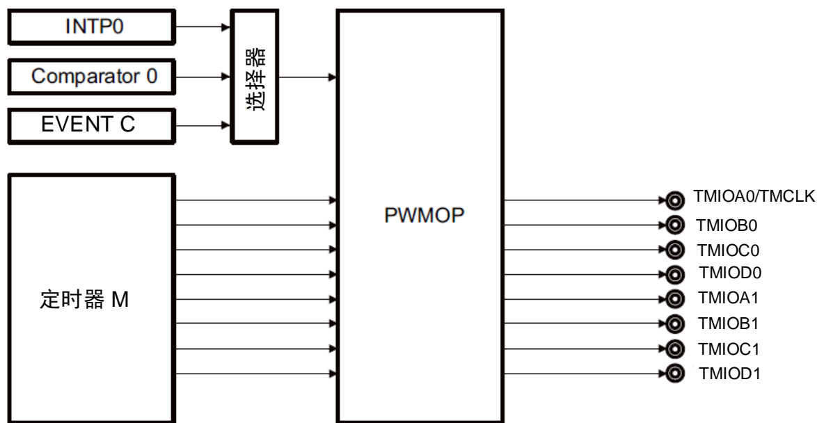
图10-68 PWMOP的框图
