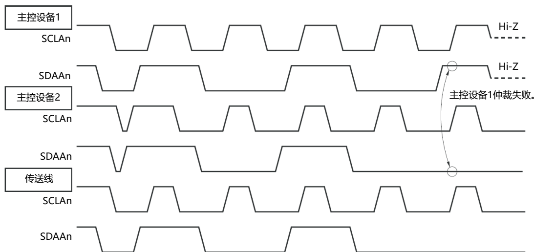
图20-21 仲裁时序例子
