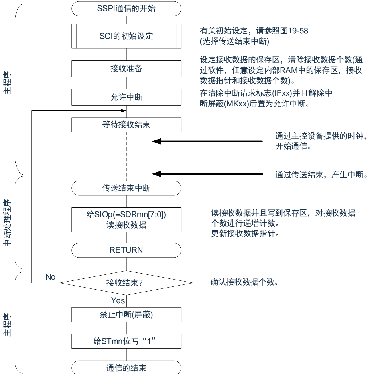
图19-62 从属接收(单次接收模式)的流程图
