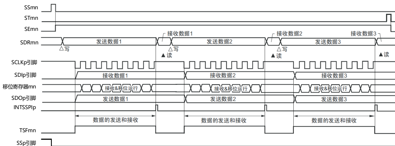
图19-96 从属发送和接收(单次发送和接收模式)的时序图(类型1: DAPmn=0、CKPmn=0)
