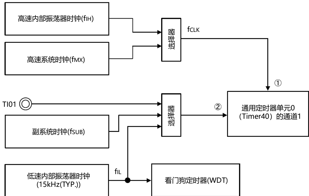
图31-10 频率检测功能的结构
