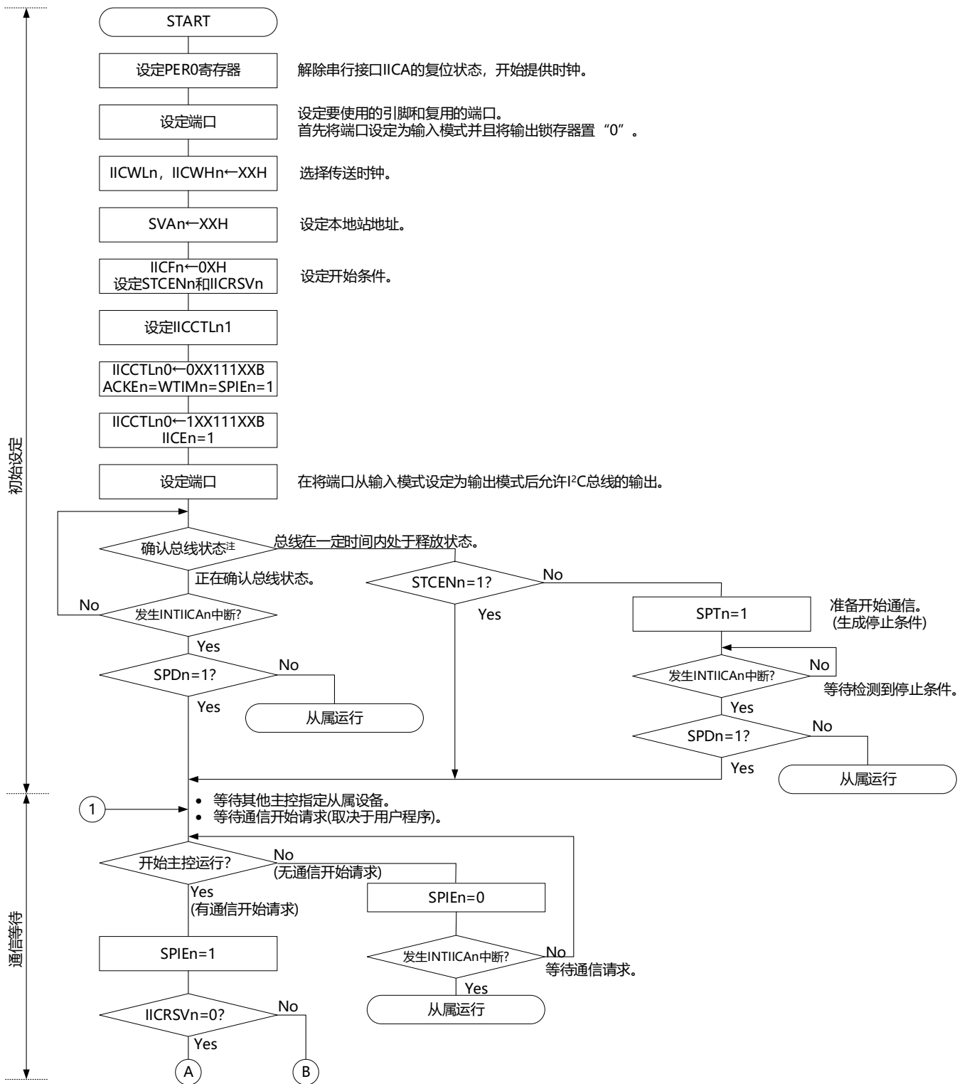
图20-29 多主控系统的主控运行(1/3)
