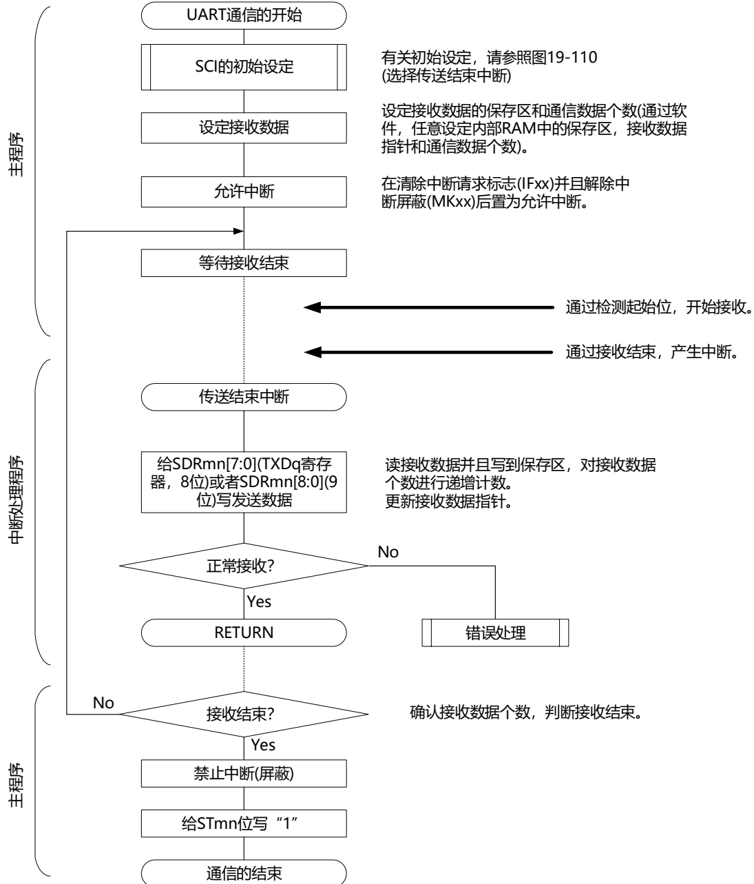
图19-114 UART接收的流程图
