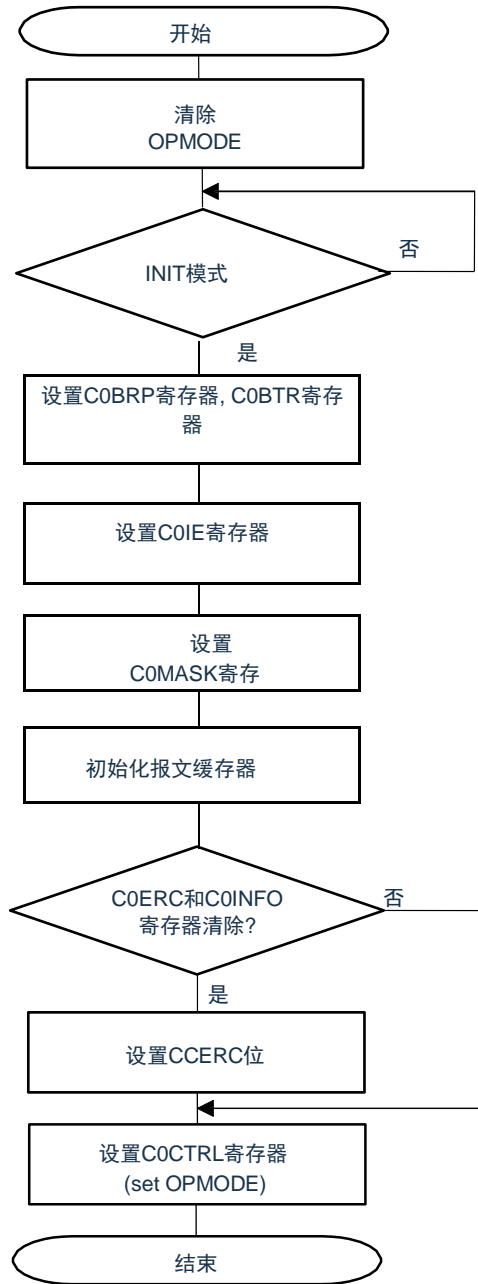
图21-64.重新初始化
