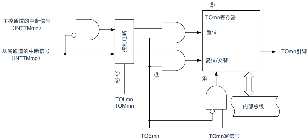
图6-31 输出电路的结构
