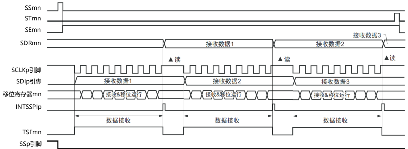
图19-90 从属接收(单次接收模式)的时序图(类型1: DAPmn=0、CKPmn=0)
