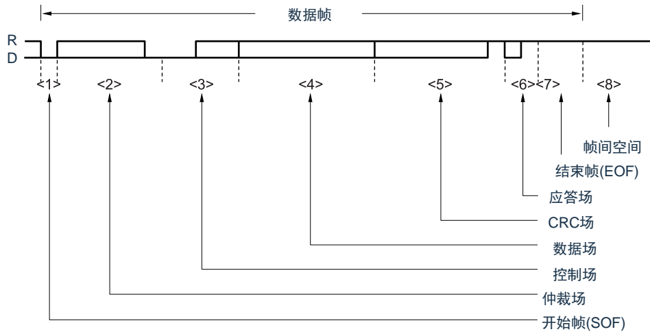
图21-3. 数据帧
