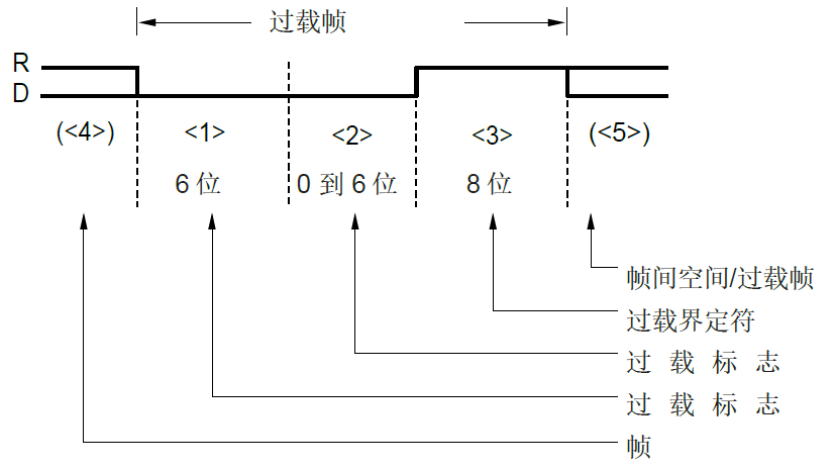
图21-16. 过载帧
