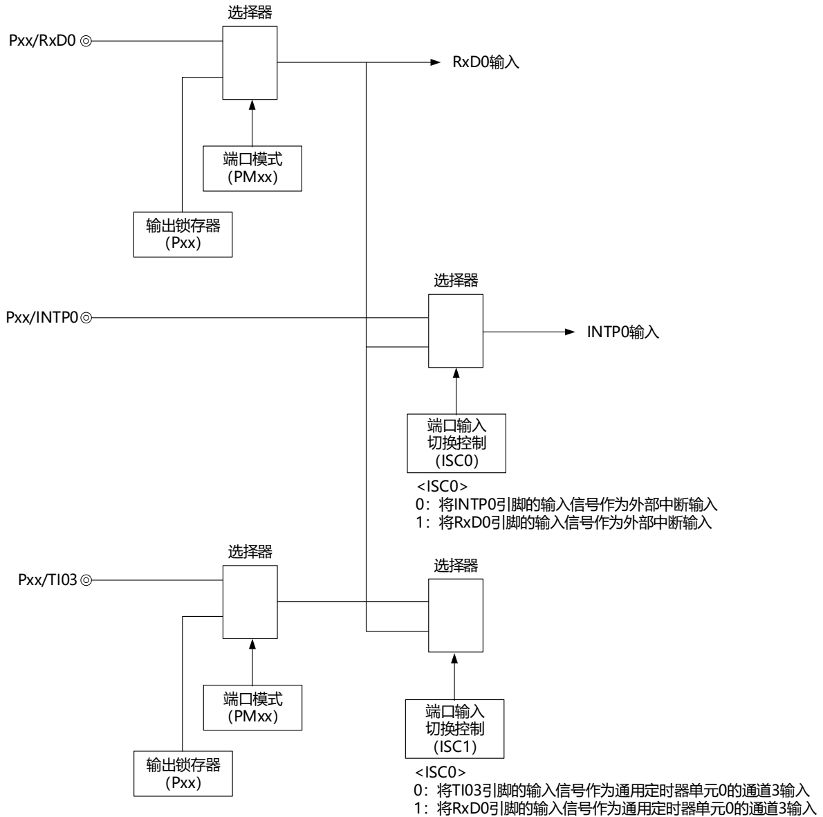
图19-127 用于LIN接收操作的端口结构图
