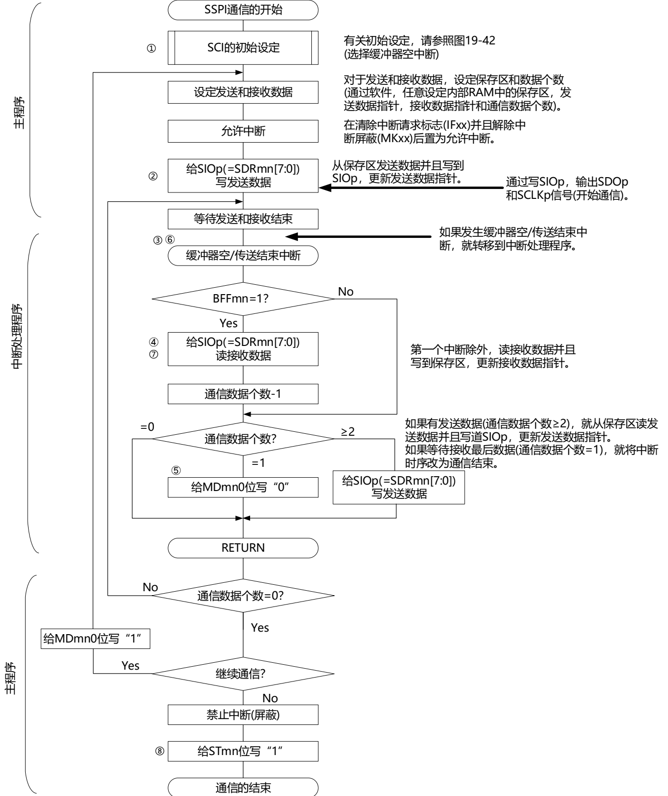
图19-48 主控发送和接收(连续发送和接收模式)的流程图
