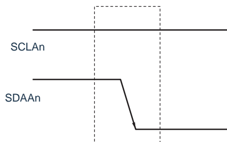
图20-15 开始条件
