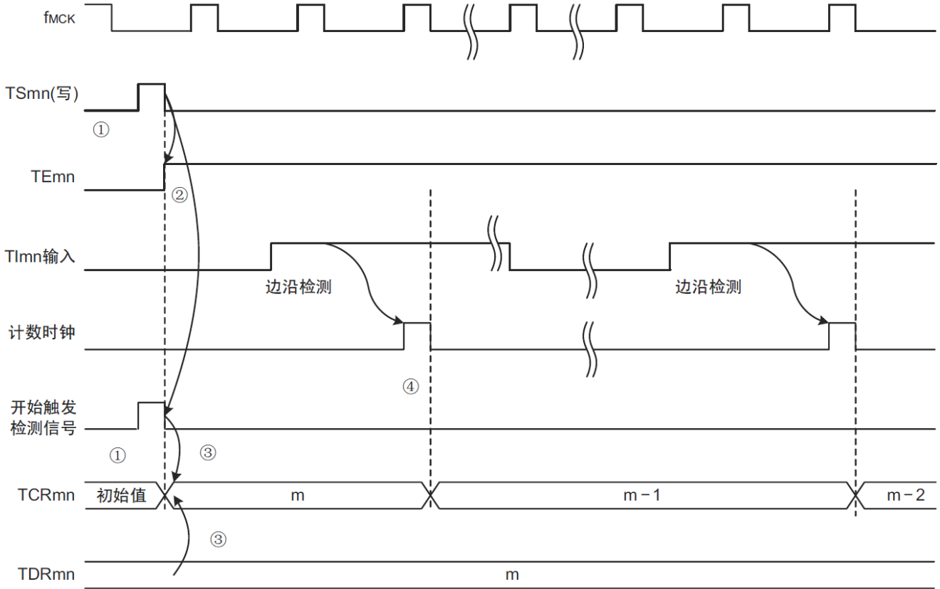
图6-27 运行时序(事件计数器模式)
