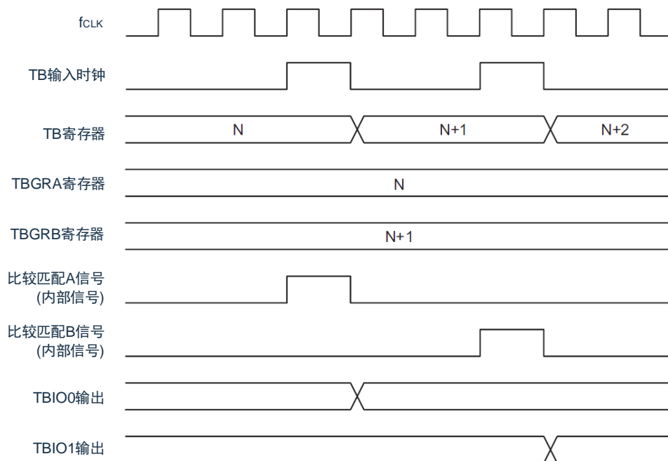
图8-20 输出比较的输出时序
