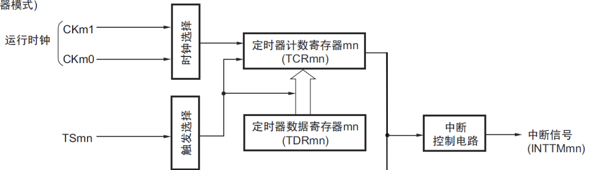
图6-72 作为多重PWM输出功能运行的框图(输出2种PWM的情况)
