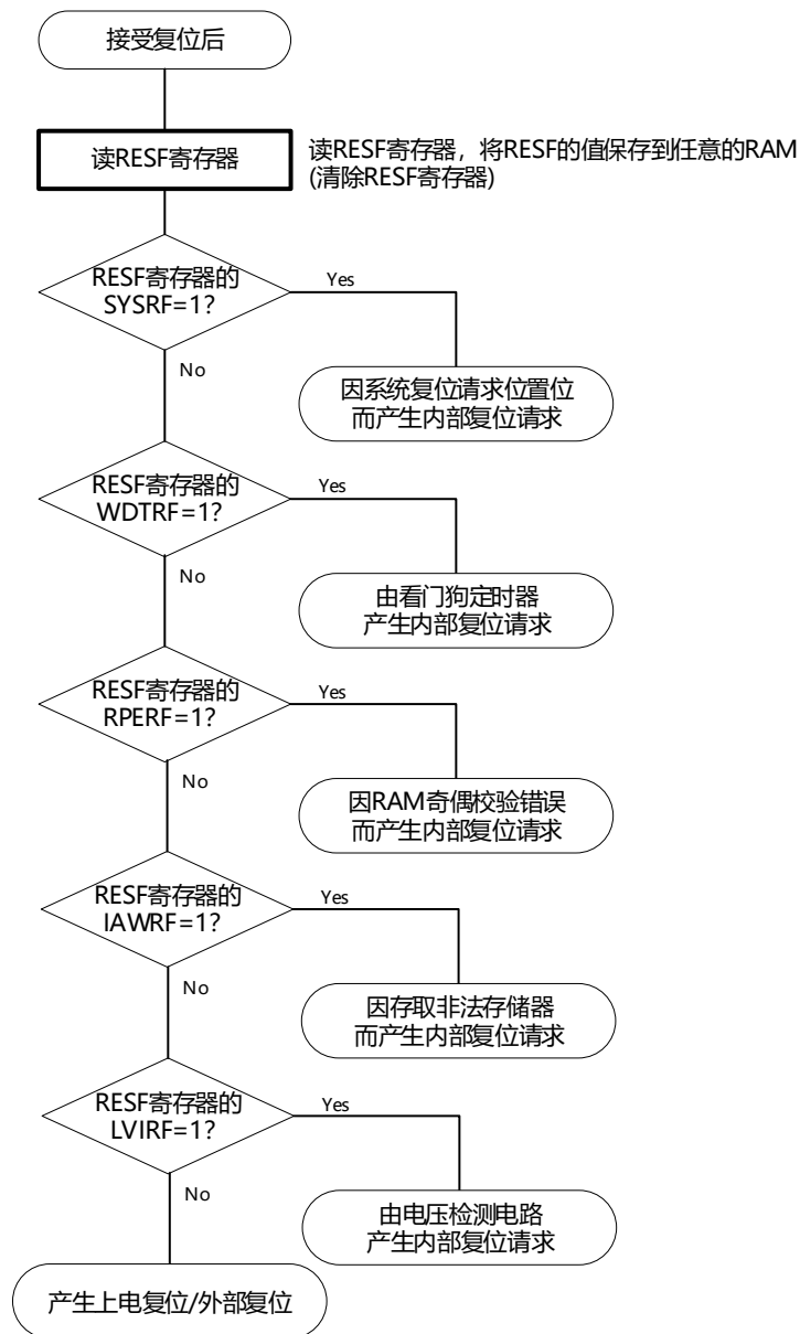
图28-5 复位源的确认步骤
