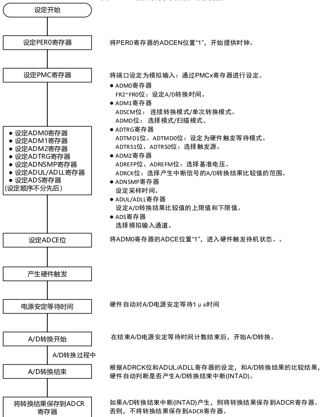
图15-32 硬件触发等待模式的设置
