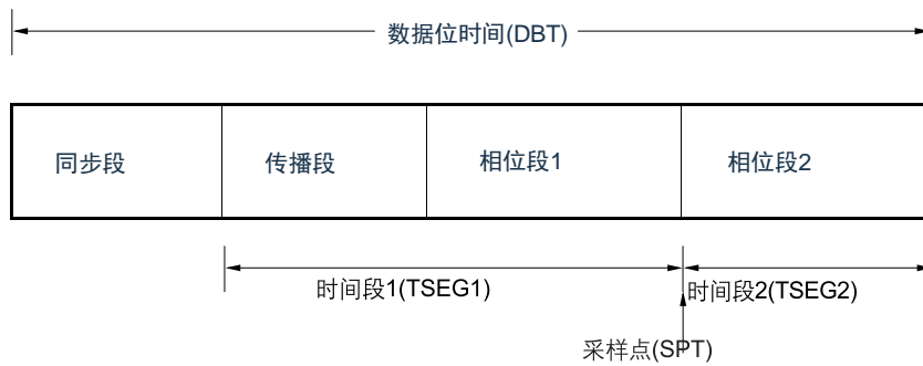
图21-40. 数据位时间
