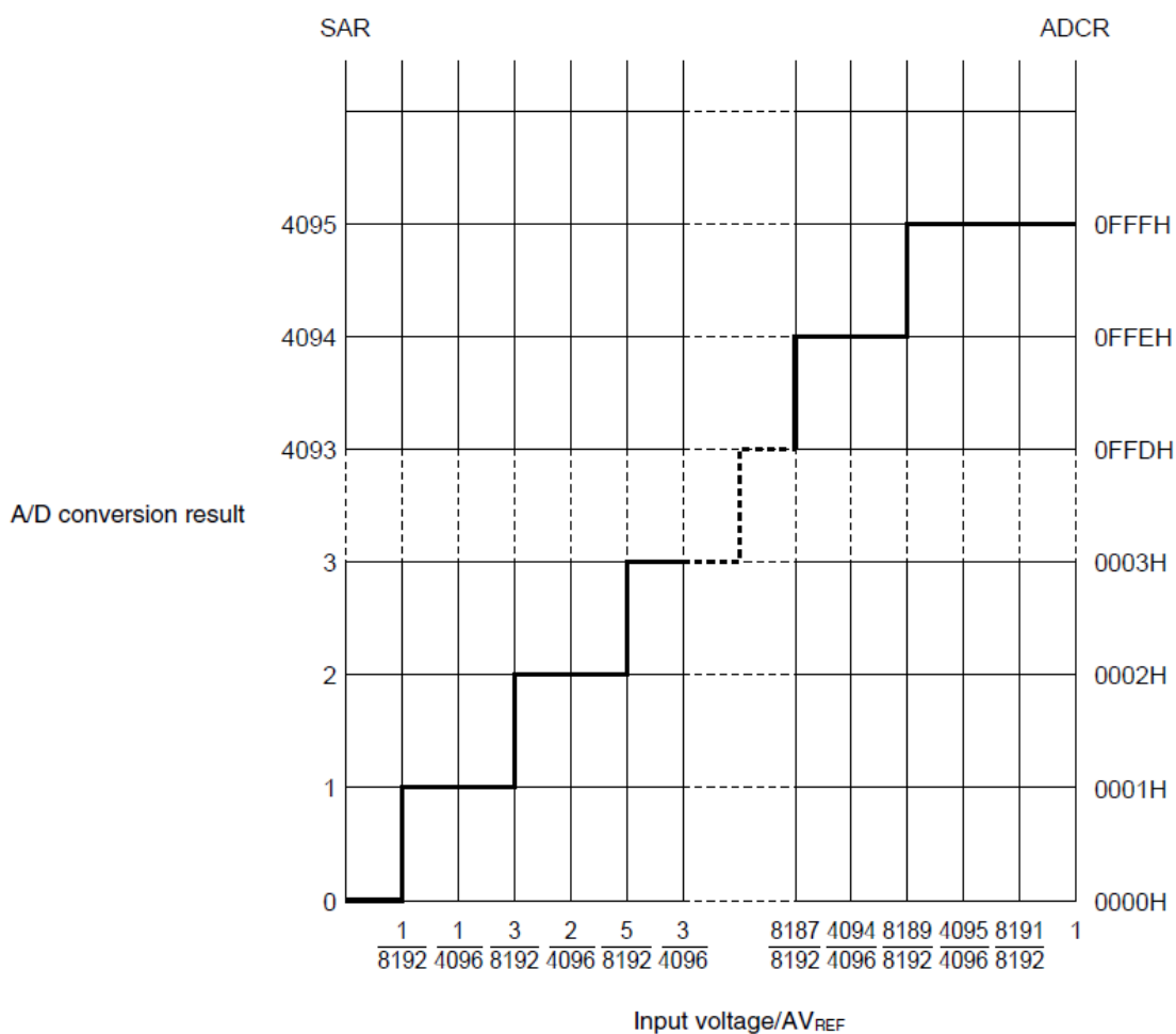
图15-16 模拟输入电压和A/D转换结果的关系
