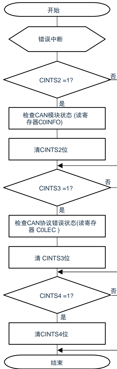
图21-86. 错误处理
